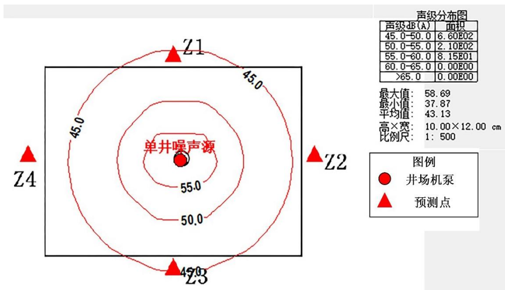
图 6.2-1 等声级线示意图
