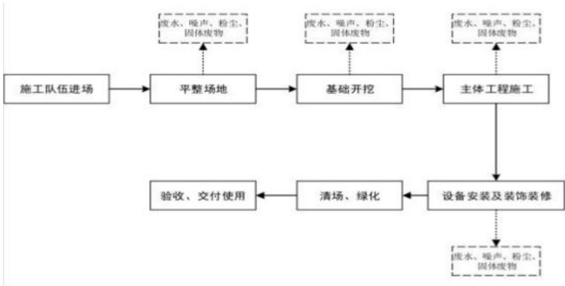
图 3.6.1-1 施工期流程及排污节点示意图
