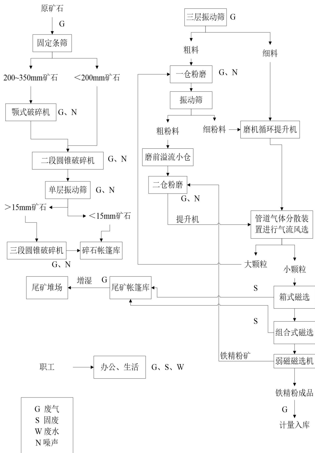
图 3.1.7-1 现有工程工艺流程及产污环节
