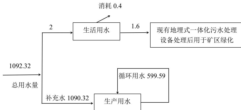
图 3.6.3-1 本项目水平衡图 (m³/d)
