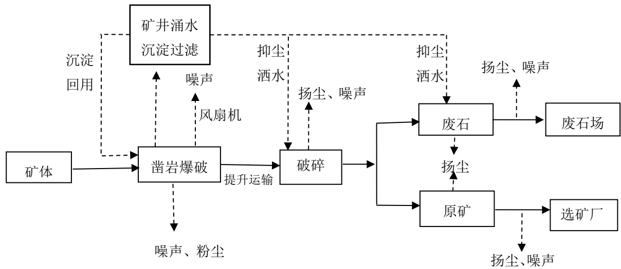
图 3.4-2 地下采矿工艺流程及排污节点示意图
