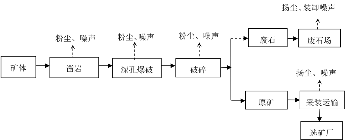
图 3.4-1 露天开采工艺排污节点示意图
