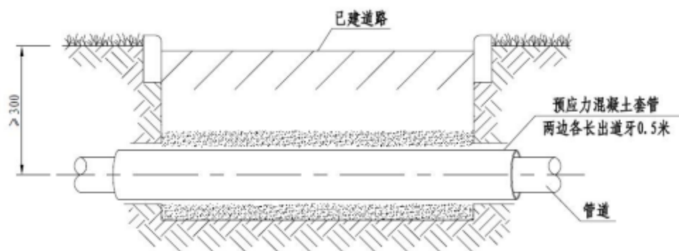
图 2.2-7 顶管施工断面示意图
