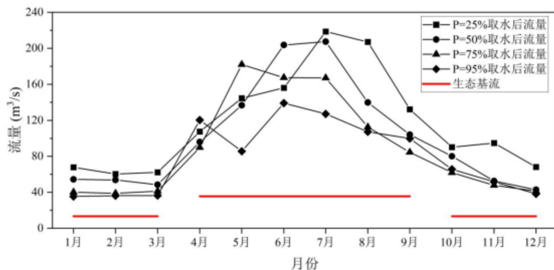
图 5.2-1 不同来水频率下取水后逐月流量变化过程
