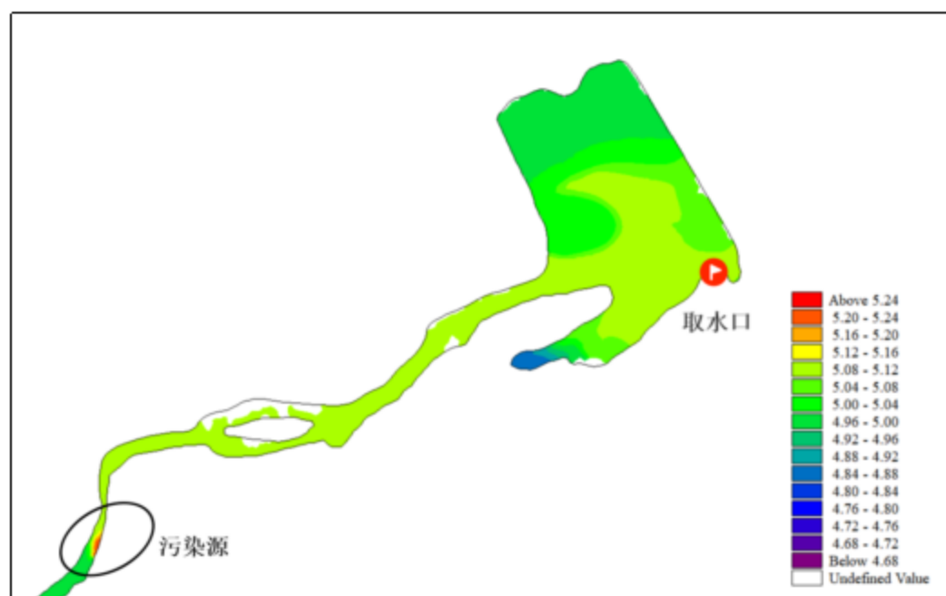
图 5.2-2 生活污水直排情境下 COD 浓度分布图
