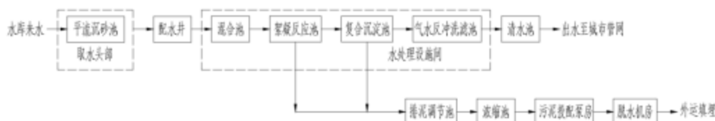
图 2.2-1 净水厂工艺流程示意图
