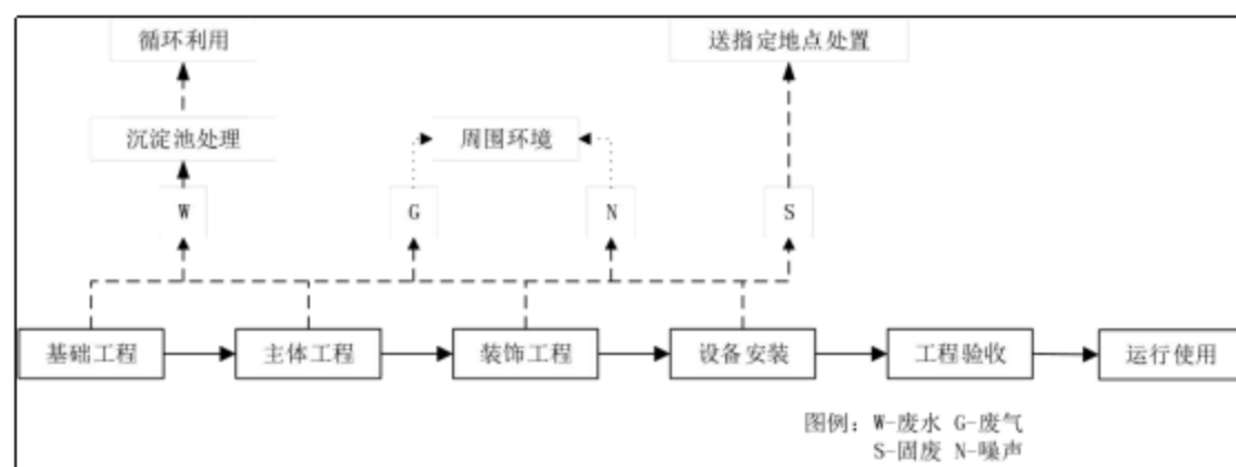
图 2.2-9 施工期建筑施工工艺及产污节点图
