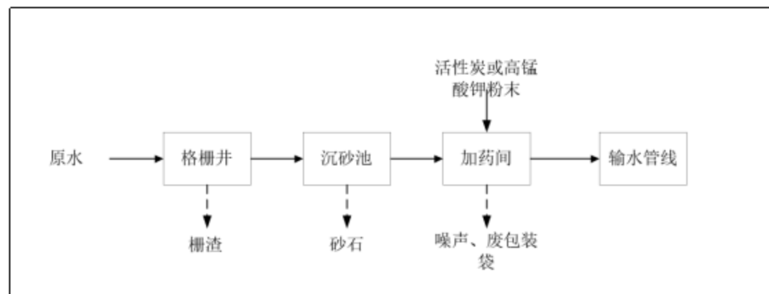
图 2.2-12 预处理站工艺及产污节点图
