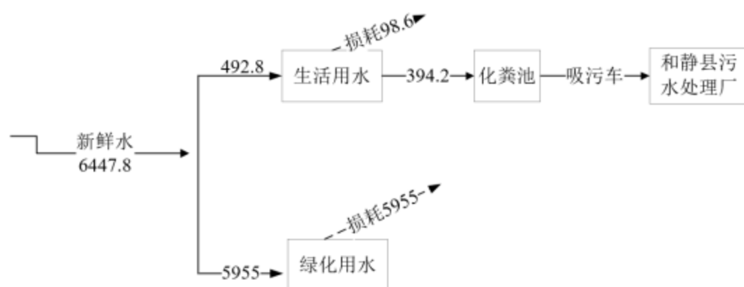
图 2.2-8 水平衡图
