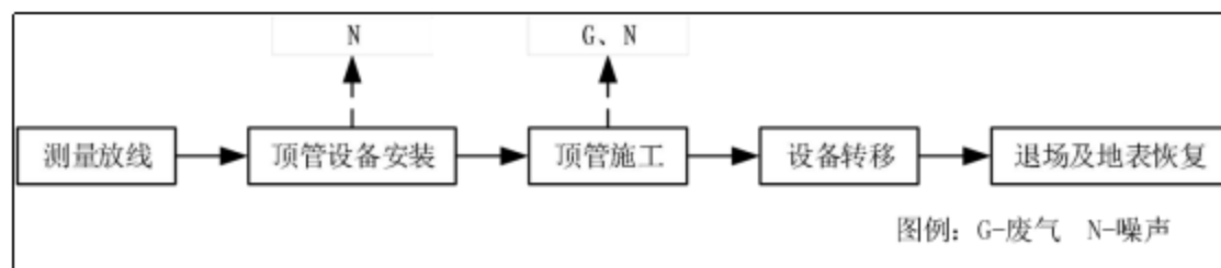
图 2.2-11 施工期管道施工（顶管法）工艺及产污节点图
