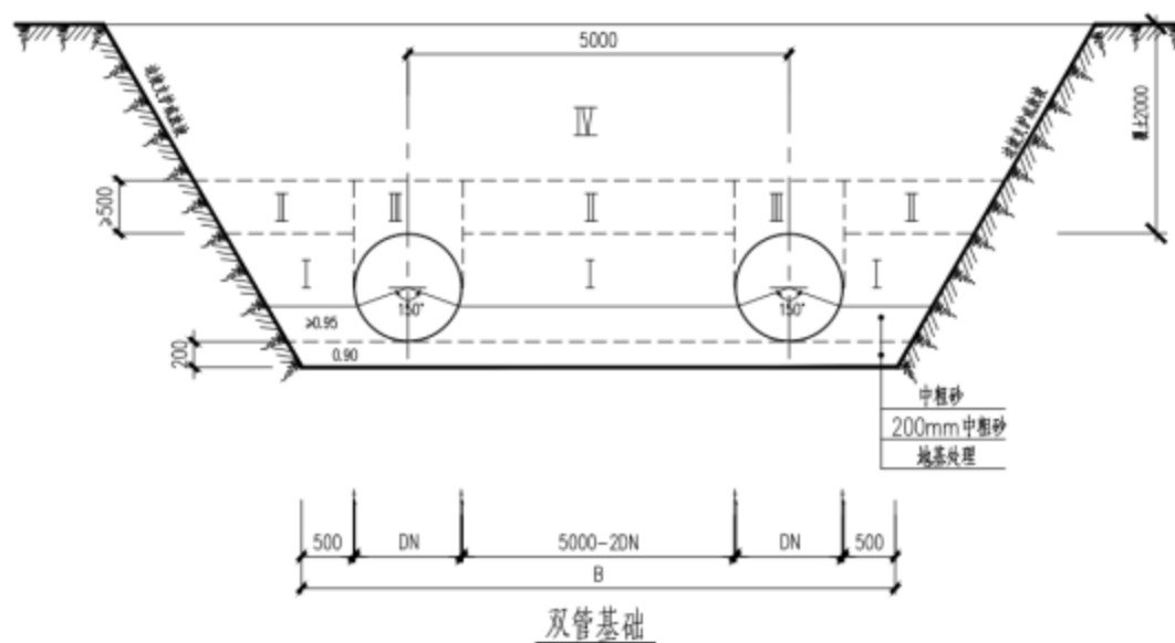
图 2.2-5 输水管线结构断面图
