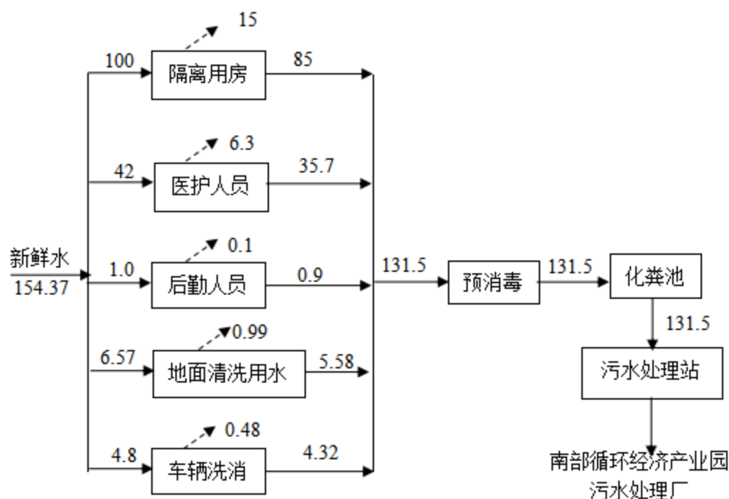
图 3.1-4 项目水平衡图 单位：m 3 /d
