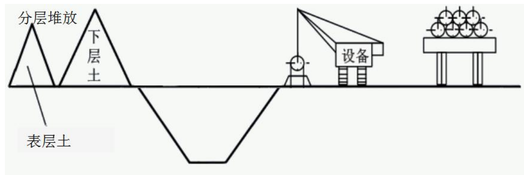
图 3.3-2 一般地段管道施工方式断面示意图
