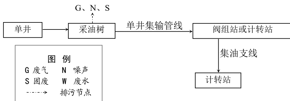
图 3.3-4 井场工艺流程图
