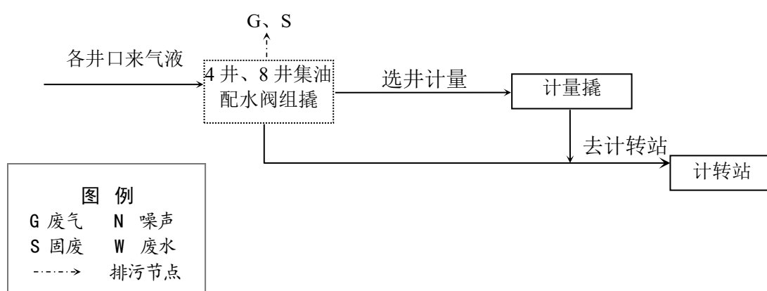
图 3.3-5 阀组站工艺流程图
