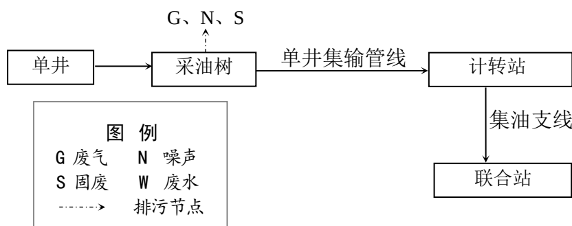
图 3.3-7 井场工艺流程图
