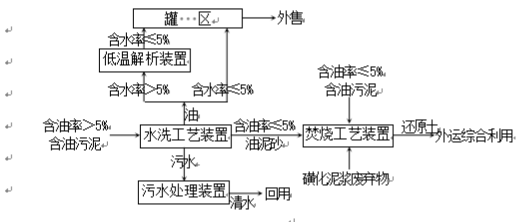
图 3.2-16 固废处理工艺流程图
