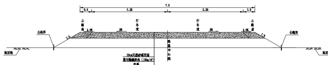
图 3.2-8 基标准横断面图
