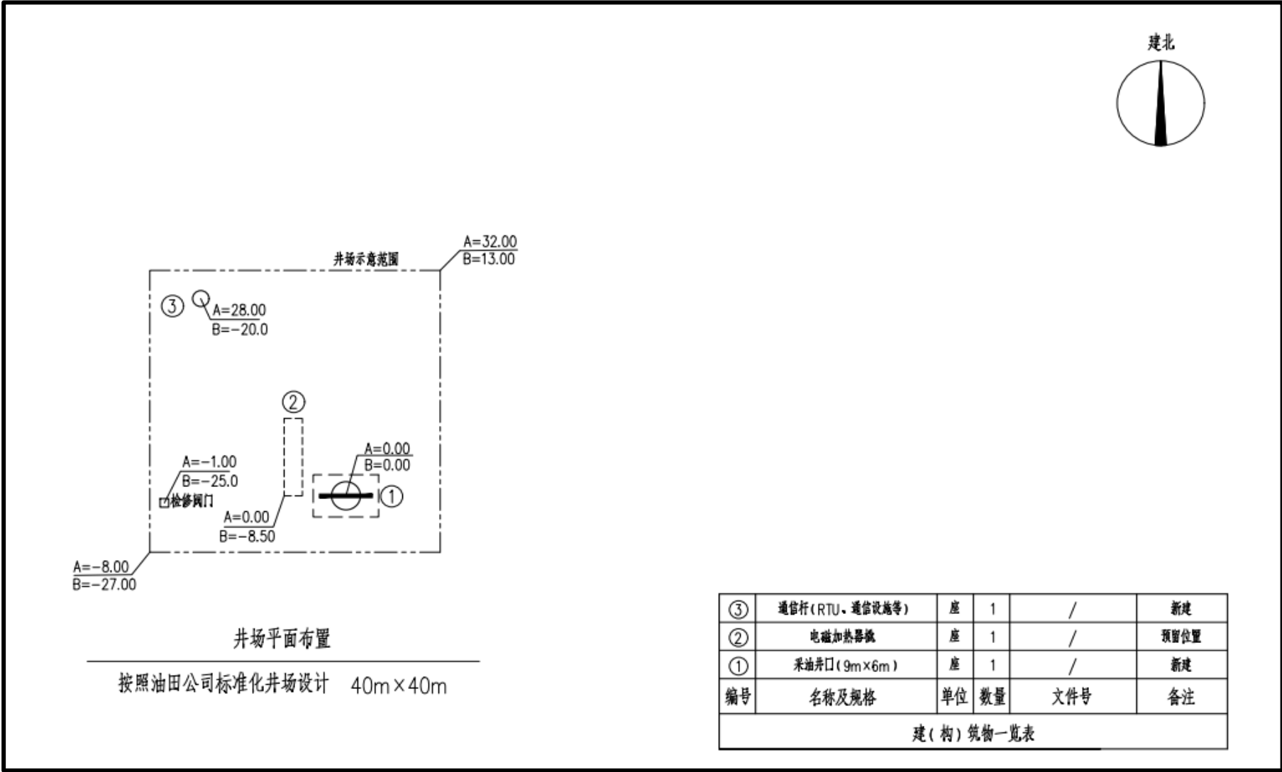
图 3.2-5 采油井场平面布置示意图
