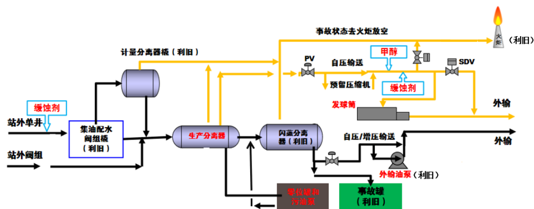
图 3.2-6 目前富源东 2 号计转站流程框图
