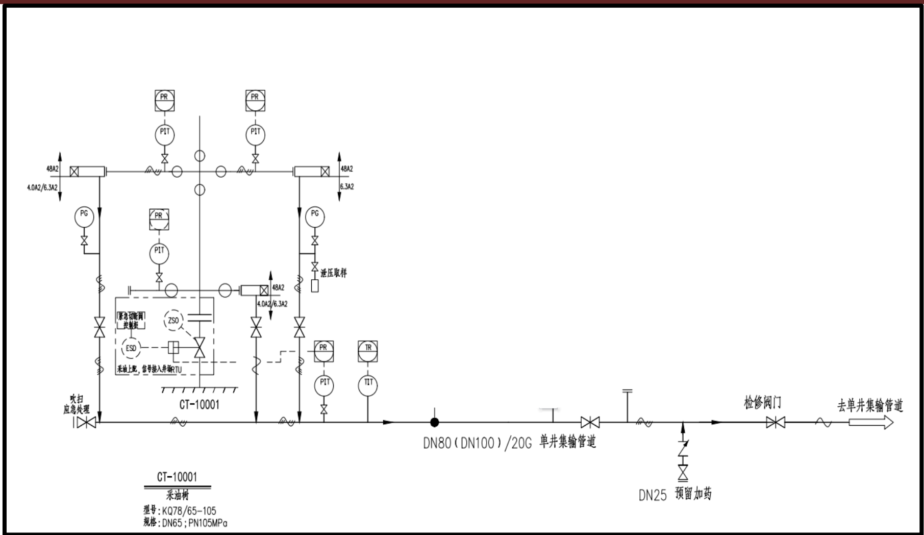
图 3.2-4 采油井场工艺流程图
