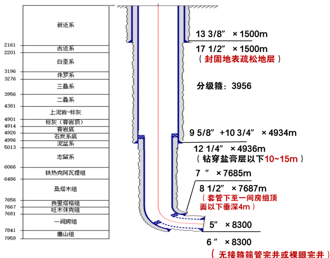
图 3.2-3 井身结构示意图
