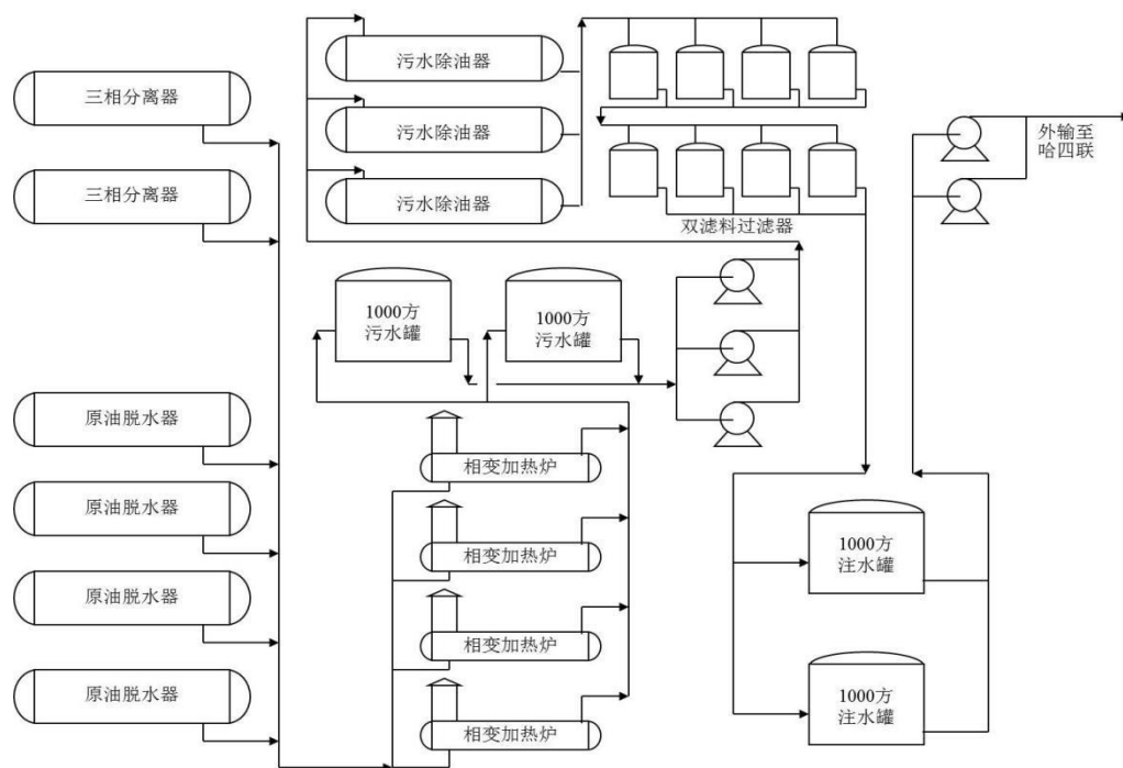
图 3.2-10 哈一联合站含油污水处理工艺流程简图
