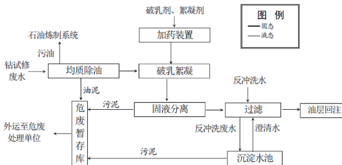
图 3.2-15 塔河南岸区块钻试修废弃物环保处理站废水处理工艺流程图
