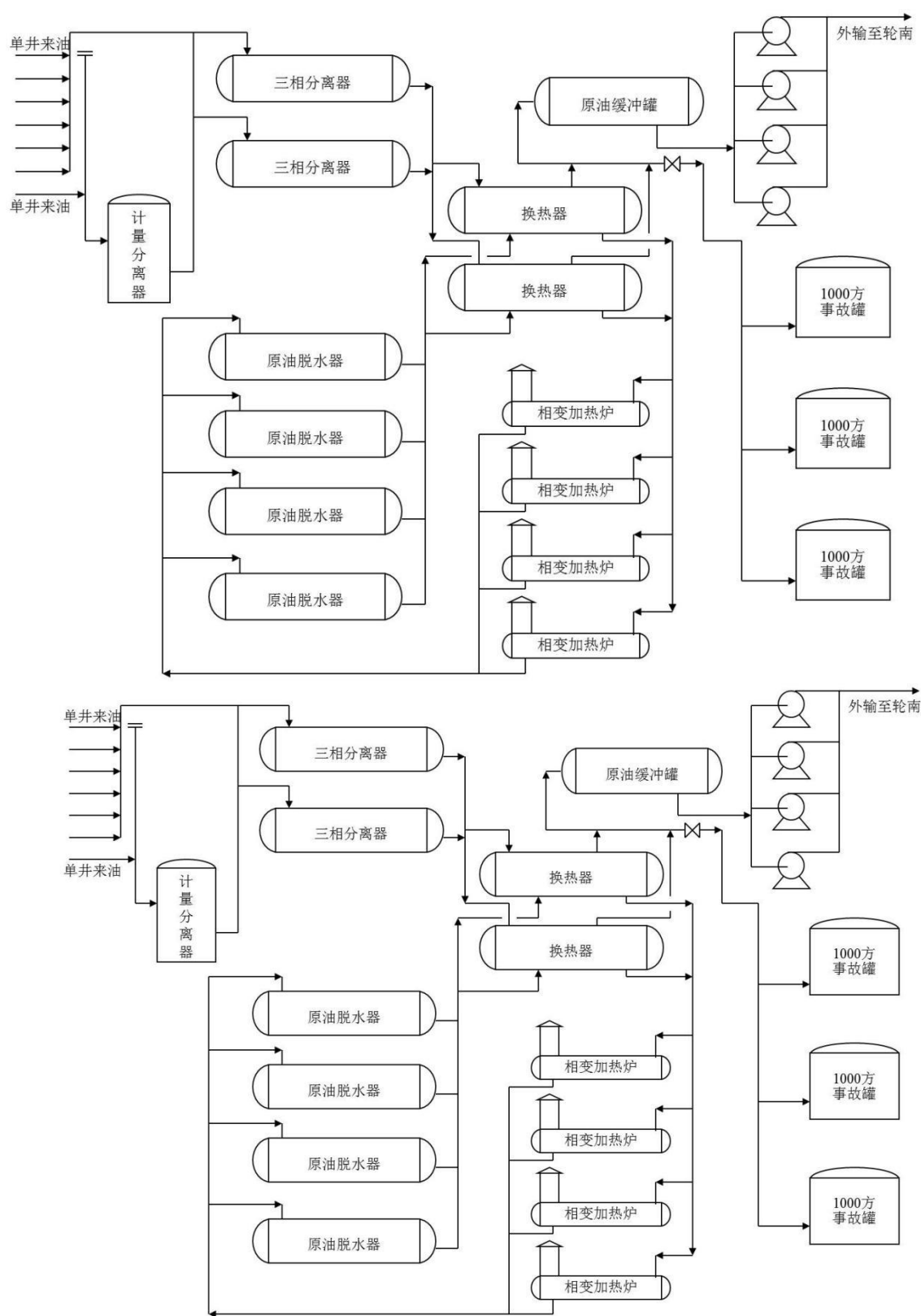
图 3.2-10 哈一联合站原油处理工艺流程简图
