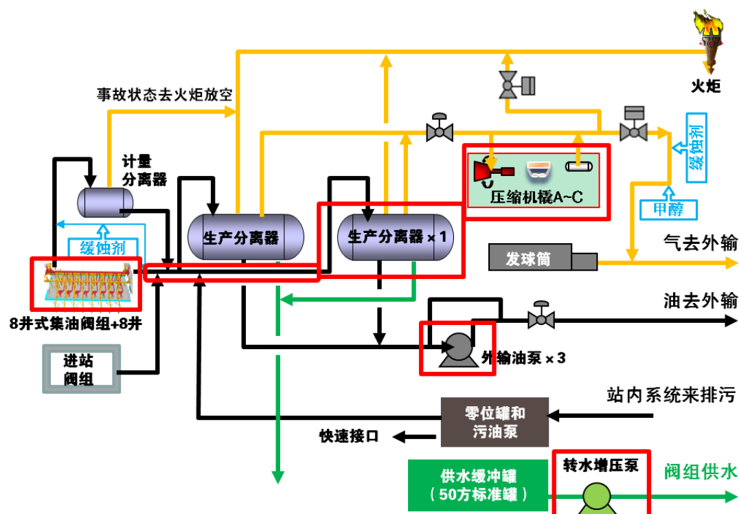
图 3.2-7 改造后富源东 2 号计转站流程框图
