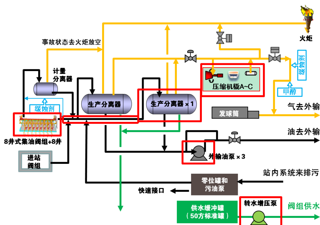
图 3.3-8 改造后富源东 2 号计转站流程框图
