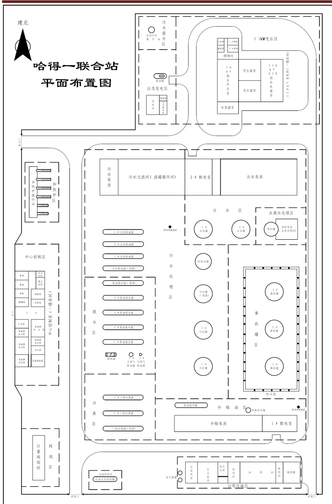
图 3.2-9 哈一联合站平面布置图
