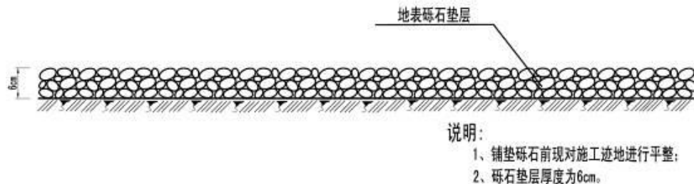
图 6.2-1 井场砾石压盖措施典型设计图
