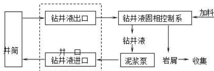
图 3.3-1 钻井液循环示意图
