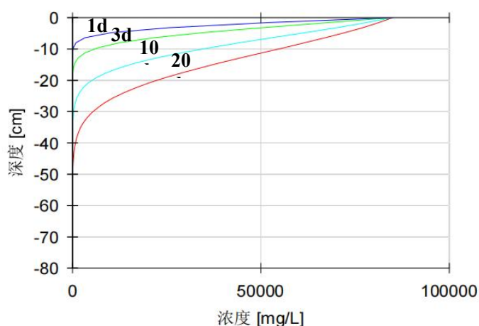
图 5.7-1 石油烃在不同水平年沿土壤垂向迁移情况
