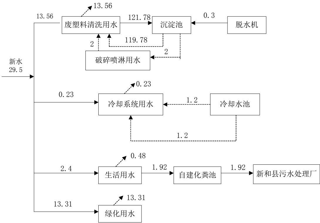
图 3.1-1 全厂用水量平衡图 (单位: m³/d)
