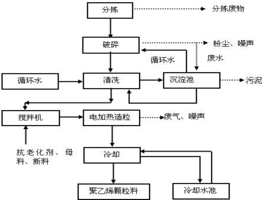
图 3.3-1 造粒工艺流程及产污环节图
