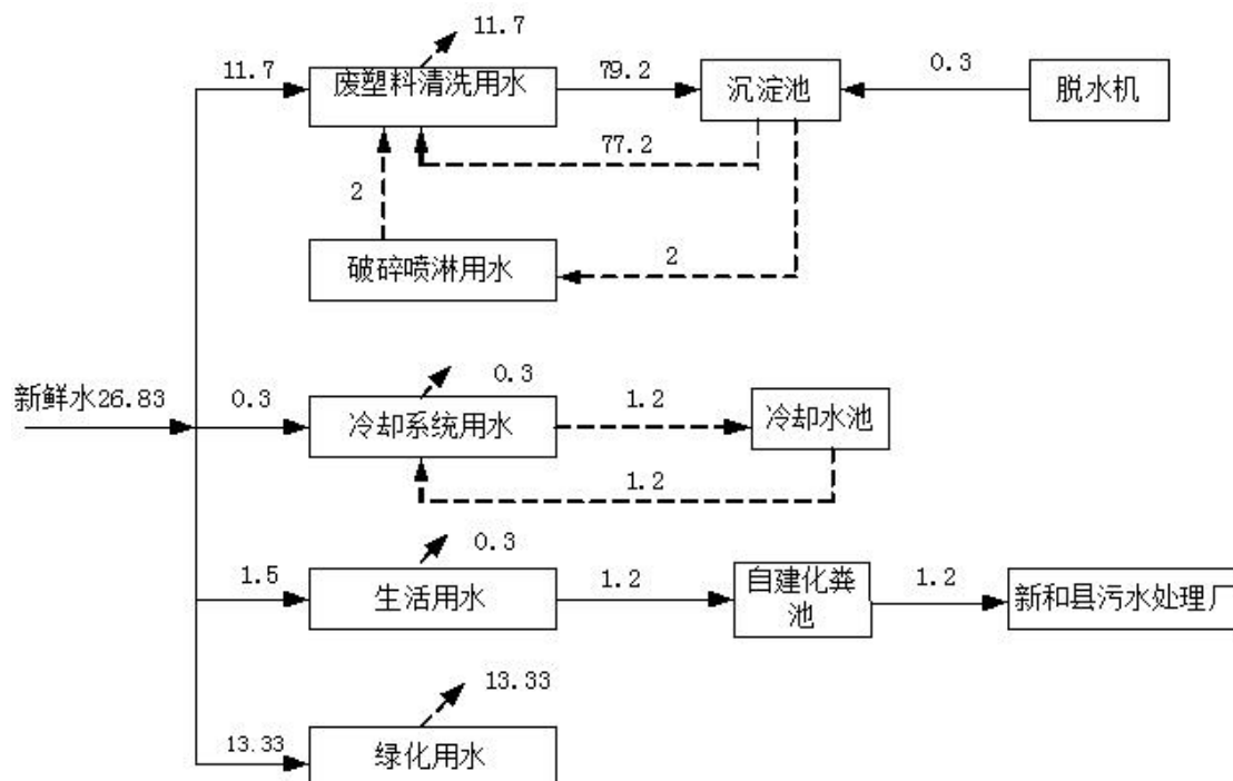
图 3.1-1 全厂总用水量平衡图 (单位: \text{m}^3/\text{d} )
