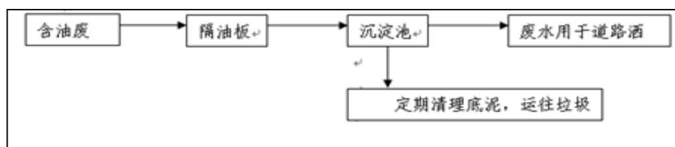
图 7-1 含油废水处理工艺流程图
