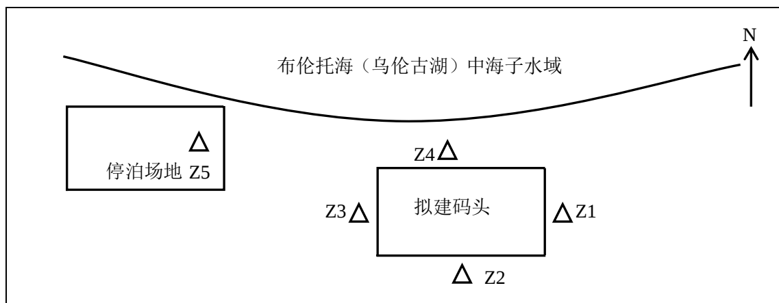
图 5.3-2 环境噪声测点示意图
