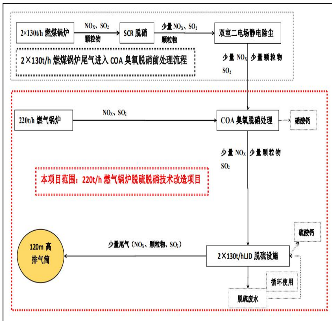
图 7 项目具体工艺流程图和产污节点图
