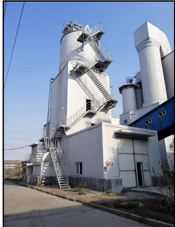
依托 130t/h 的脱硫塔
