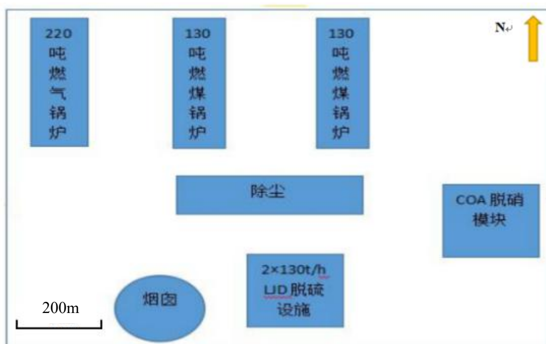
图 5 平面布置图
