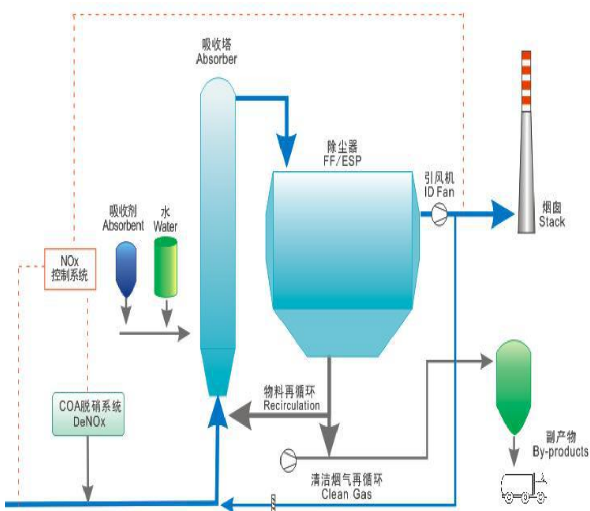
图 6 项目工艺流程及排污节点图
