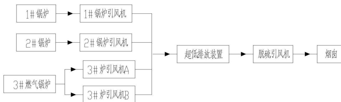
图8 废气处理走向示意图
