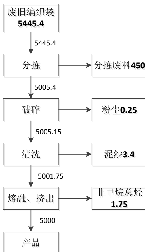
框图 2-4 本项目物料平衡图 单位：t/a
