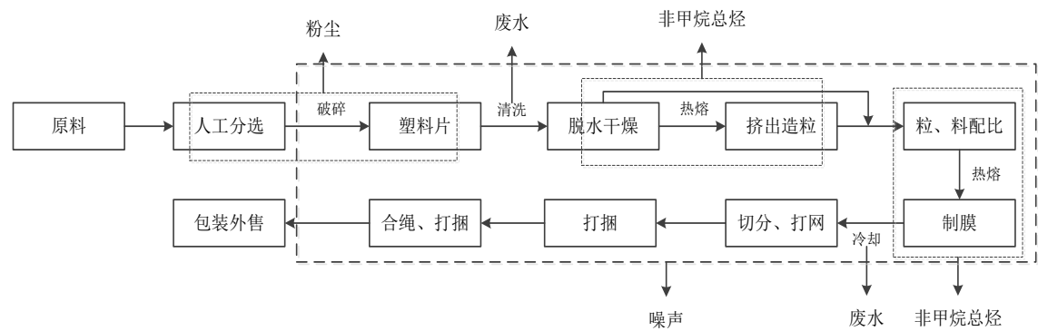
框图 2-2 运营期生产工艺流程及产污环节图
