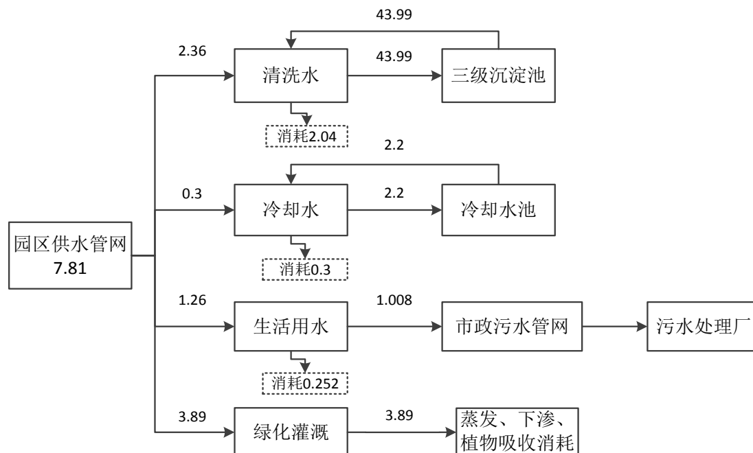
框图 2-3 项目运营期水平衡图 单位 ( \text{m}^3/\text{d} )
