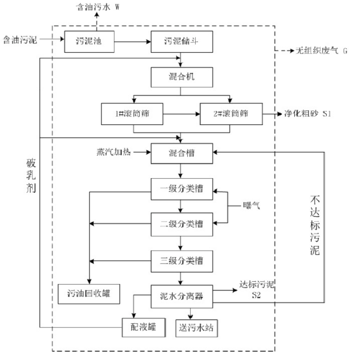
图 3.1-3 水-助溶剂萃取处理工艺流程图
