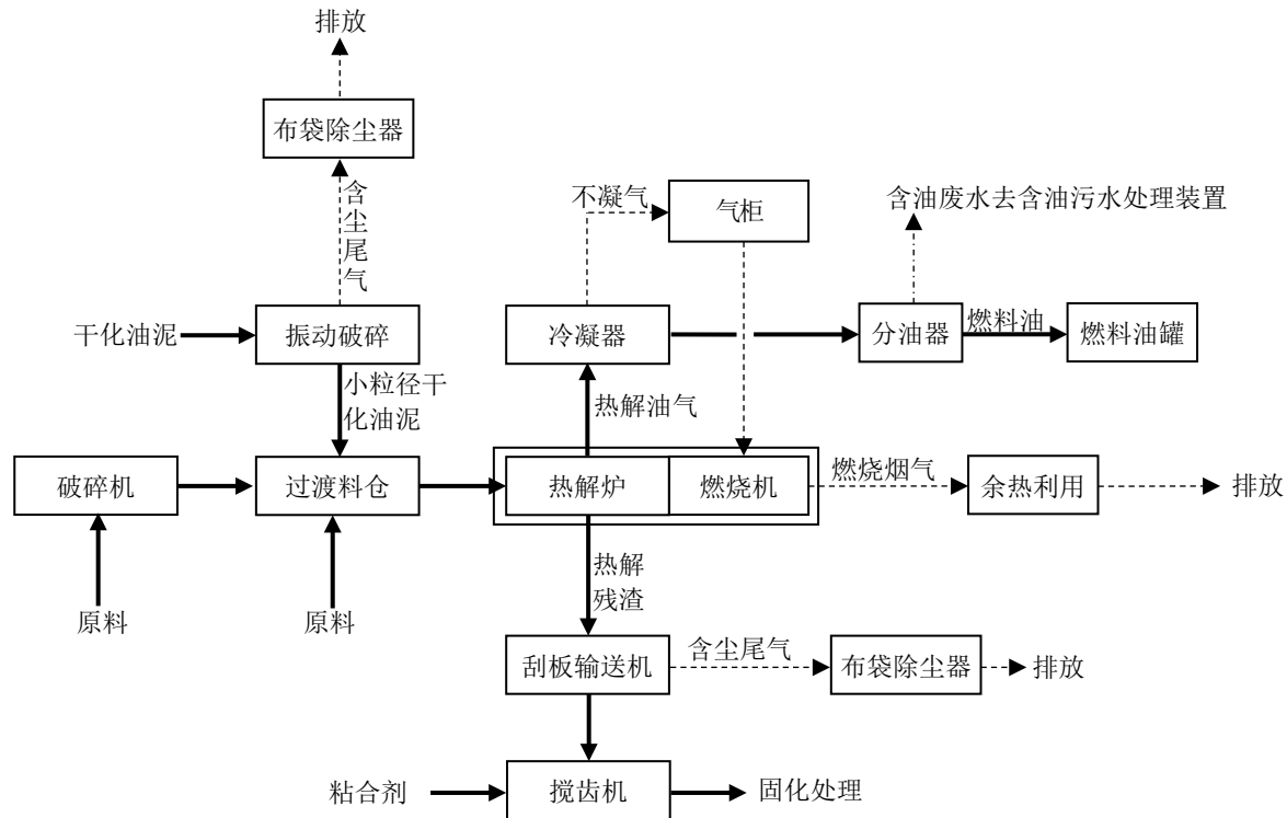
图 3.1-4 热解工艺流程图
