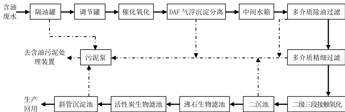
图 3.1-5 含油废水处理工艺流程图
