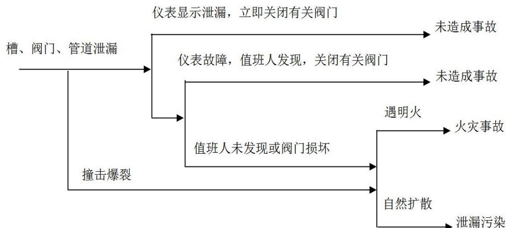
图 6.4-1 项目运行中潜在事故的事件树示意图
