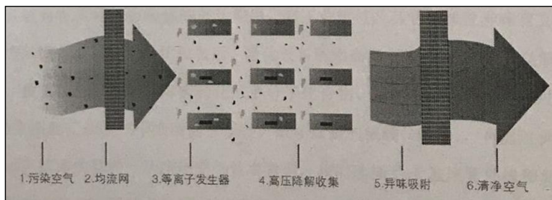
图 7.2-2 等离子光氧设备流程图
