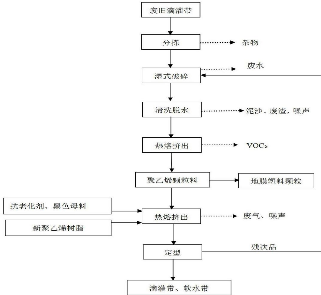
图 3.2-1 本项目造粒生产工艺流程及产污环节图
