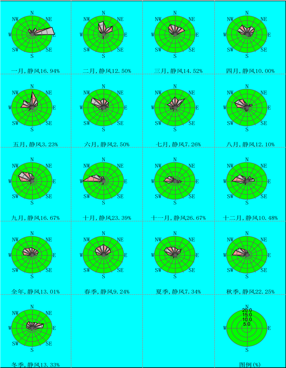
图 5.2-1 项目区风向频率玫瑰图
