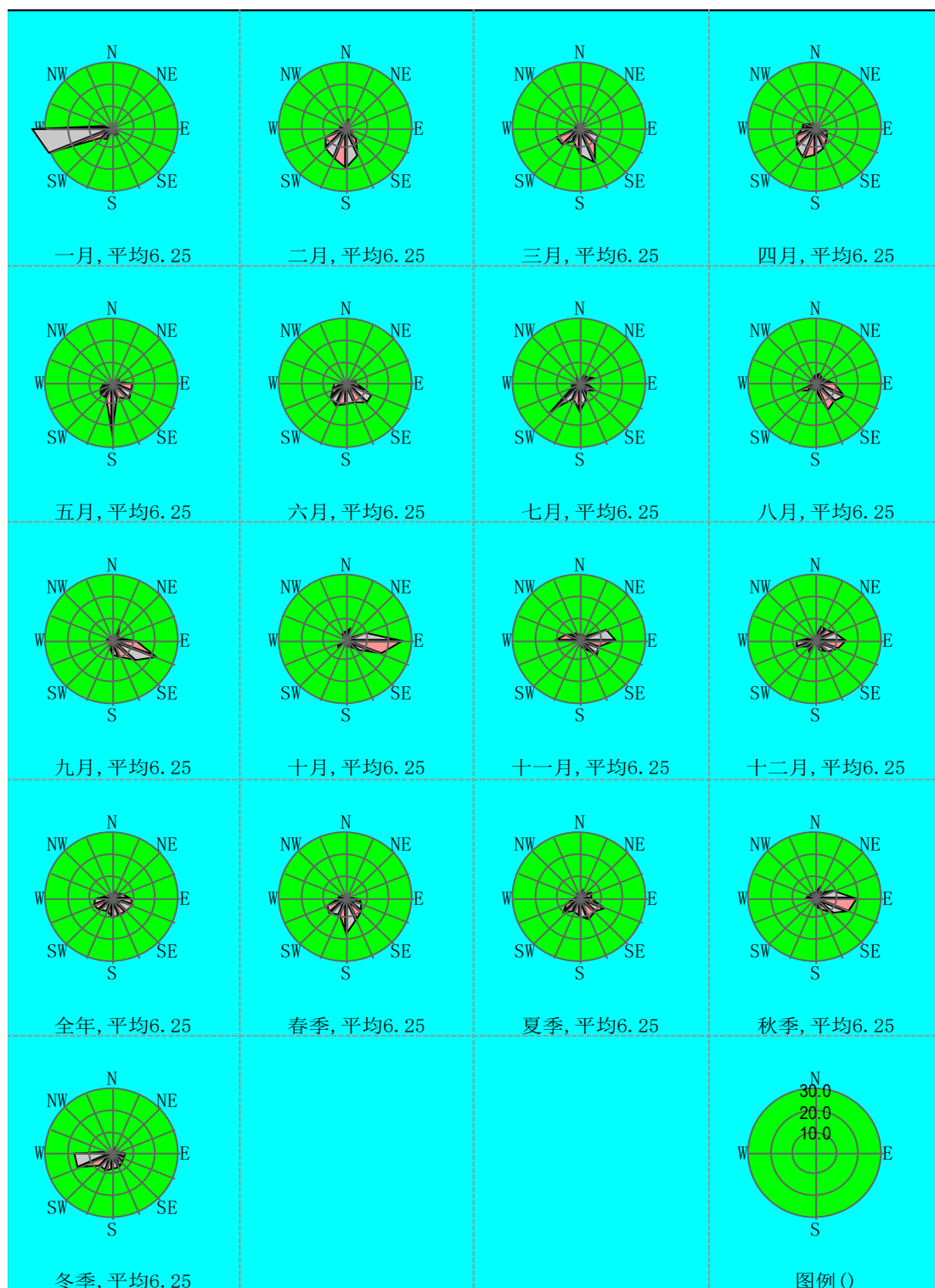
图 5.2-3 污染系数玫瑰图
