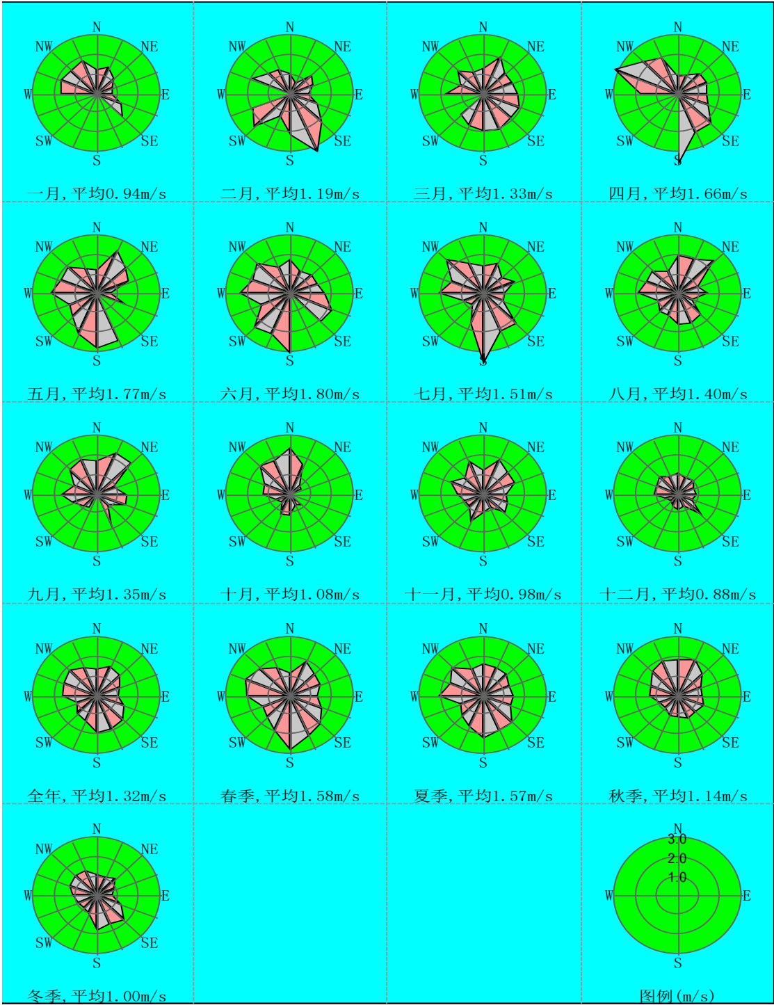
图 5.2-2 风速频率玫瑰图
