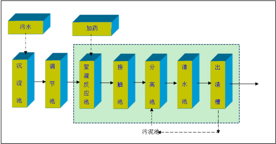
图 7.3-1 絮凝沉淀流程图
