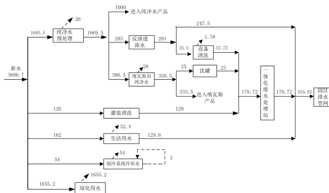
图 3.4-1 本项目水量平衡图 (单位: m 3 /a)
