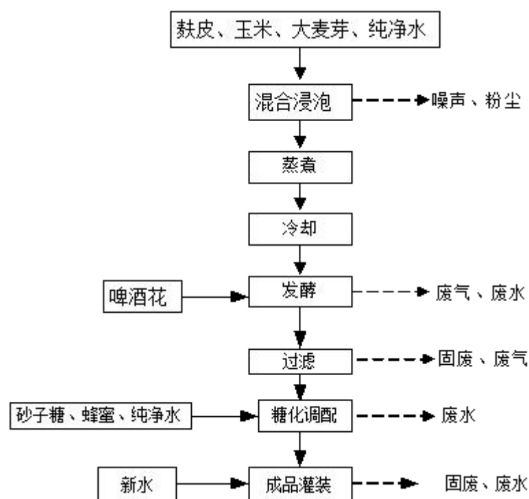
图 3.6-3 喀瓦斯生产工艺流程及产污节点图
