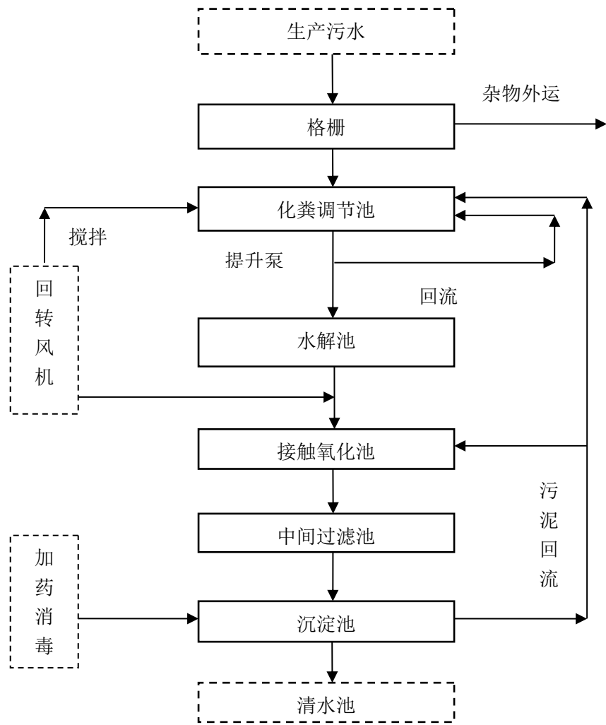
图 7.2-1 生产污水处理工艺流程图
