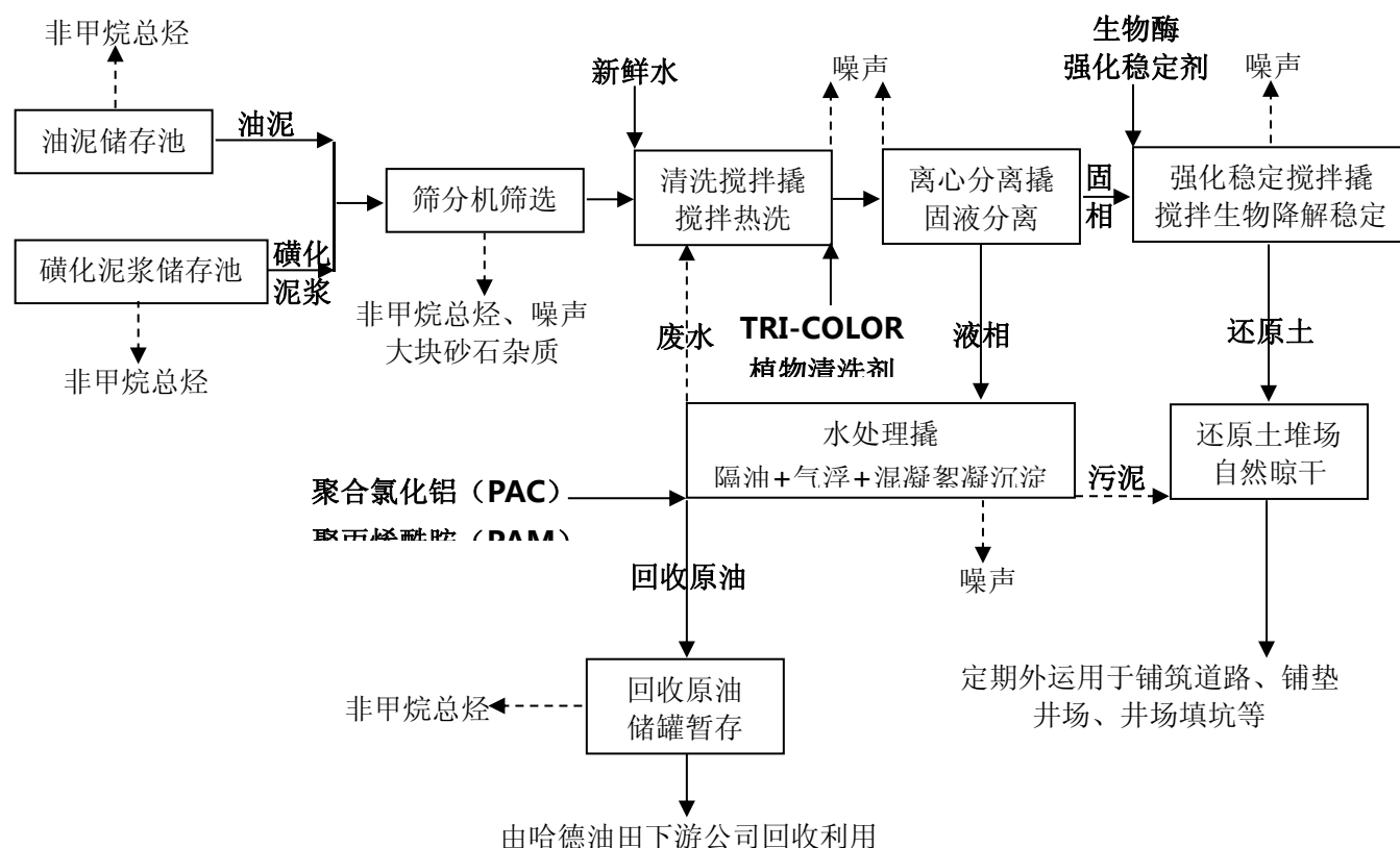
图 4-3 运营期工艺流程及产污环节示意图
