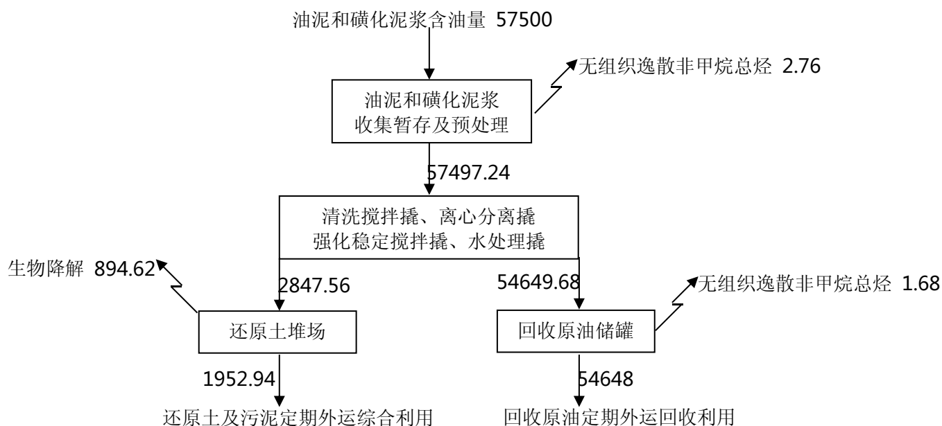
图 4-5 本项目油平衡分析示意图 单位：t/a
