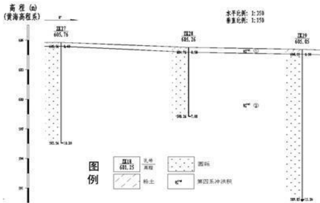
图 5.4-2 场地浅部包气带岩性特征
