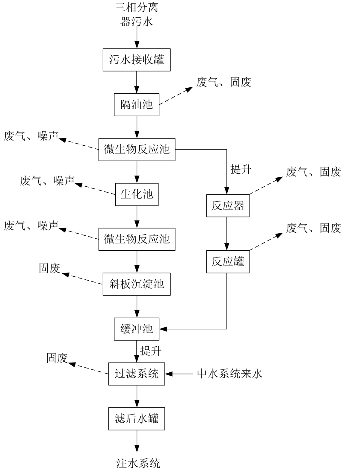
图 3.3-2 改造后污水处理工艺及产污环节图
