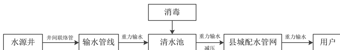
图 3-1 水厂供水流程图
