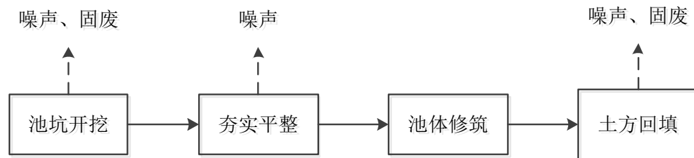
框图 3-2 清水池施工工序及产污环节图
