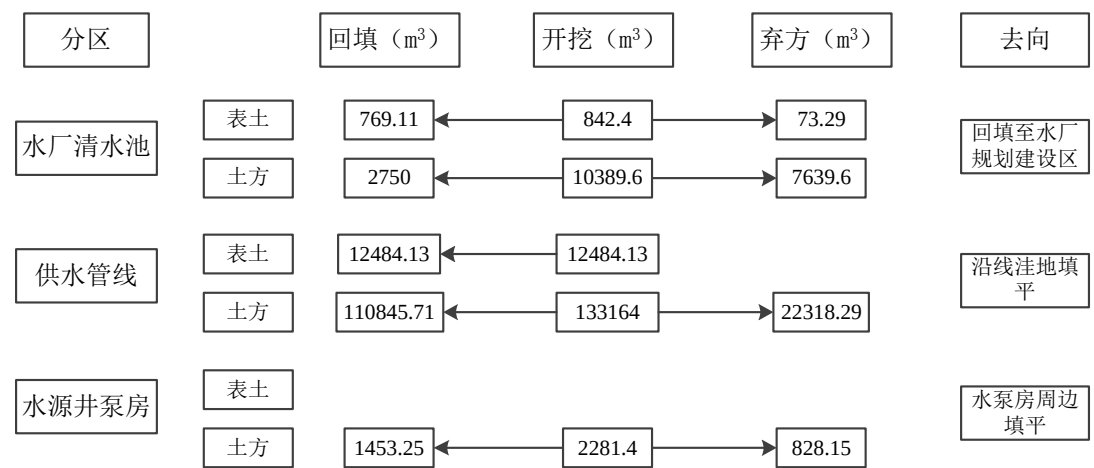
框图 3-6 土石方平衡图
