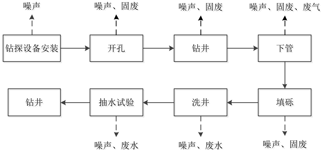
框图 3-3 供水井施工工序及产污环节图
