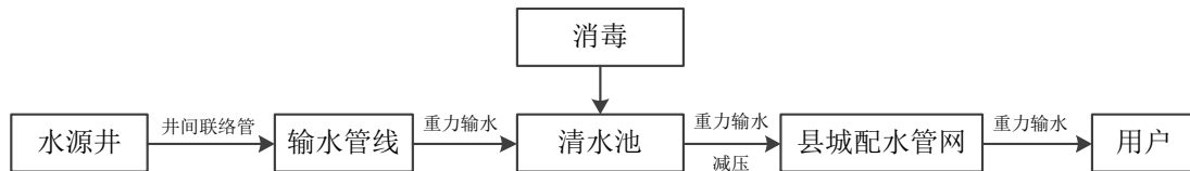
框图 3-5 运营期生产工艺流程及产污环节图
