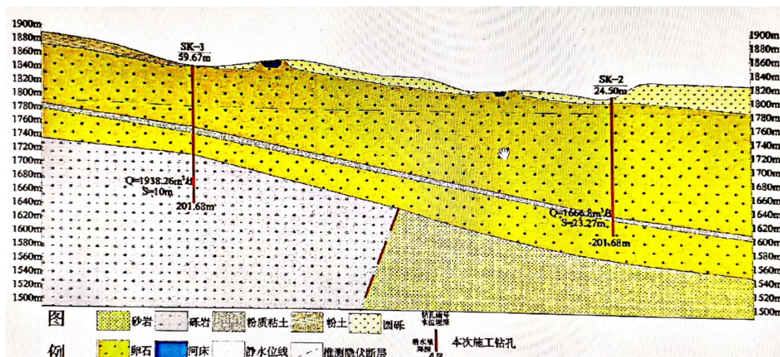
图 5.6 钻孔水文地质剖面图
