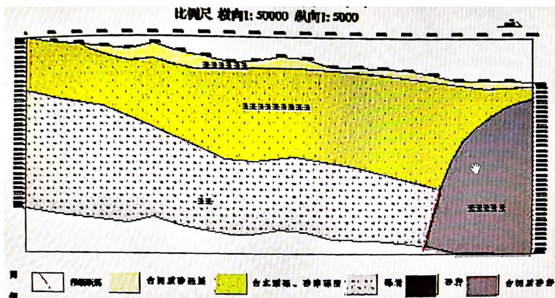
图 5.5.4 线推断解释断面图
