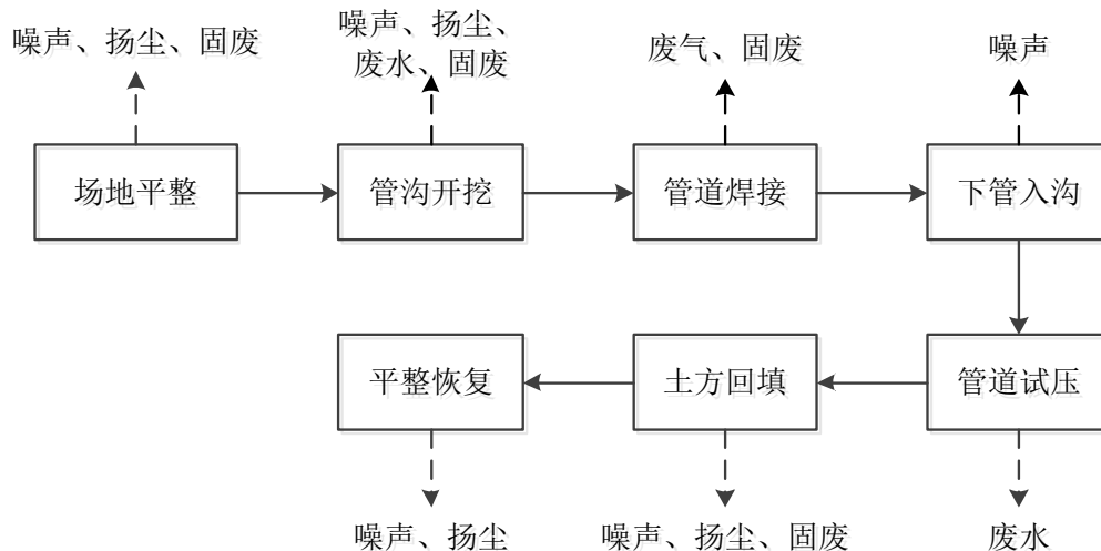
框图 3-4 管线施工工序及产污环节图
