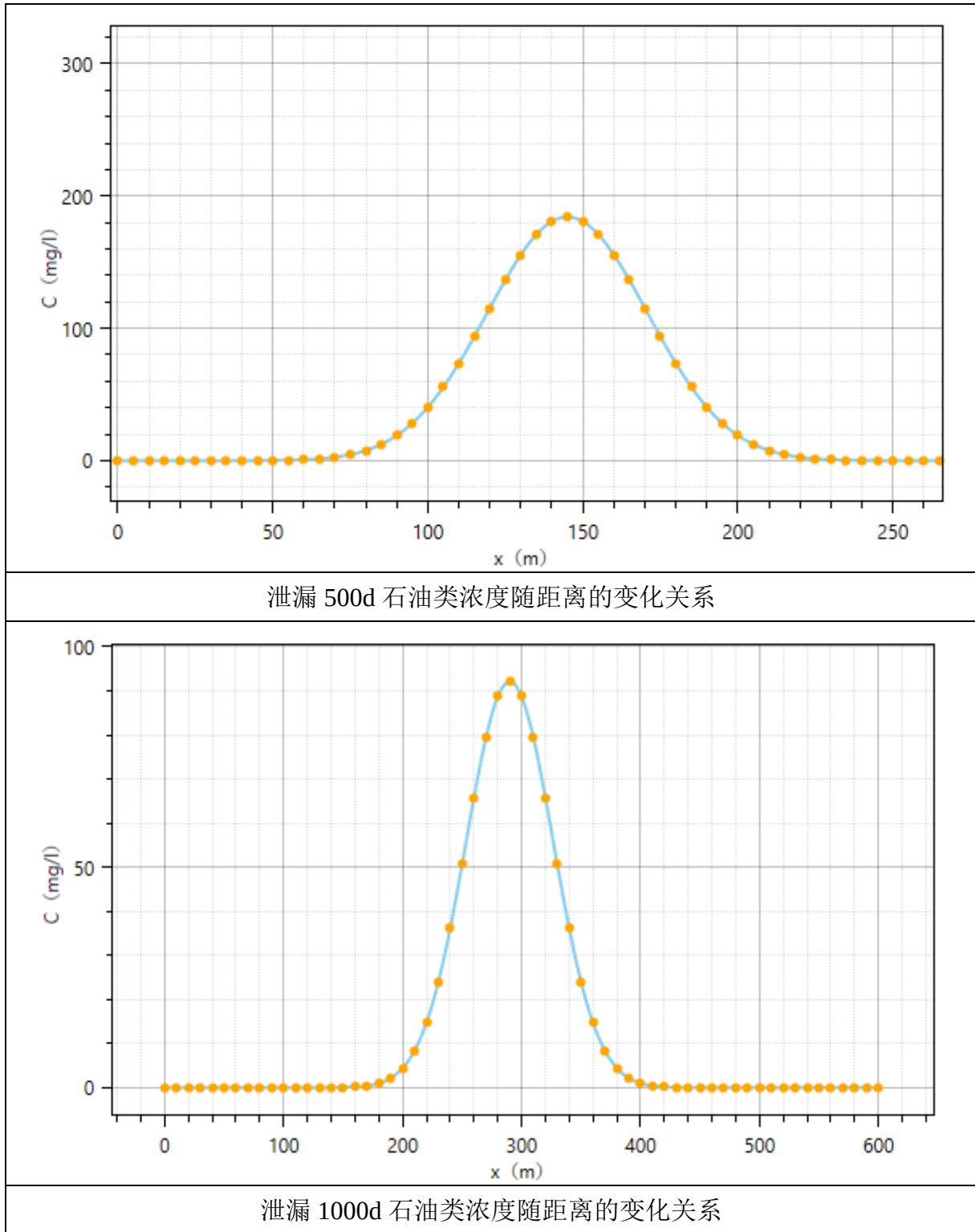
图 4.3-2 储油罐发生全管径泄漏时石油类浓度随距离的变化关系
