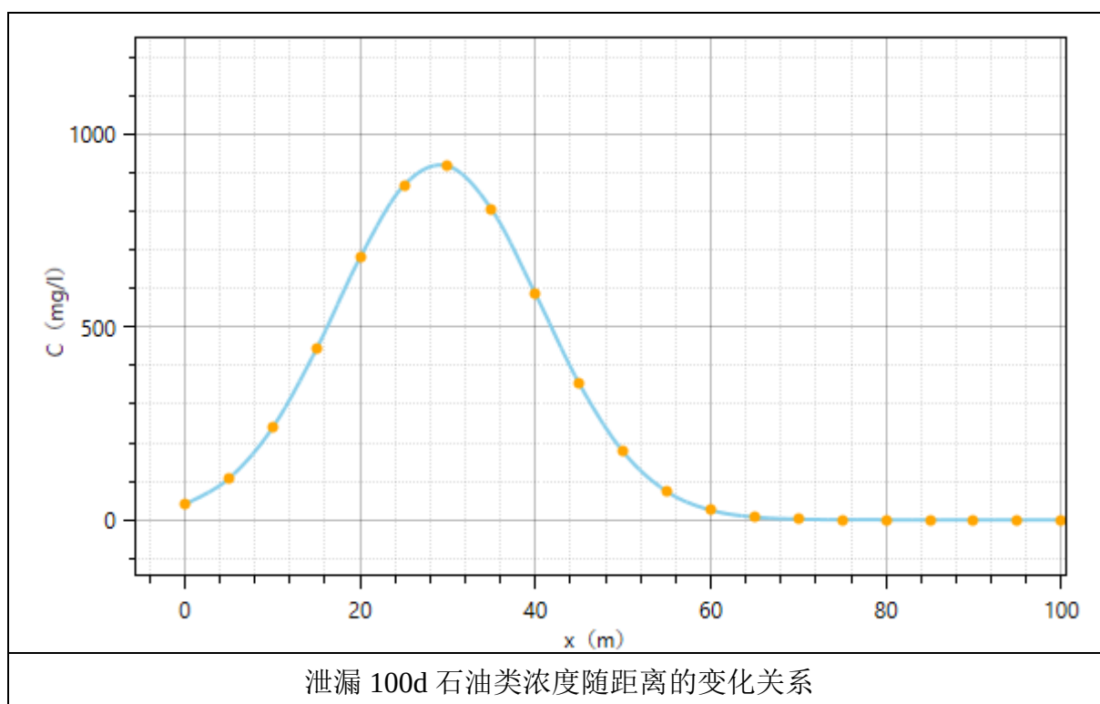
图 4.3-1 集输管线发生全管径泄漏时石油类浓度随距离的变化关系
