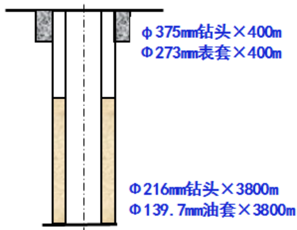
图 2.3-3-1 条 34 块井身（水平井）结构示意图
