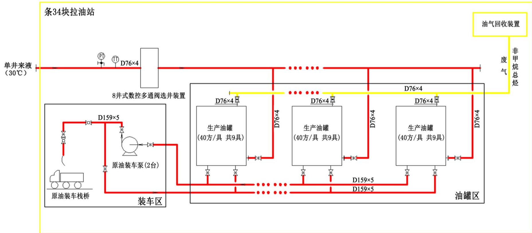
图 2.3-5 项目油气集输工艺流程图
