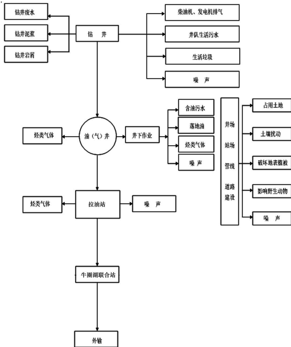
图 2.4-1 油田开发过程污染物排放流程
