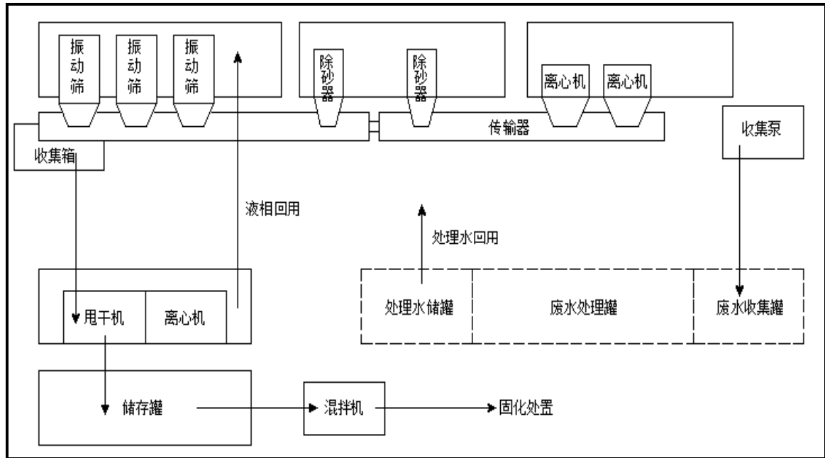
图 6.5-1 不落地处理系统工艺流程图
