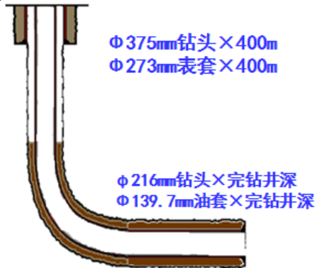
图 2.3-3-1 条 34 块井身（水平井）结构示意图
