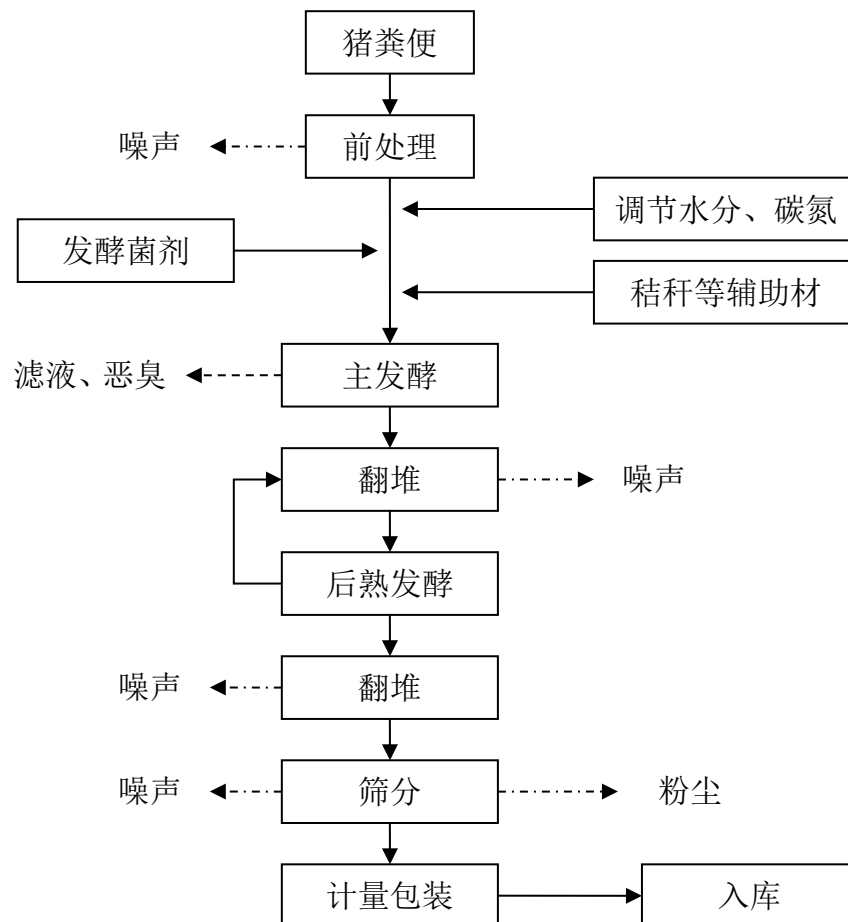
图3.1-7 堆肥工艺流程及产污环节
