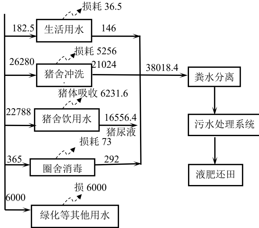
图3-1-2 项目水量平衡图(单位: t/a)
