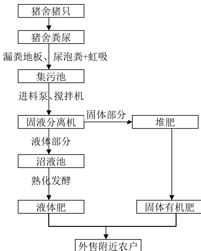
图 3.1-5 粪肥处理利用工艺流程图
