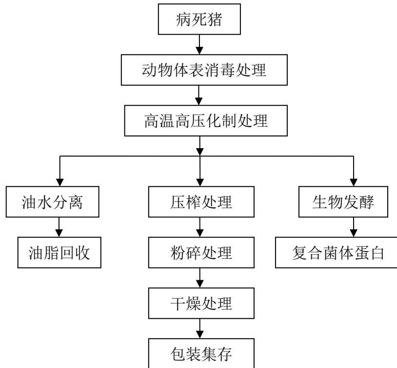
图3.1-8 项目病、死猪尸体无害化处理工艺图
