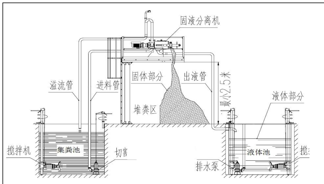
图 3.1-6 固液分离系统断面示意图
