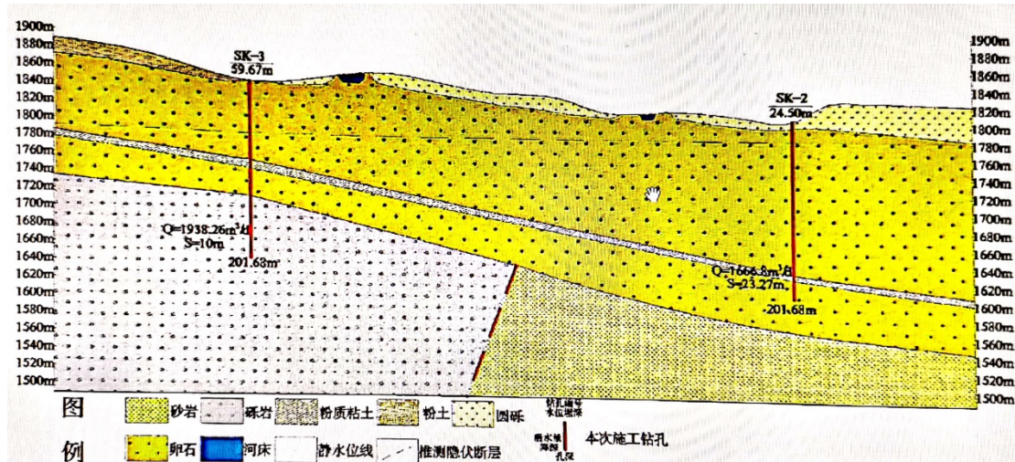
图 4.6 钻孔水文地质剖面图
