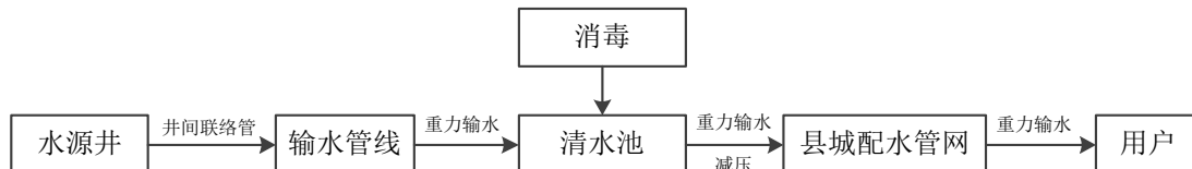
框图 2-5 运营期生产工艺流程及产污环节图
