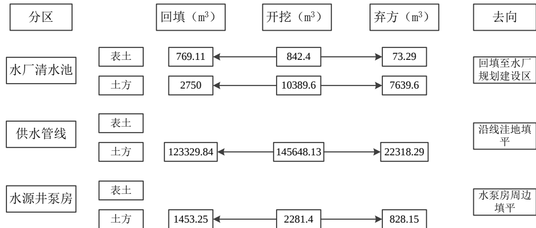
框图 2-6 土石方平衡图
