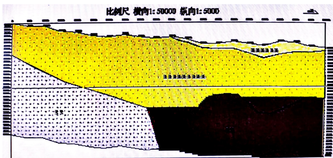
图 4.4.3 线推断解释断面图
