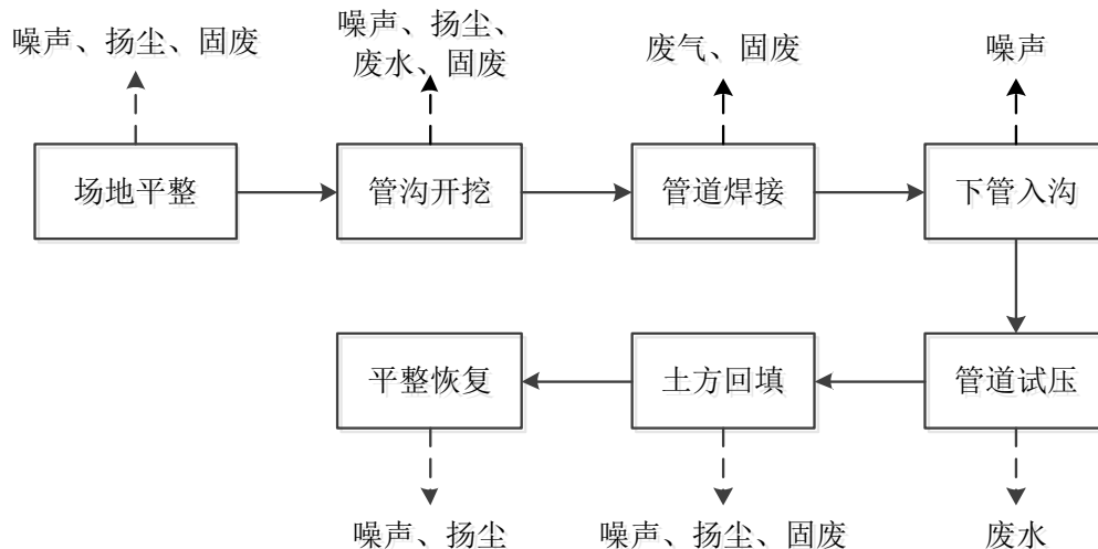
框图 2-4 管线施工工序及产污环节图
