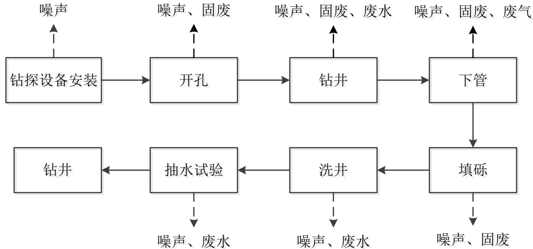
框图 2-3 供水井施工工序及产污环节图
