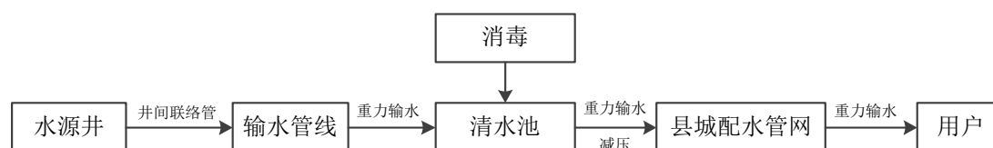
图 2-1 水厂供水流程图
