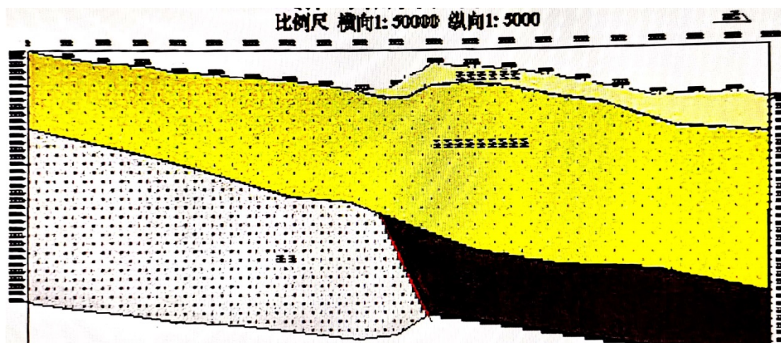
图 4.2.2 线推断解释断面图
