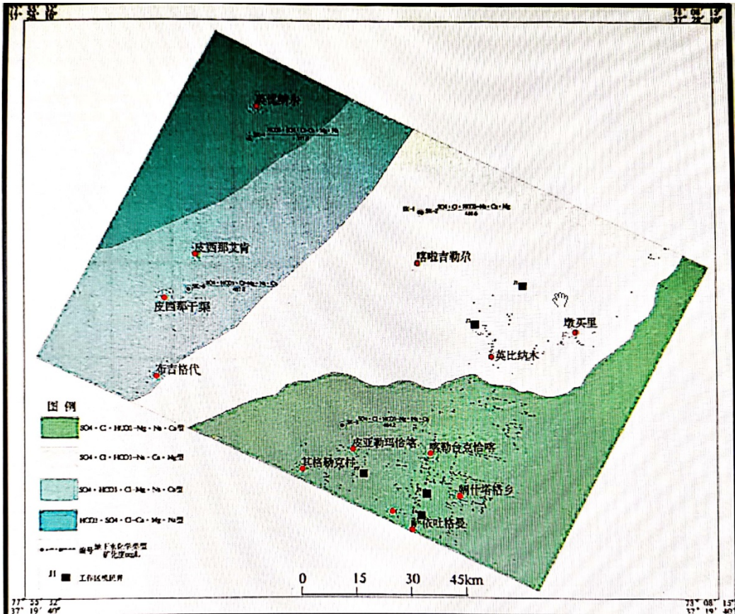
图 4.7 工作区地下水化学图
