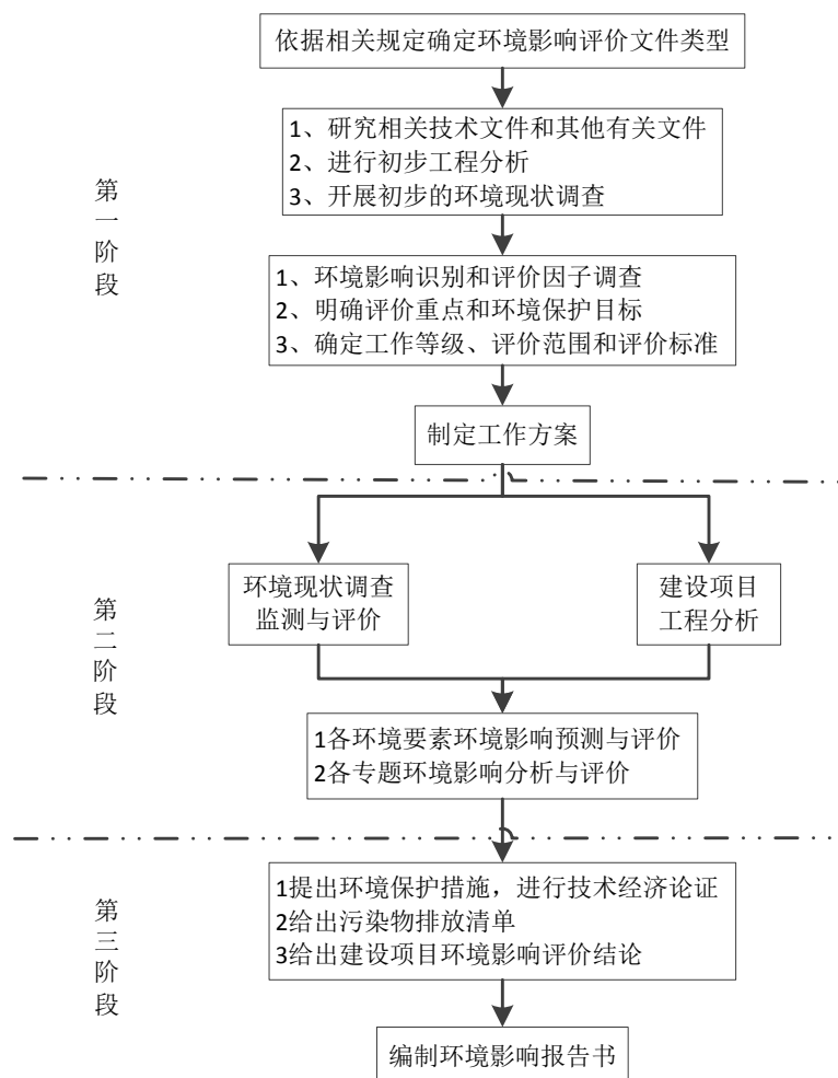
图 1-1 环境影响评价工作程序图
