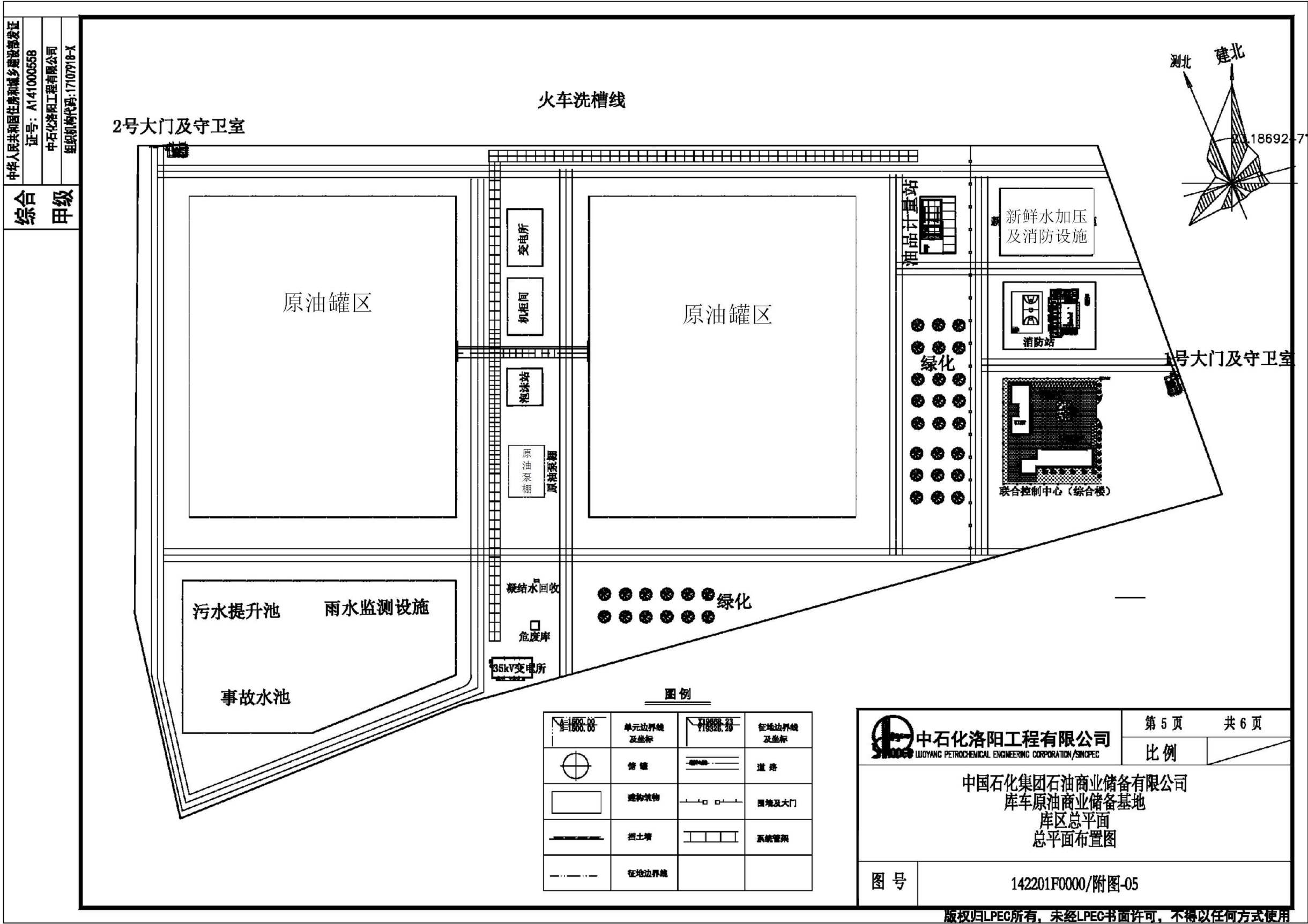
图 4. 1-3 本项目平面布置图
