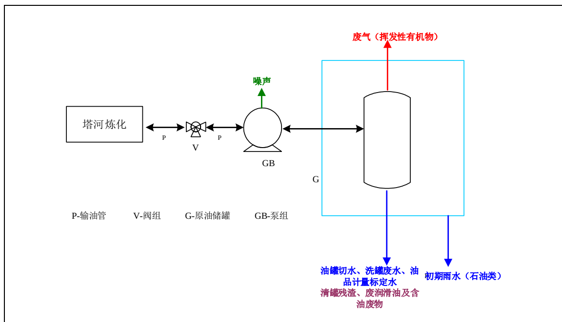
图 4.6-2 本项目运营期产污环节图
