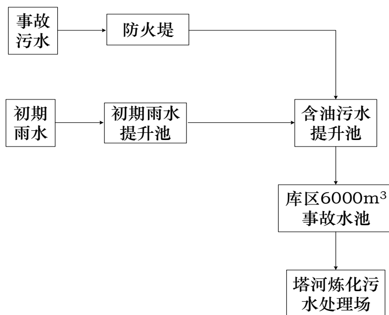
图 7.6-1 事故污水调储系统示意图
