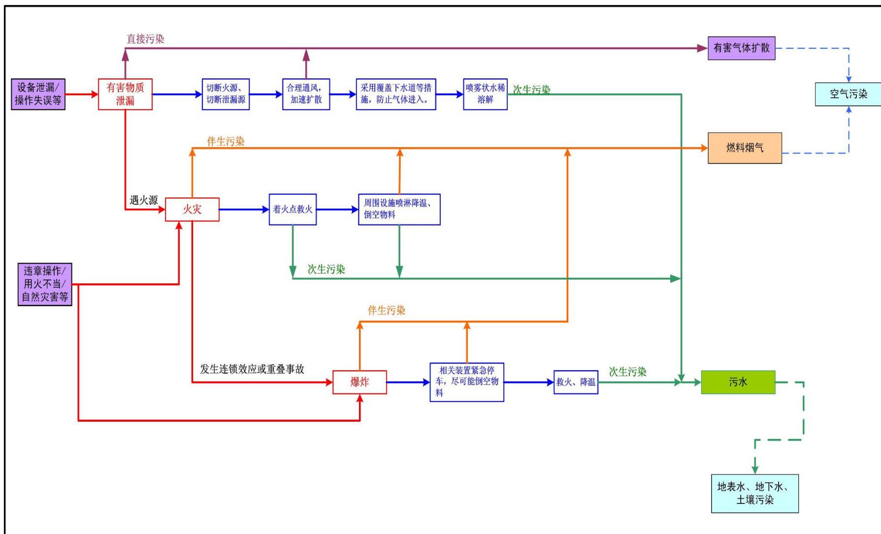
图 7.5-1 紧急事故处置措施及污染物输送途径示意图
