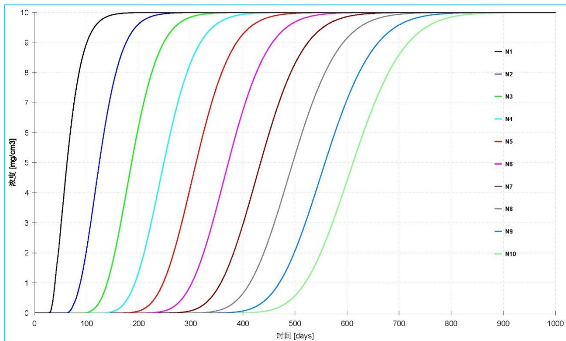
图 6.2—30 各观测点耗氧量的浓度随时间变化
