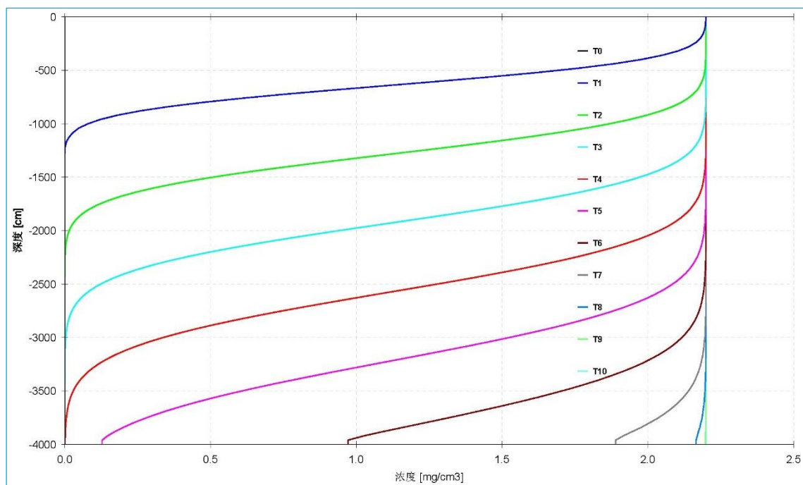
图 6.2—29 各时间点石油类的浓度随深度变化
