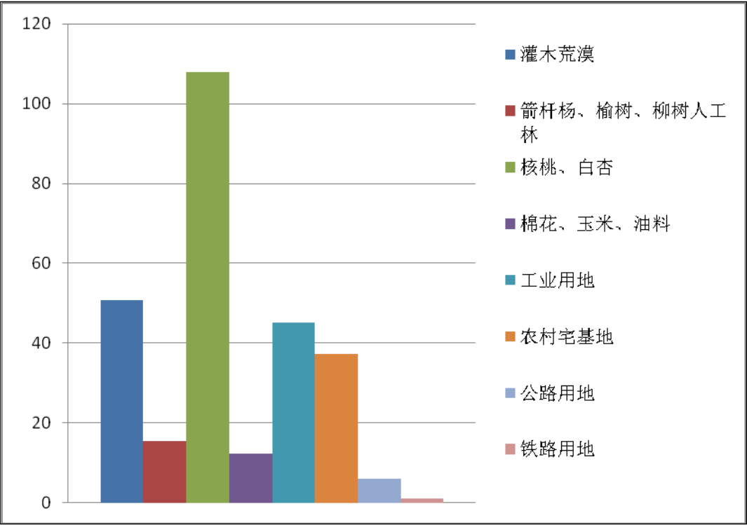
图 5.2-6 库区评价范围内植被类型现状统计图
