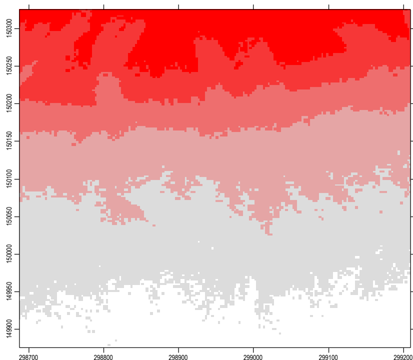
图 6.2-24 评价区地形示意图
