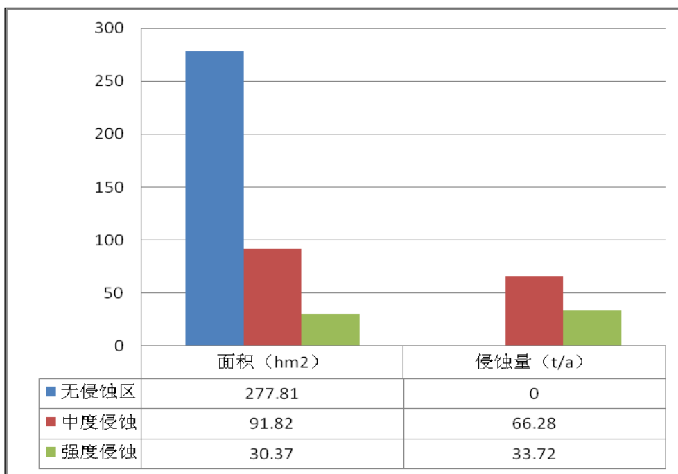
图 5.2-9 库外管线评价范围内土壤侵蚀现状统计图
