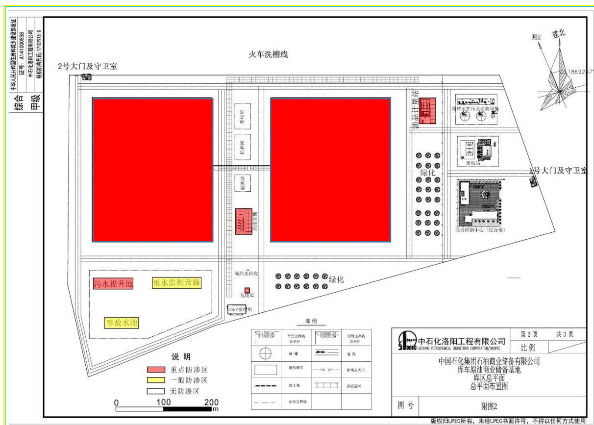
图 9.3—2 油库项目区分区防渗示意图
