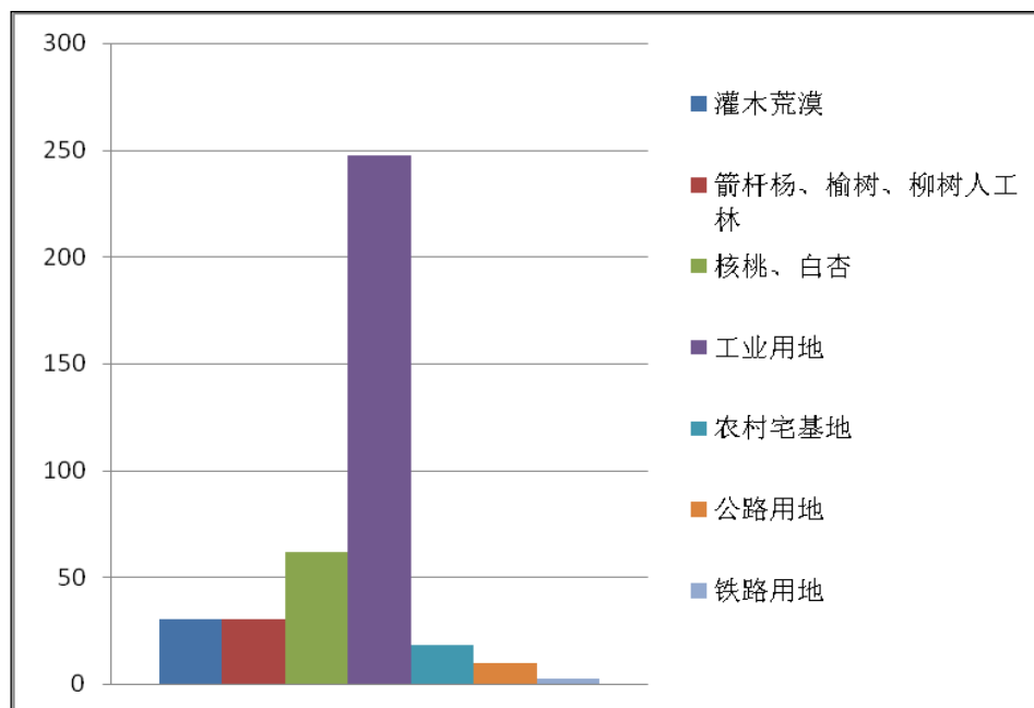
图 5.2-7 库外管道评价范围内植被类型现状统计图
