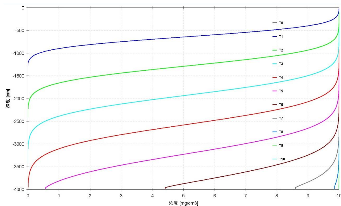
图 6.2—31 各时间点耗氧量的浓度随深度变化
