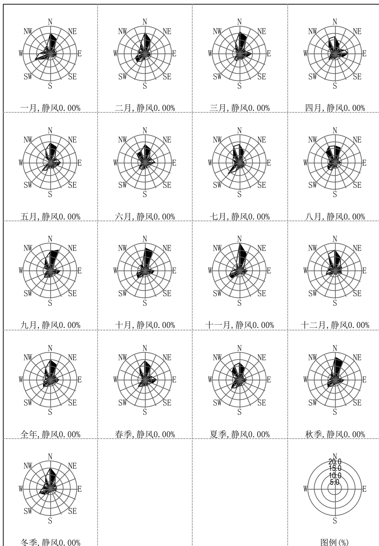
图 6.2—23 库车县气象站 2017 年风频玫瑰图
