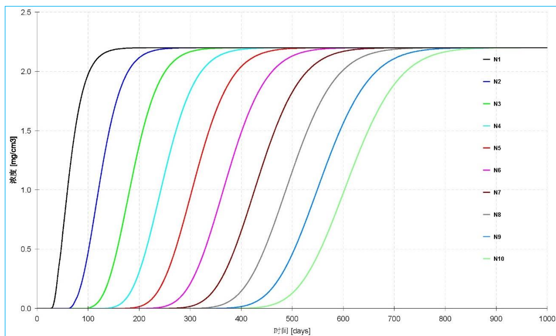
图 6.2—28 各观测点石油类的浓度随时间变化
