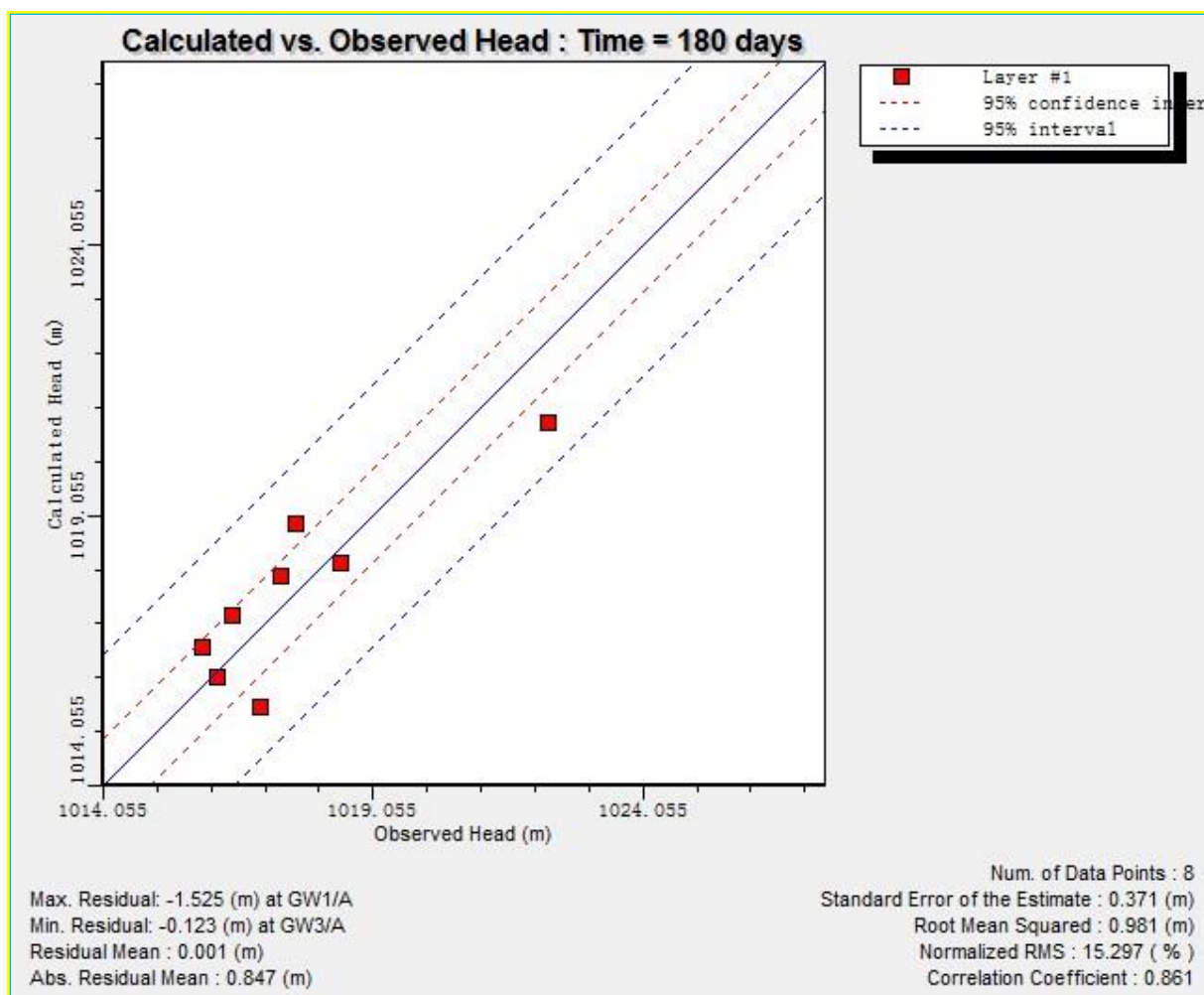
图 6.2—4 计算和观测水位拟合结果对比
