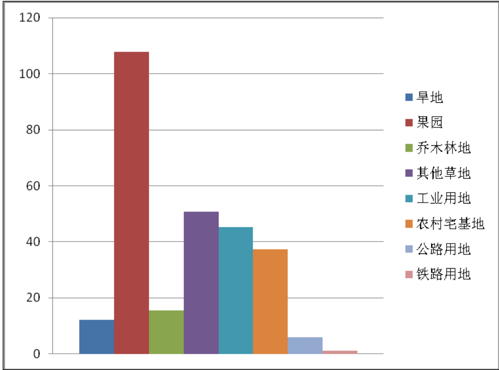
图 5.2-4 库区评价范围内土地利用类型现状统计图
