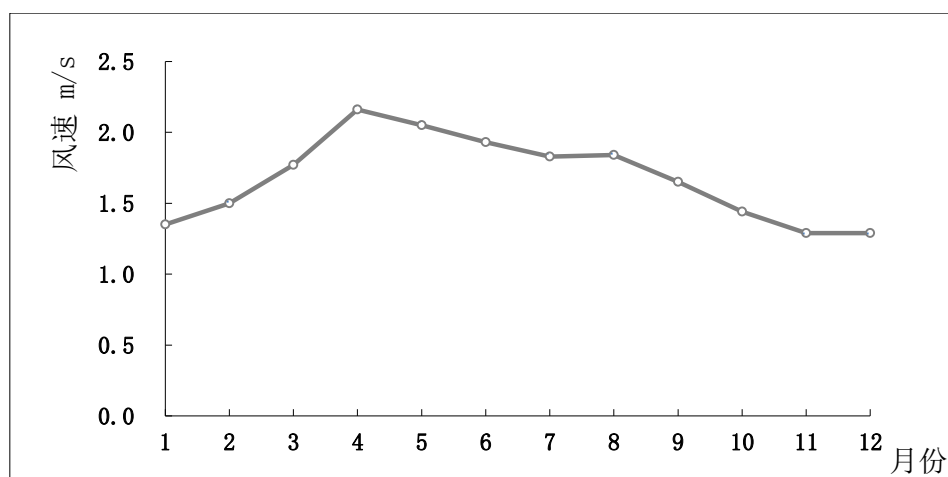
图 6.2—21 库车县气象站 2017 年各月平均风速
