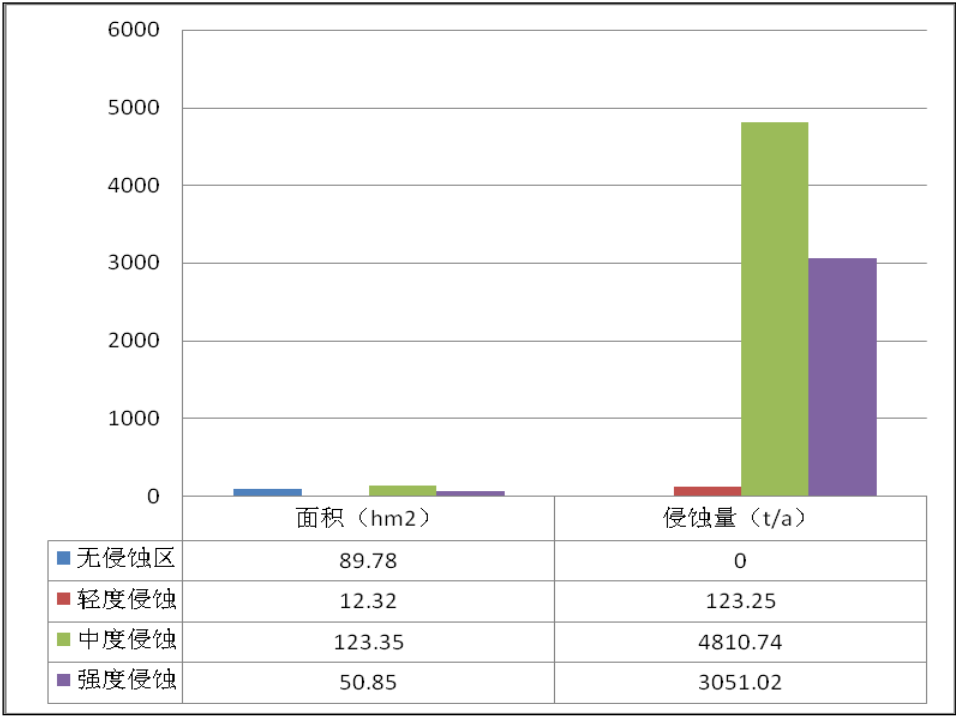
图 5.2-8 库区评价范围内土壤侵蚀现状统计图
