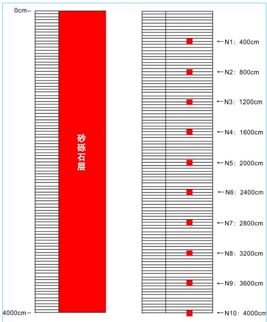
图 6.2—27 包气带分层、剖分和观测点位置
