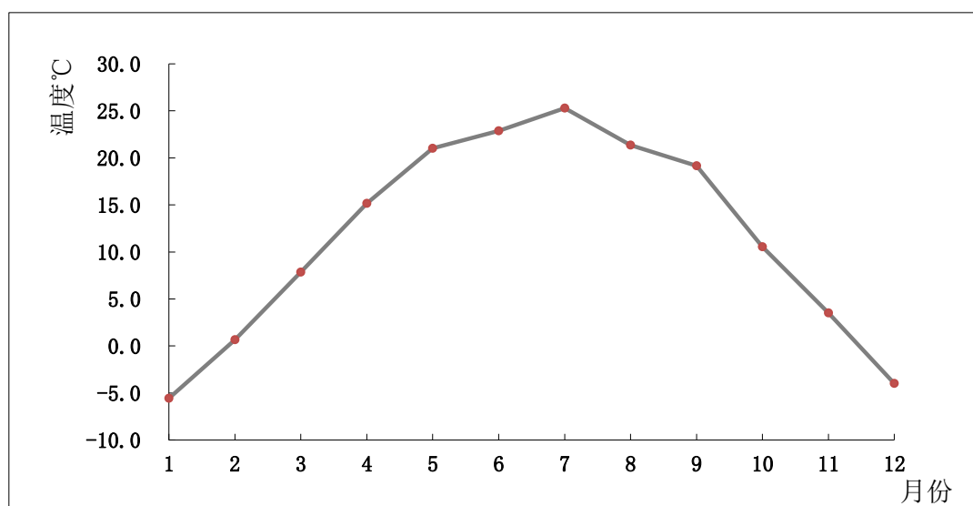
图 6.2—22 库车县气象站 2017 年各月平均气温
