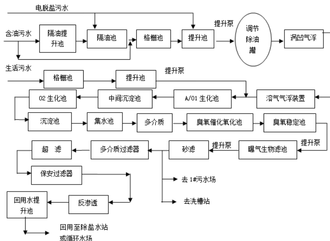
图 3.1-1 2#污水处理场及污水回用设施工艺流程图
