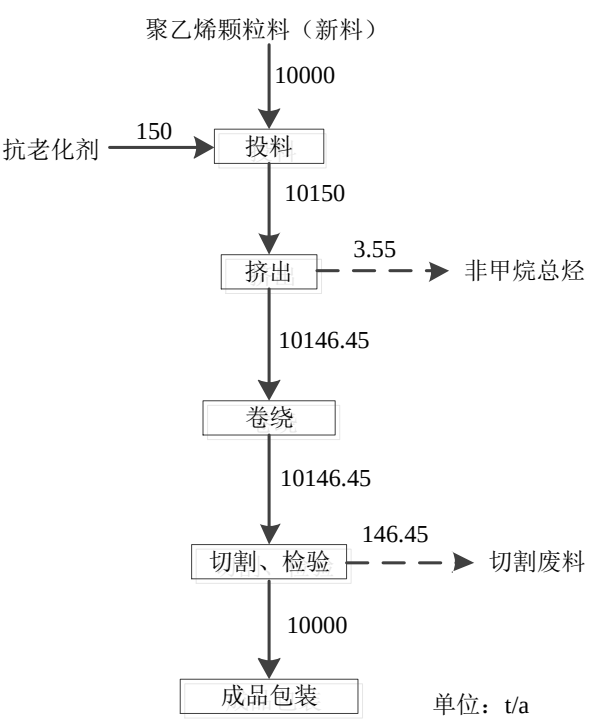
图3.4-3 地膜生产物料平衡图
