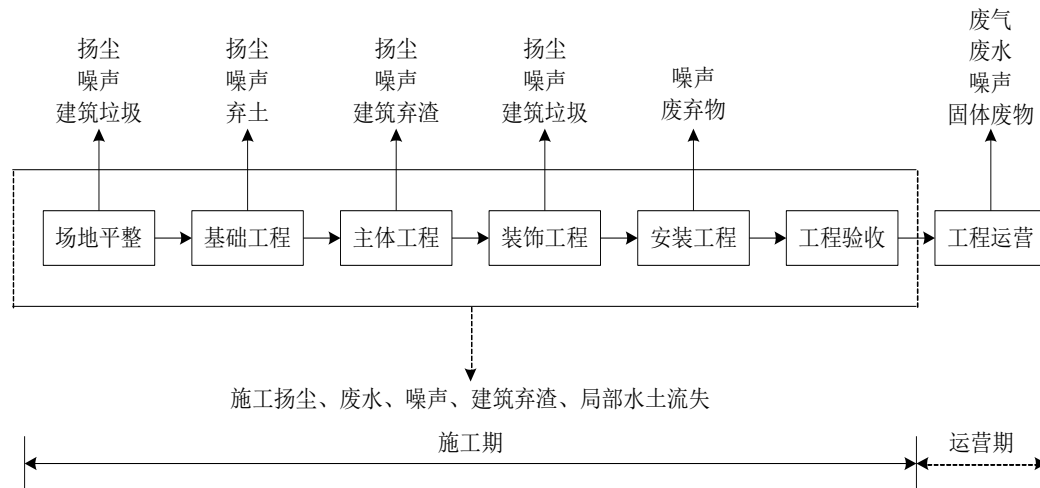
图3.3-1 项目施工期工艺流程及产污节点图
