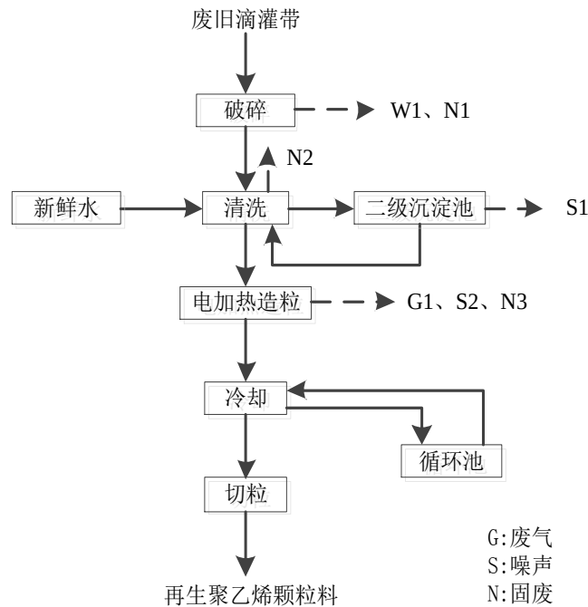
图 3.3-1 再生塑料颗粒工艺流程及产污环节图
