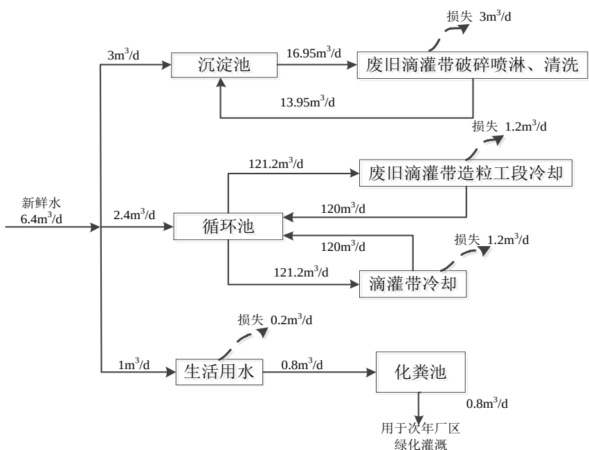
图3.4-4 水平衡图
