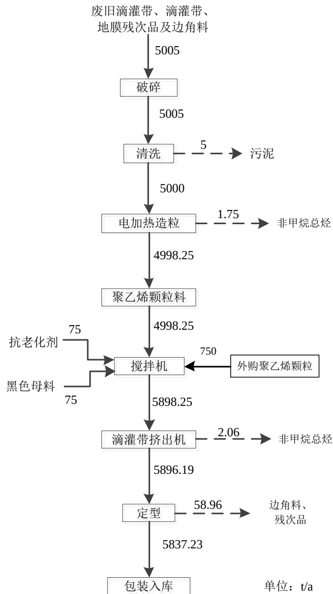
图3.4-2 废旧塑料加工及滴灌带生产物料平衡图
