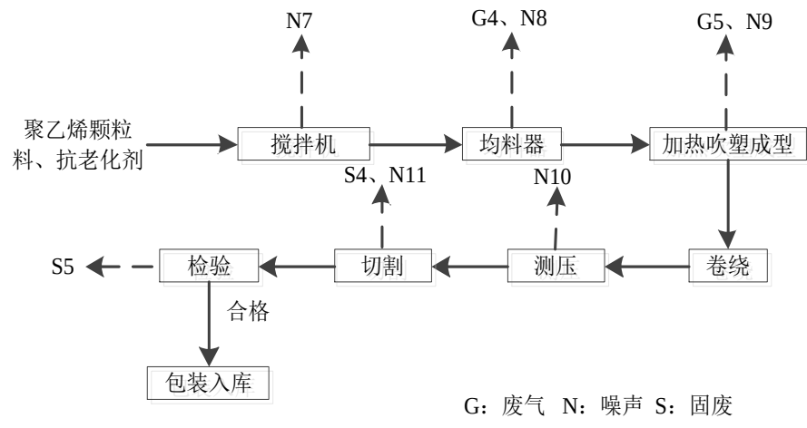
图3.3-3 地膜加工工艺流程及产污环节图
