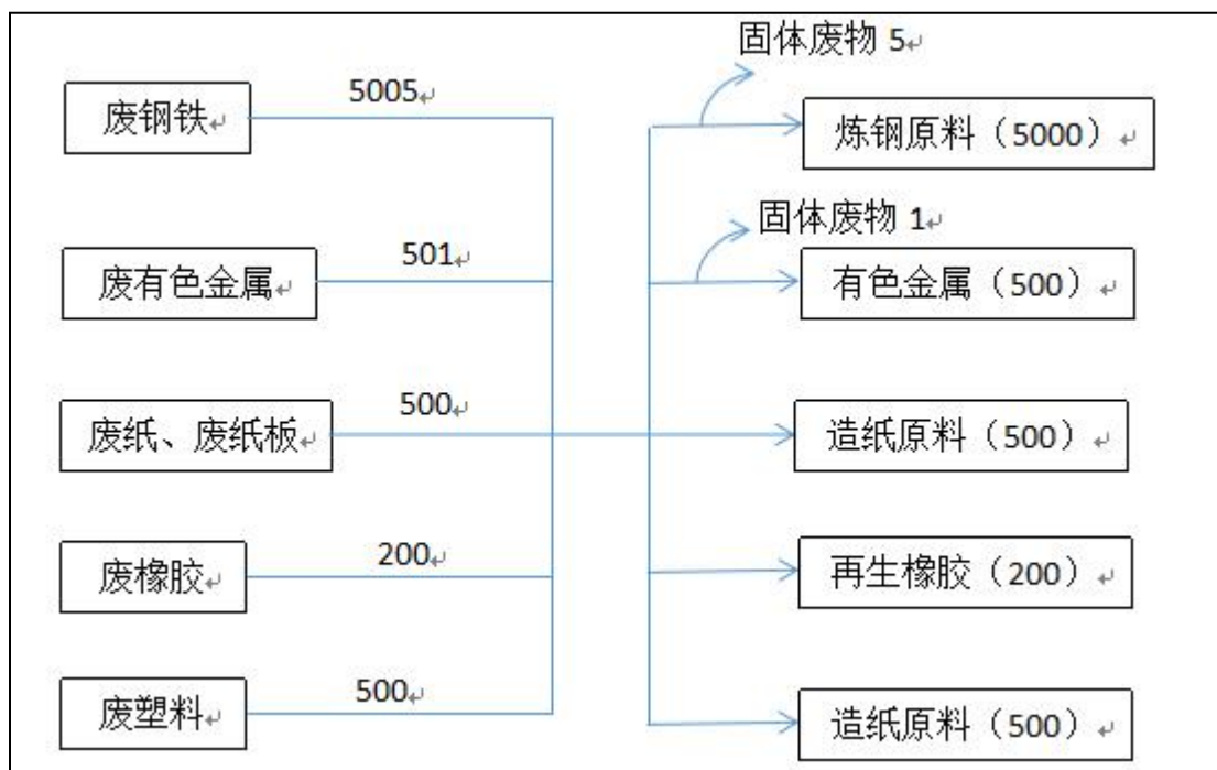
图 2.1-1 项目物料平衡图 (单位: t/a)
