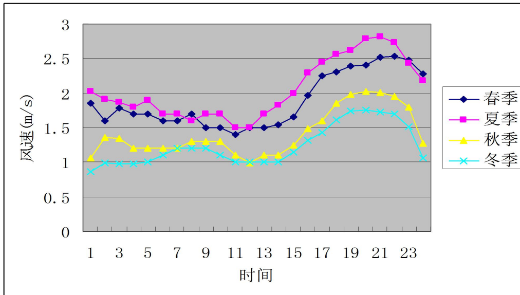
图 4.2-1 平均风速月变化曲线图
