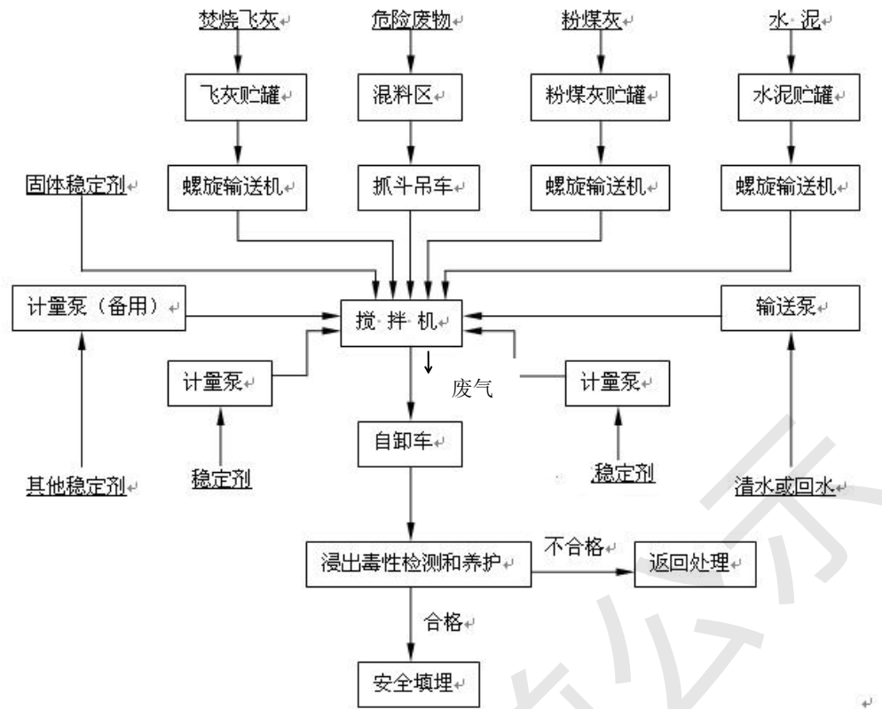
图 3.1-4 稳定固化工艺流程及产污节点图
