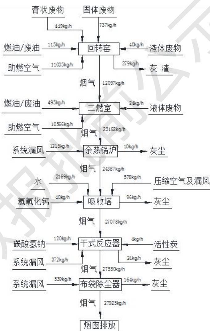
图 3.1-1 焚烧系统工艺流程及产物节点图
