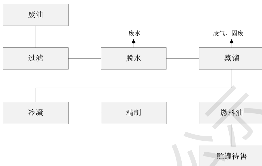
图 3.1-3 废油处置工艺及产物节点图
