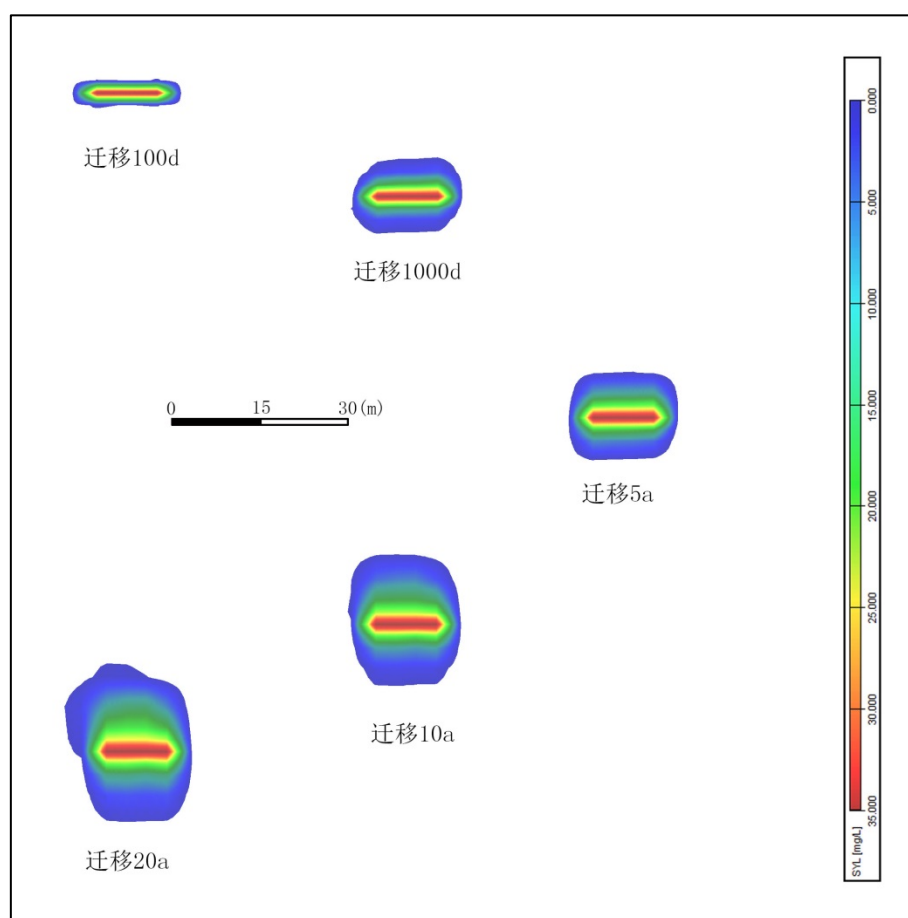
图 5.3-22 正常情况下氨氮迁移平面图
