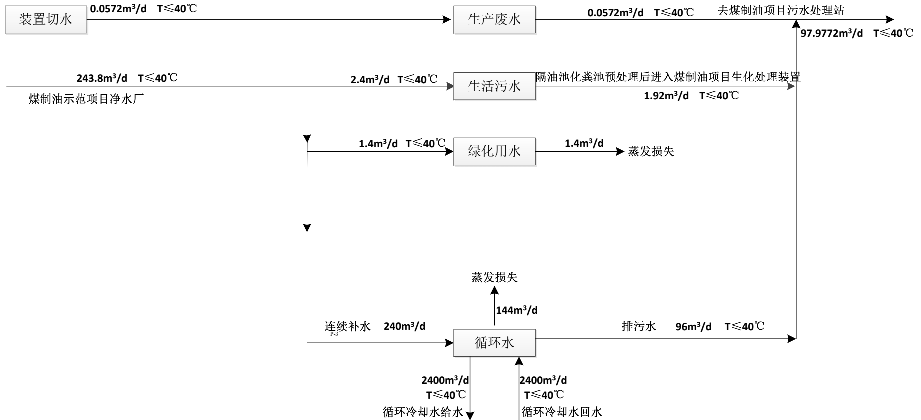
图 3.2-2 烷基苯项目水平衡示意图
