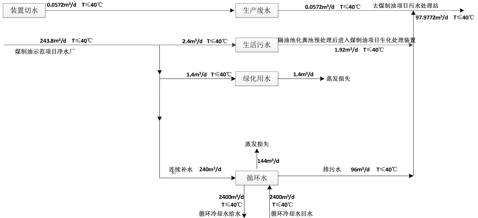
图3.3-7 烷基苯项目水平衡示意图
