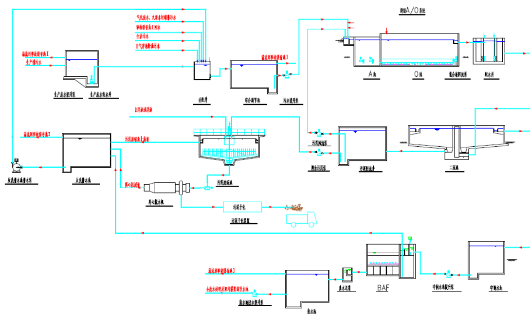
图 7.2-2 污水处理场工艺流程图（生化污水处理）
