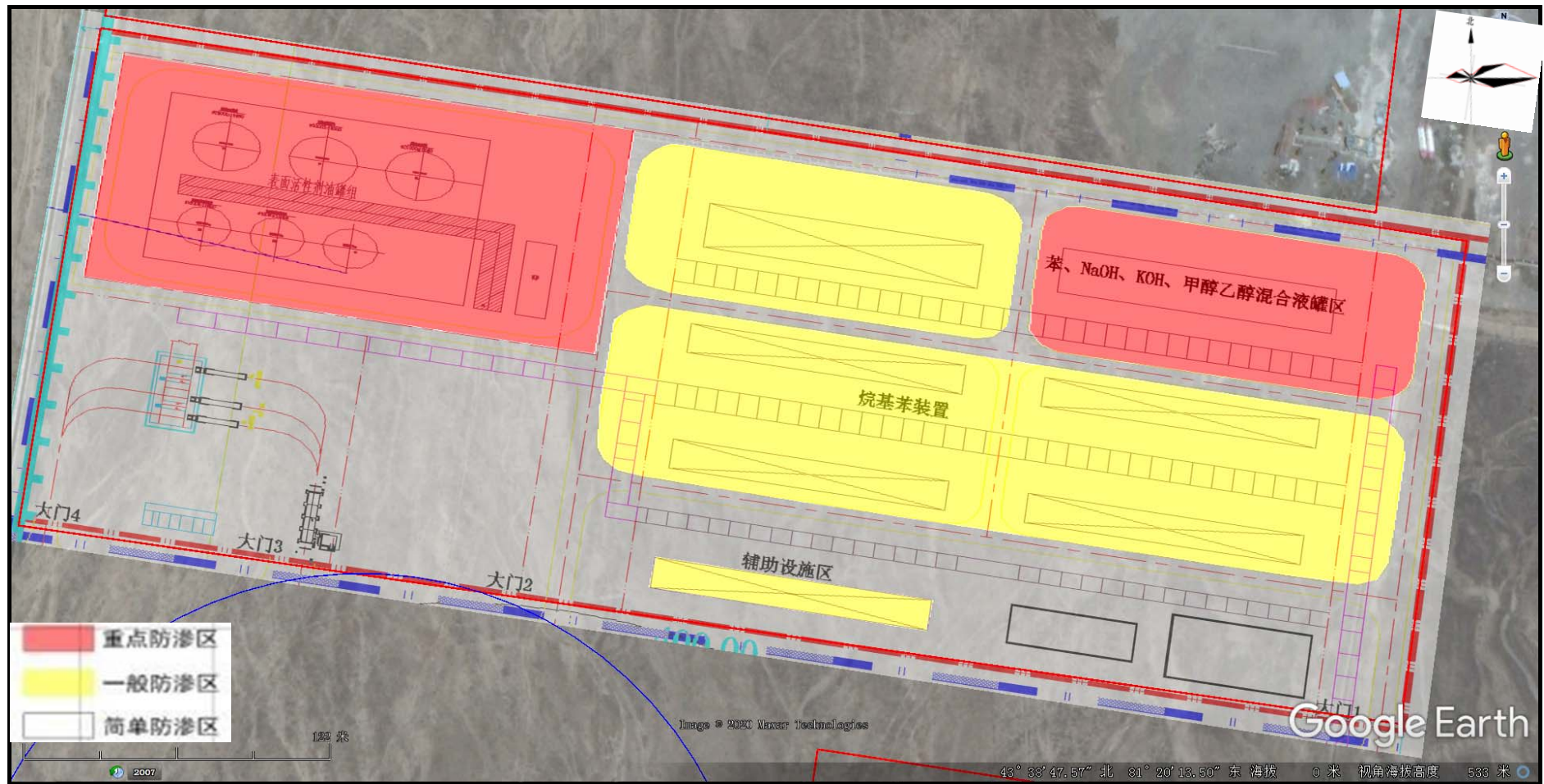
图 7.2-4 地下水污染防渗分区图
