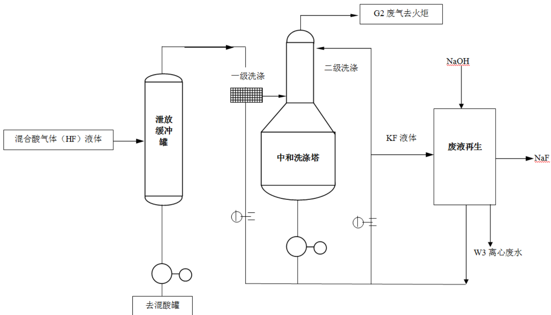
图 3.3-5 中和工序工艺流程及产污节点图
