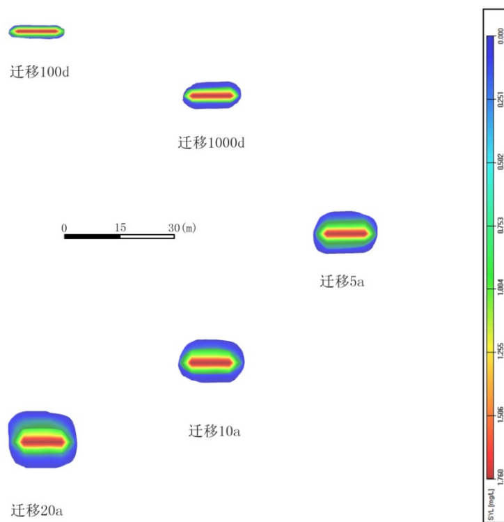
图 5.3-26 正常情况下氟化物迁移平面图
