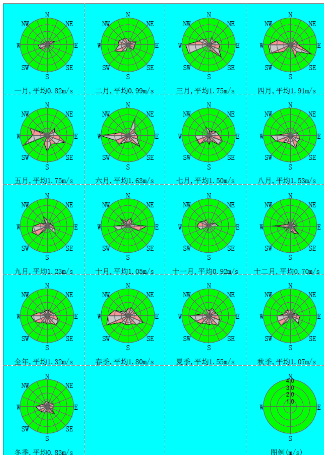
图 5.1-3 伊宁市 2018 年风频玫瑰图
