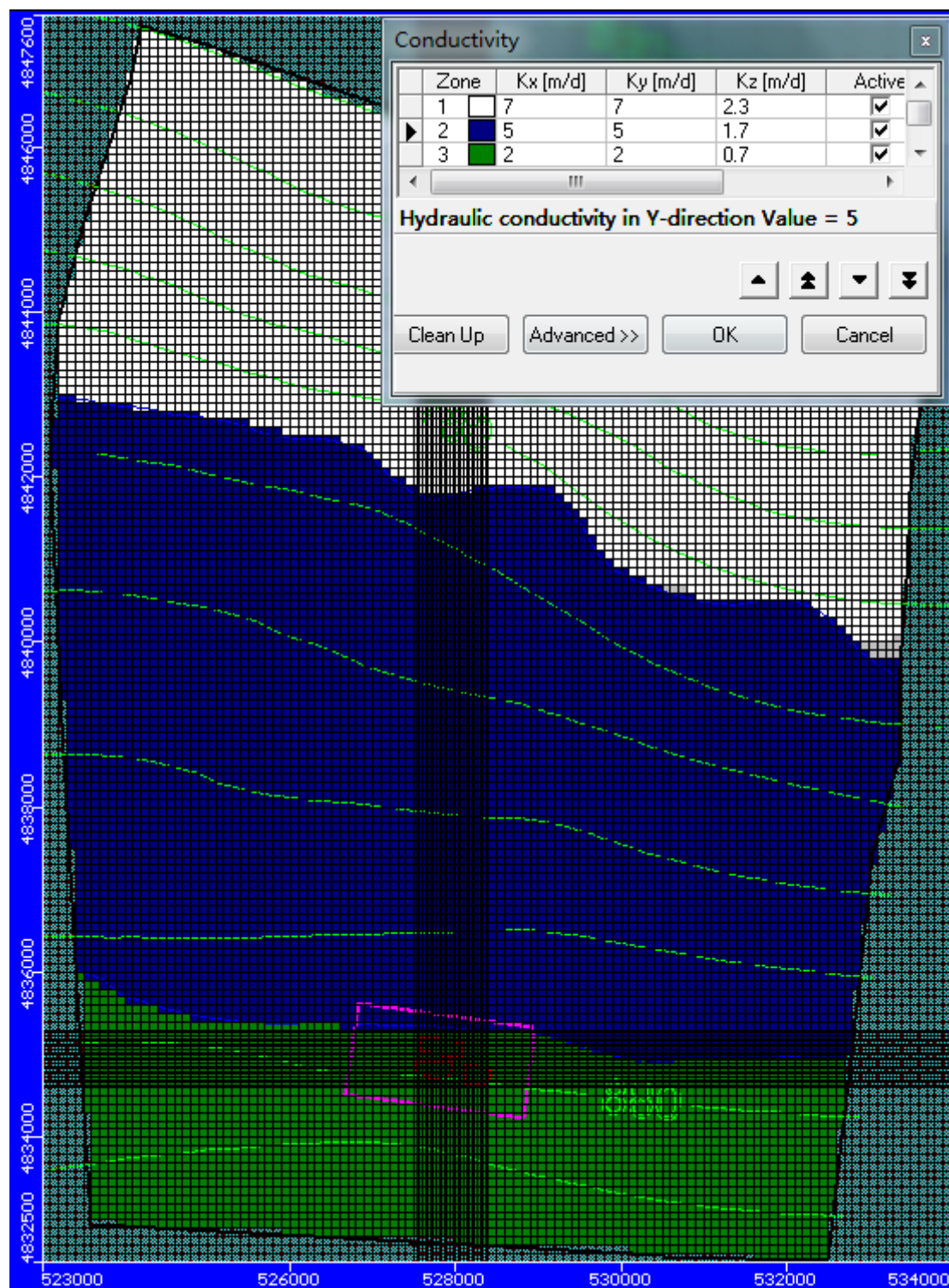
图 5.3-14 模型中初始渗透系数分区图
