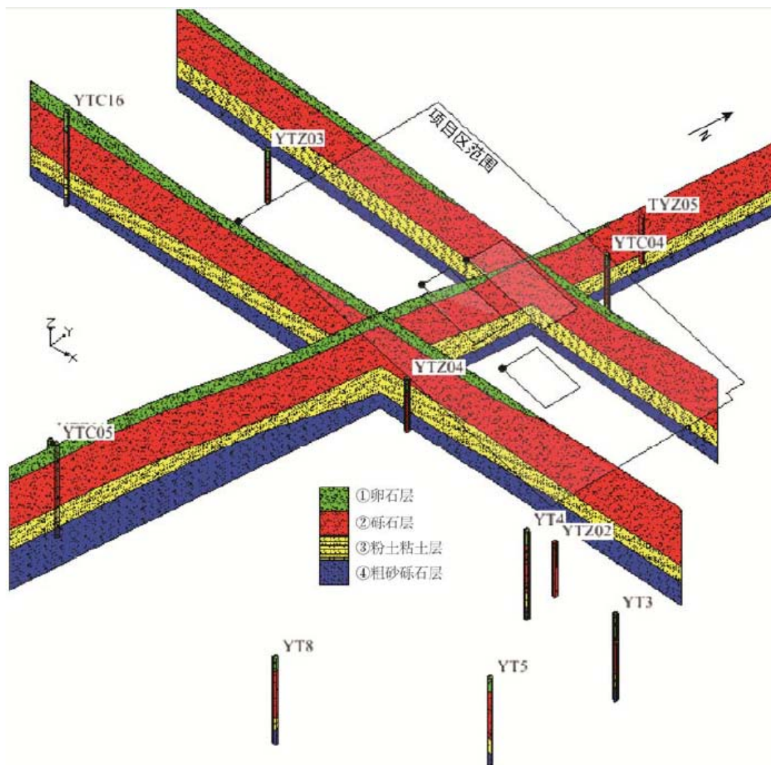
图 5.3-12 项目区地质实体三维视图
