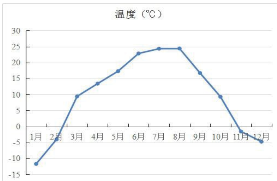
图 5.1-1 伊宁市 2018 年月平均温度变化图
