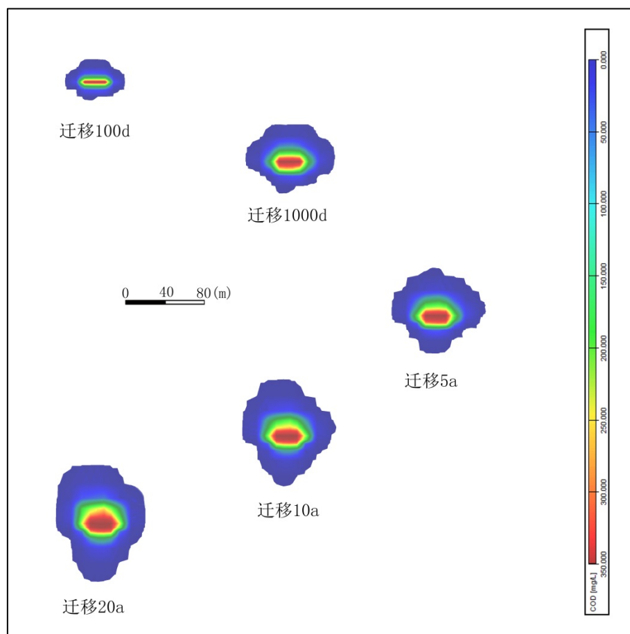
图 5.3-20 非正常情况下 COD 迁移平面图
