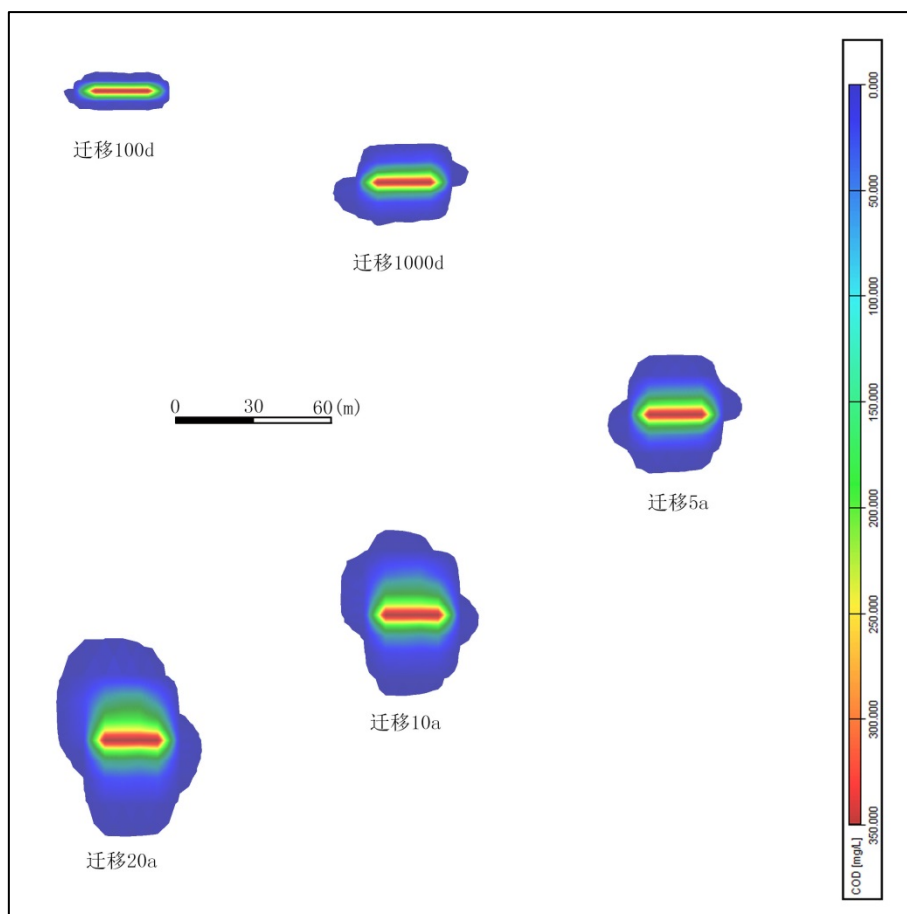
图 5.3-18 正常情况下 COD 迁移平面图
