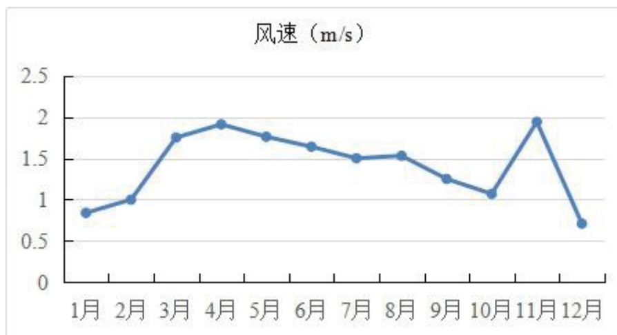
图 5.1-2 伊宁市 2018 年月平均风速变化图
