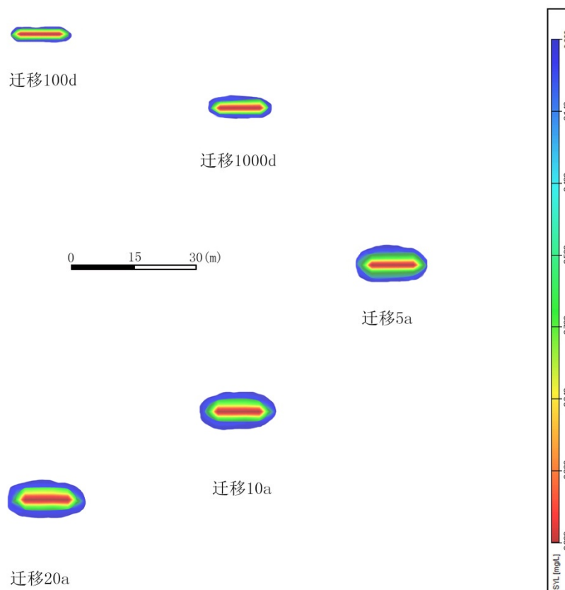
图 5.3-30 正常情况下苯迁移平面图
