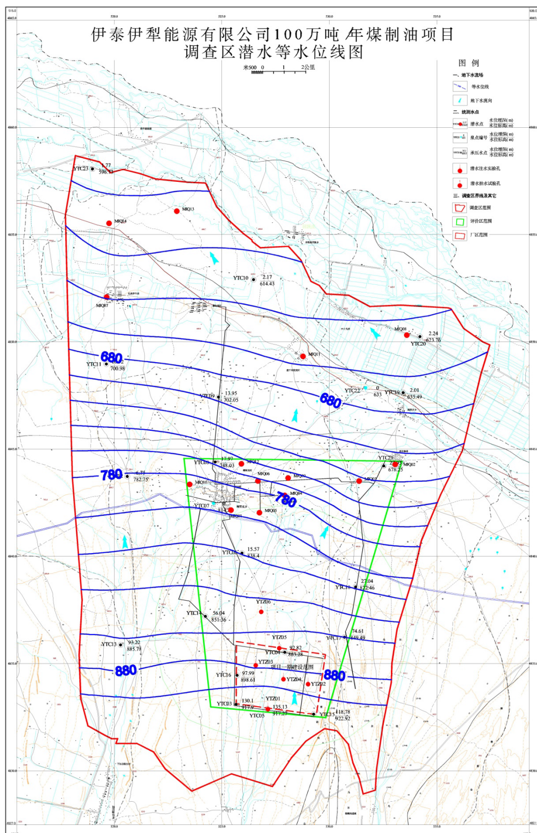
图 5.3-3 调查区潜水等水位线图
