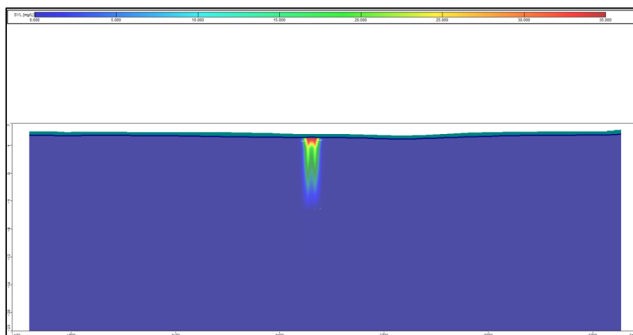
图 5.3-25 正常情况下 a-a'剖面图（氨氮迁移 20a 扩散图）
