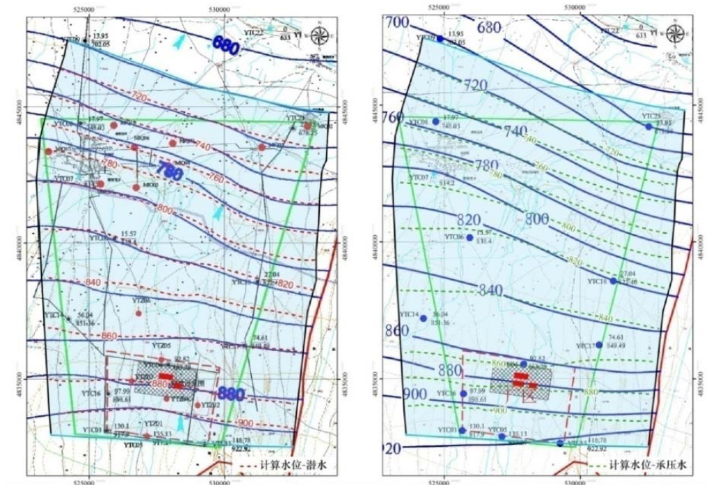
图 5.3-16 模拟等水位线与实测等水位线对比图（左潜水层、右承压水层）
