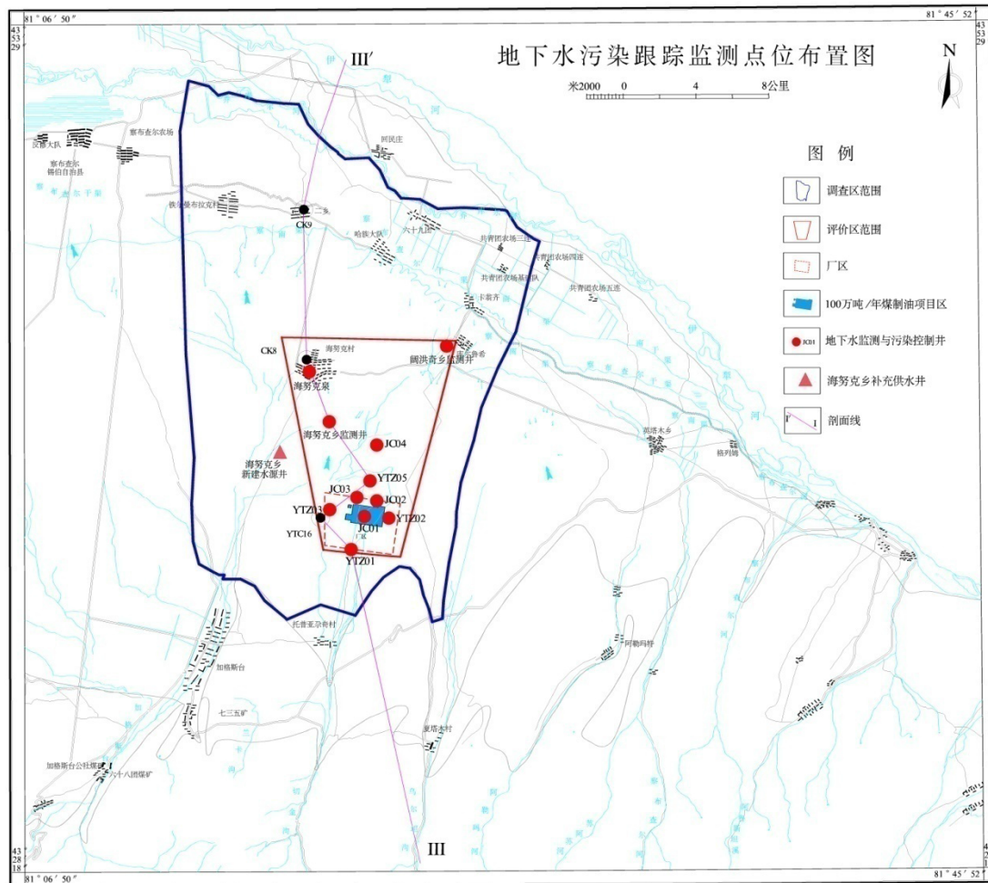
图 7.2-5 地下水跟踪监测井布置示意图
