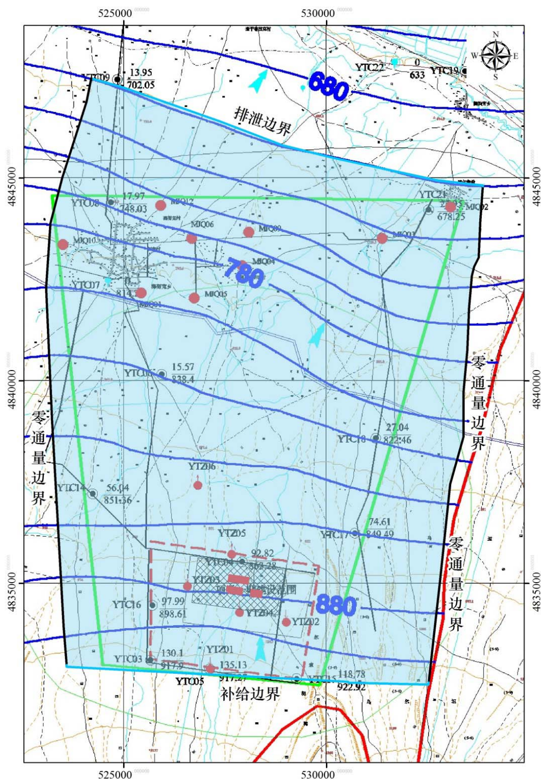
图 5.3-11 地下水模型范围及边界（图中黑色和浅蓝色线条包围区域）
