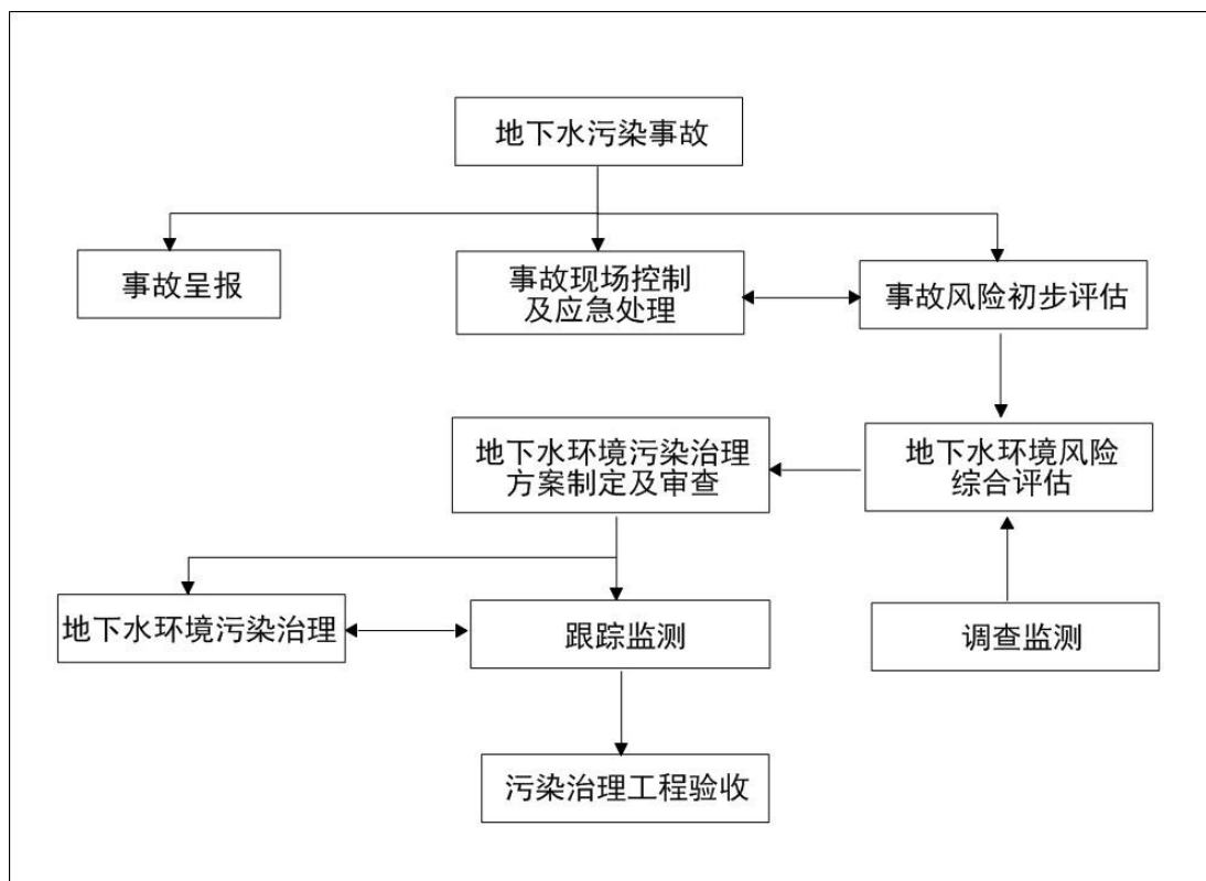
图 7.2-6 地下水污染事故应急处理程序图
