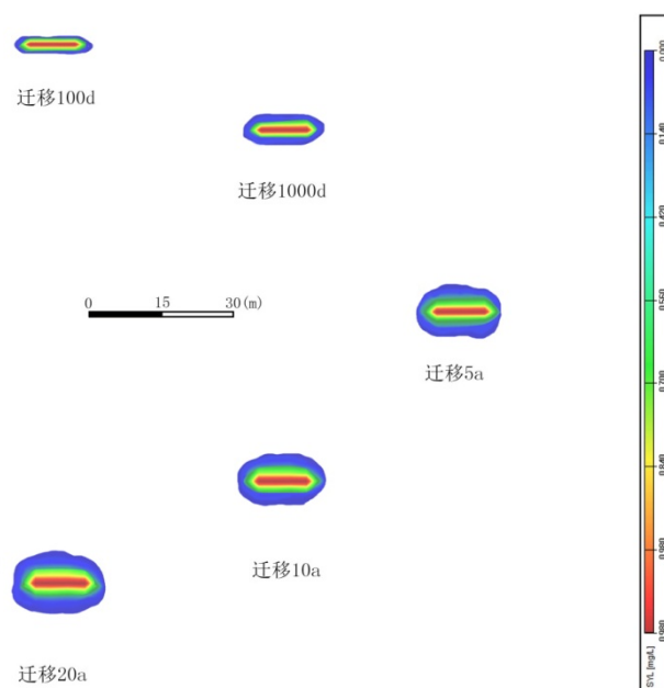
图 5.3-32 非正常情况下苯迁移平面图
