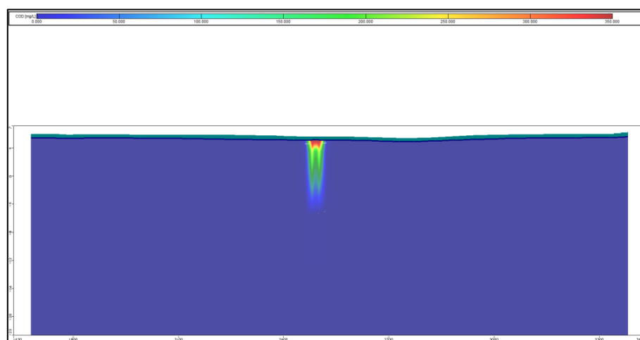
图 5.3-21 非正常情况下 a-a'剖面图 (COD 迁移 20a 扩散图)
