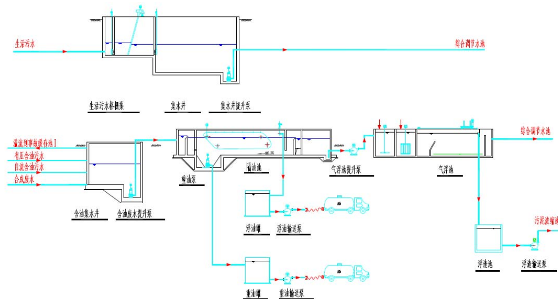
图 7.2-1 含油污水预处理工艺流程图
