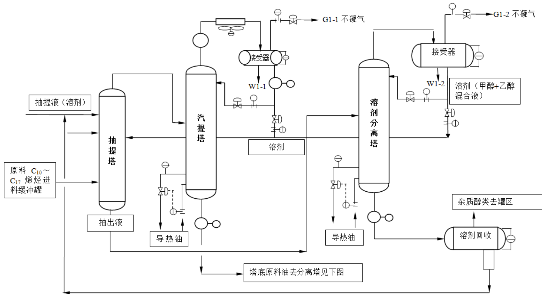
图 3.3-1 净化分离工艺流程及产污节点图 (一)
