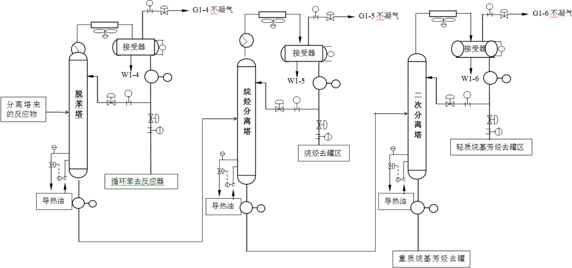
图 3.3-4 反应工序工艺流程及产污节点图（二）
