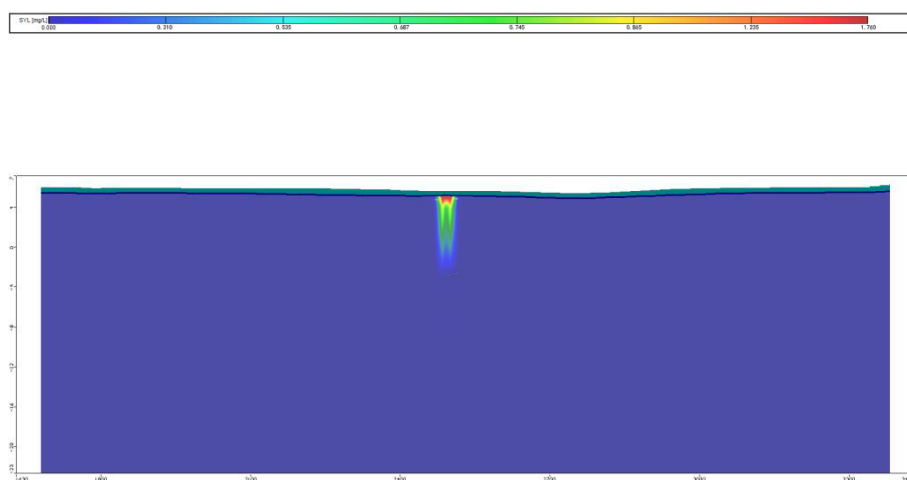
图 5.3-27 正常情况下 a-a'剖面图（氟化物迁移 20a 扩散图）
