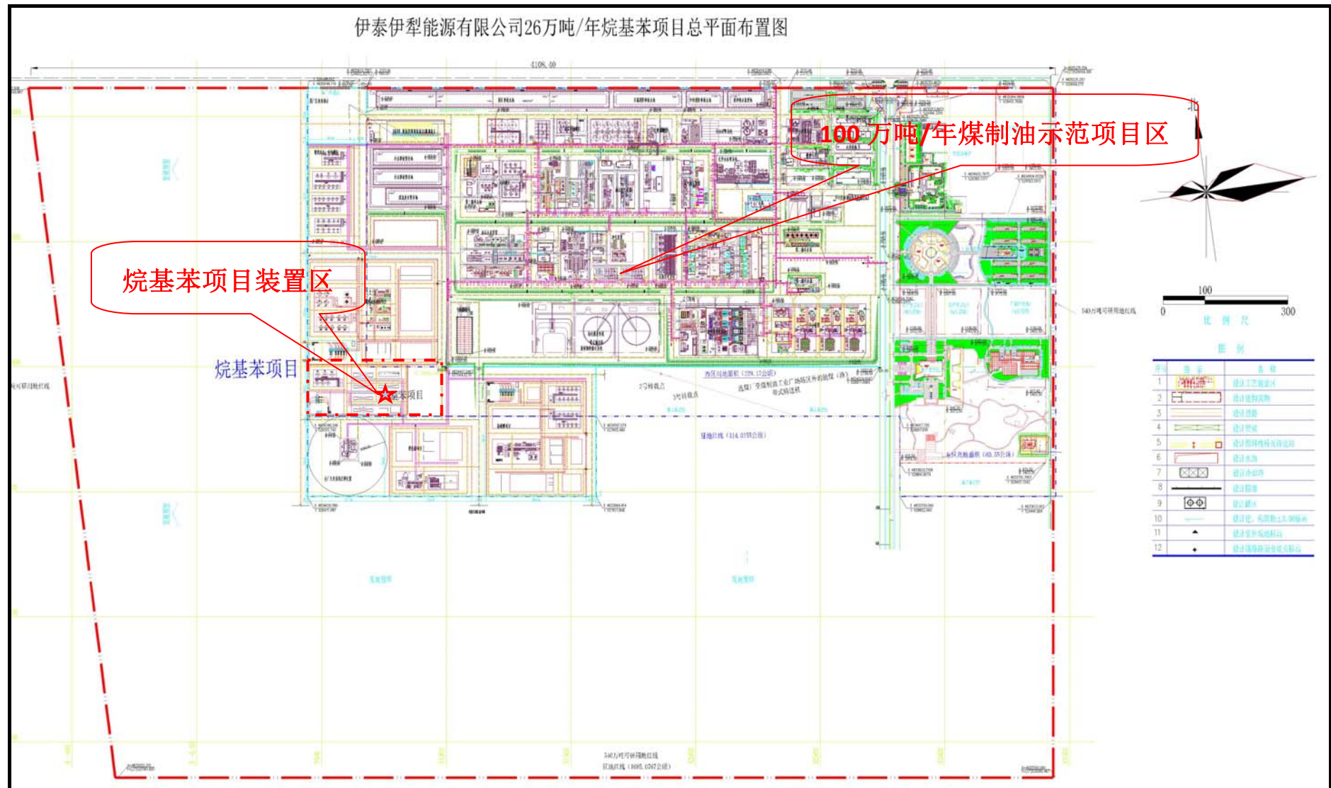
图 3.2-1 烷基苯项目总平面布置示意图
