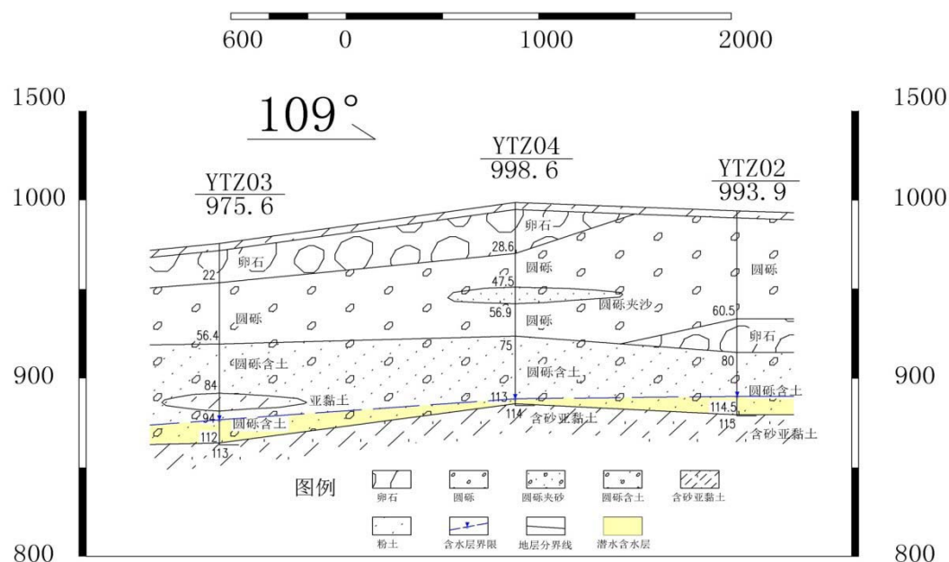
图 5.3-9 厂区 D-D 水文地质剖面图
