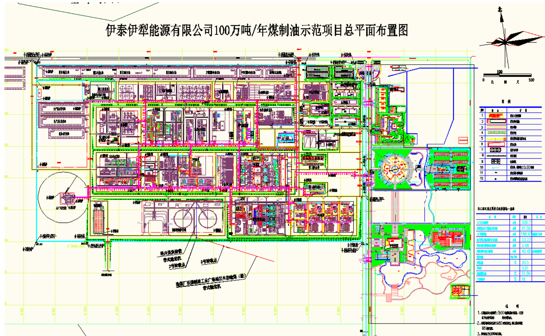
图 3.1-2 现有工程总平面布置示意图
