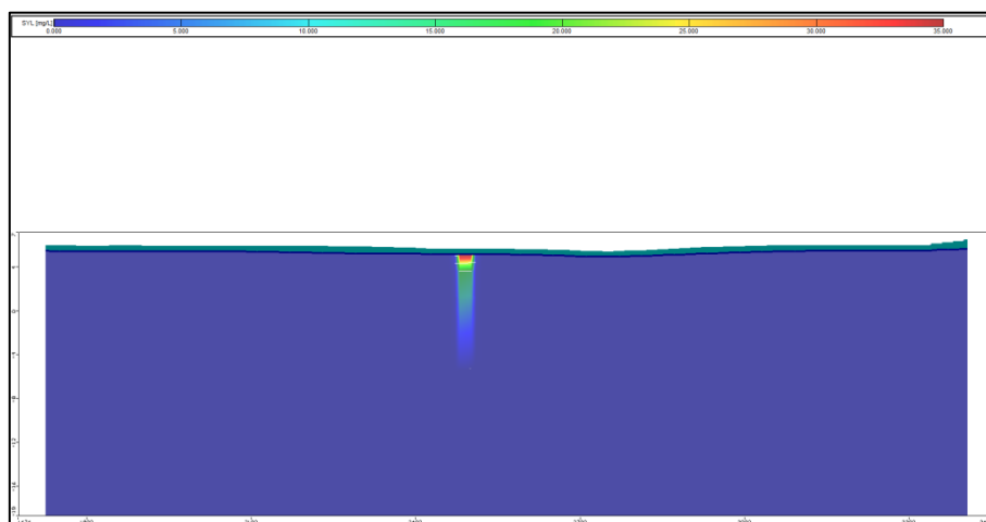
图 5.3-23 正常情况下 a-a'剖面图（氨氮迁移 20a 扩散图）
