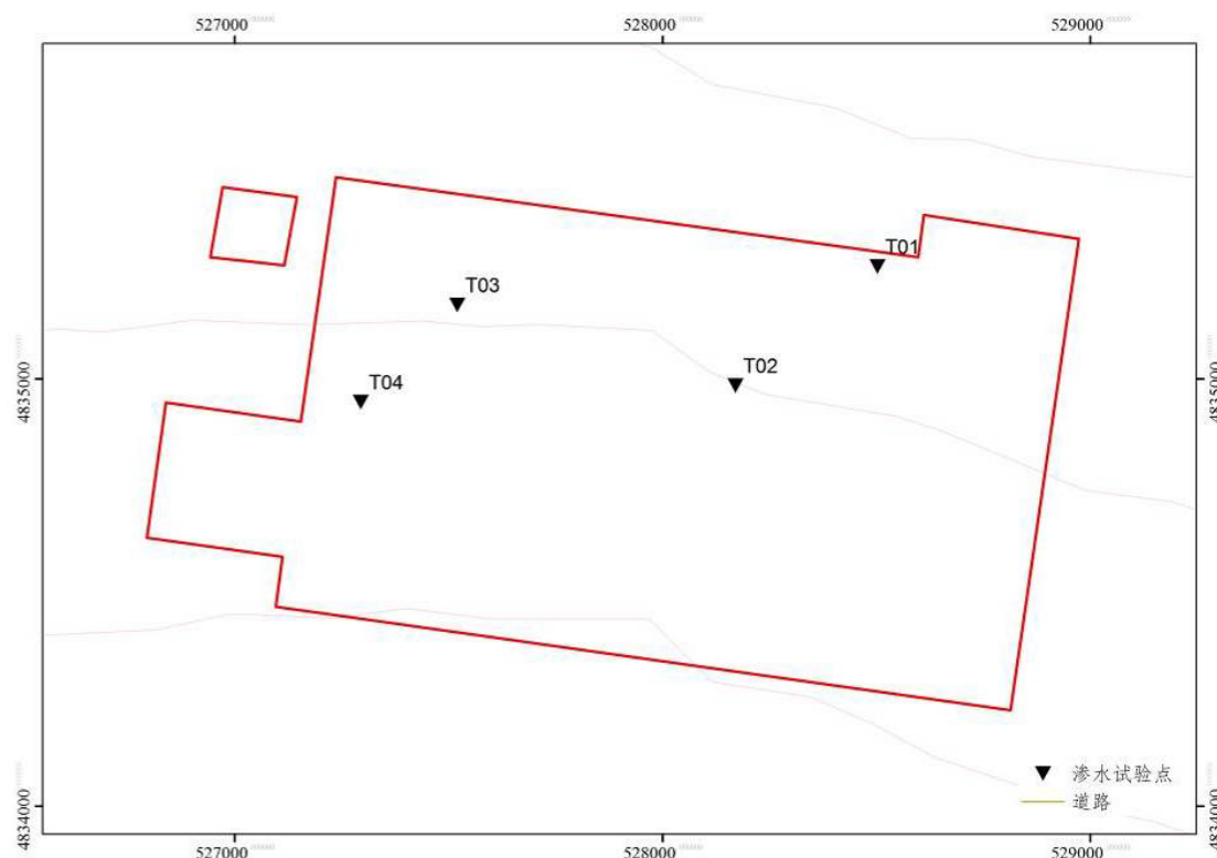
图 5.3-10 厂址区渗水试验点分布图
