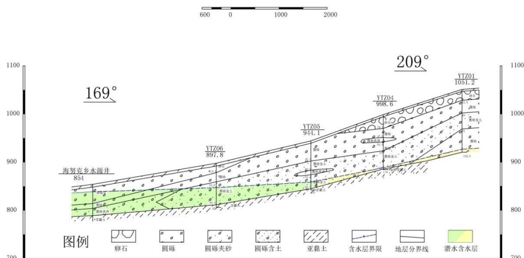
图 5.3-6 厂区 C-C 水文地质剖面图
