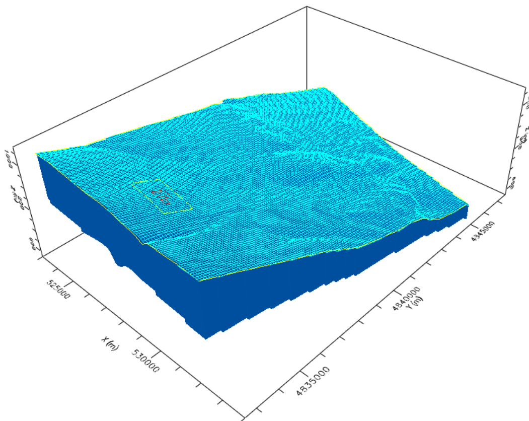
图 5.3-13 模型网格剖分示意图
