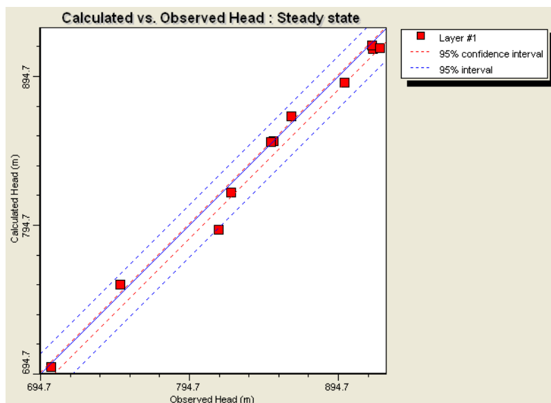
图 5.3-17 实测水位与模拟水位拟合效果图
