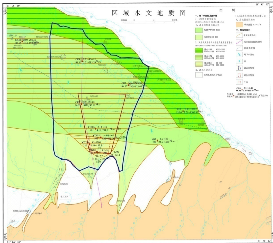
图 5.3-1 区域水文地质图
