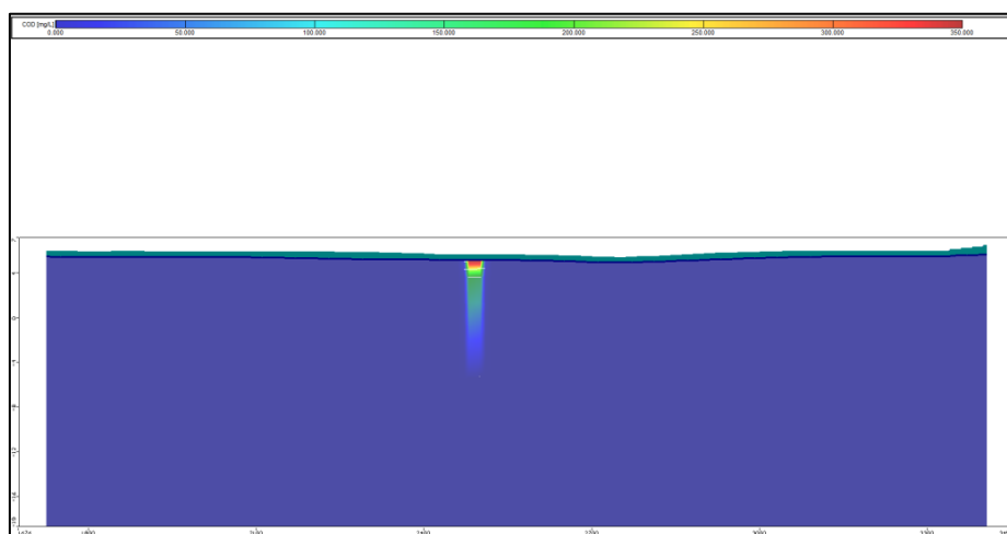
图 5.3-19 正常情况下 a-a'剖面图 (COD 迁移 20a 扩散图)
