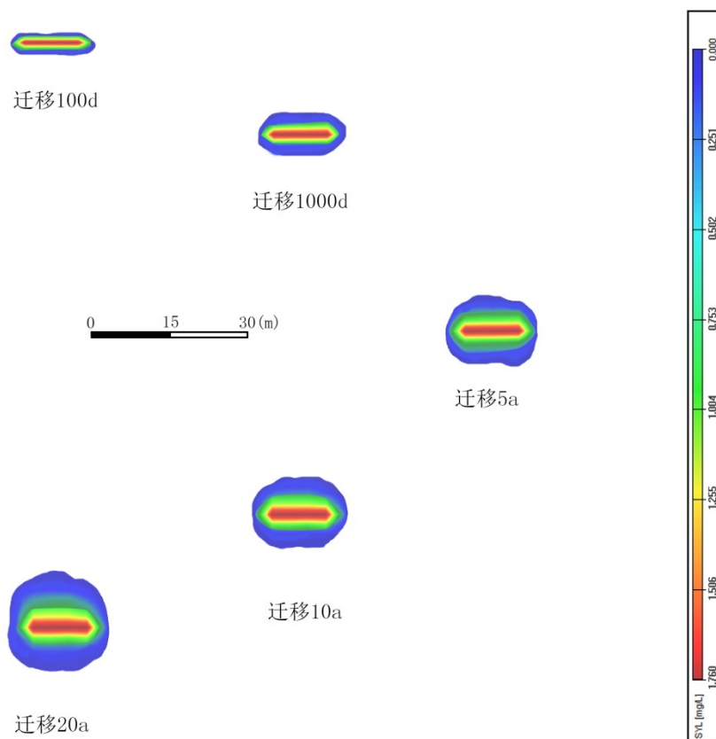
图 5.3-28 非正常情况下氟化物迁移平面图
