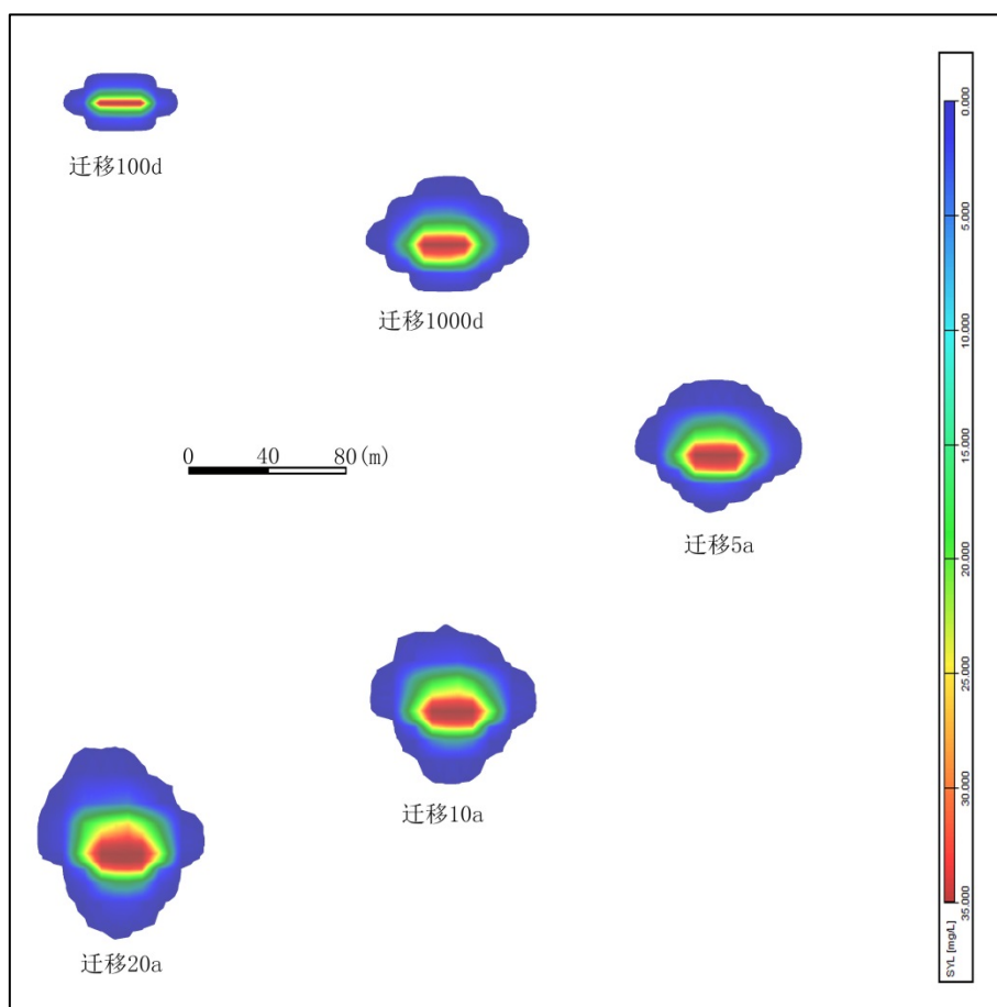
图 5.3-24 非正常情况下氨氮迁移平面图
