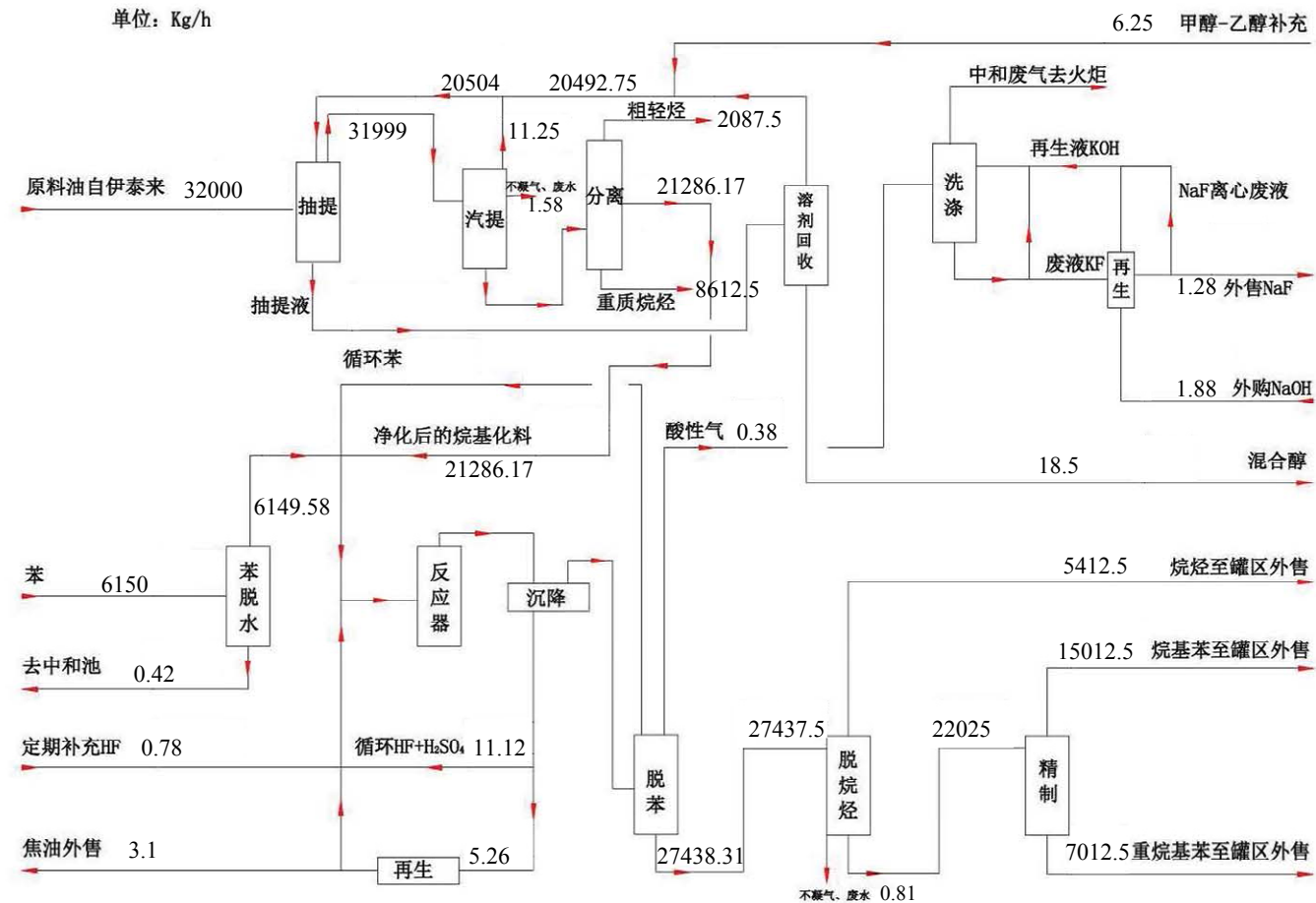
图 3.3-6 烷基苯项目物料平衡示意图
