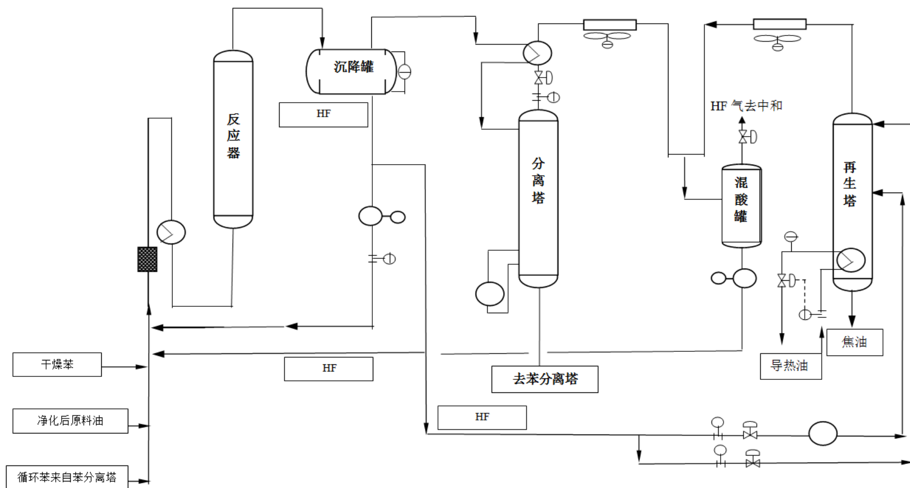
图 3.3-3 反应工序工艺流程及产污节点图（一）
