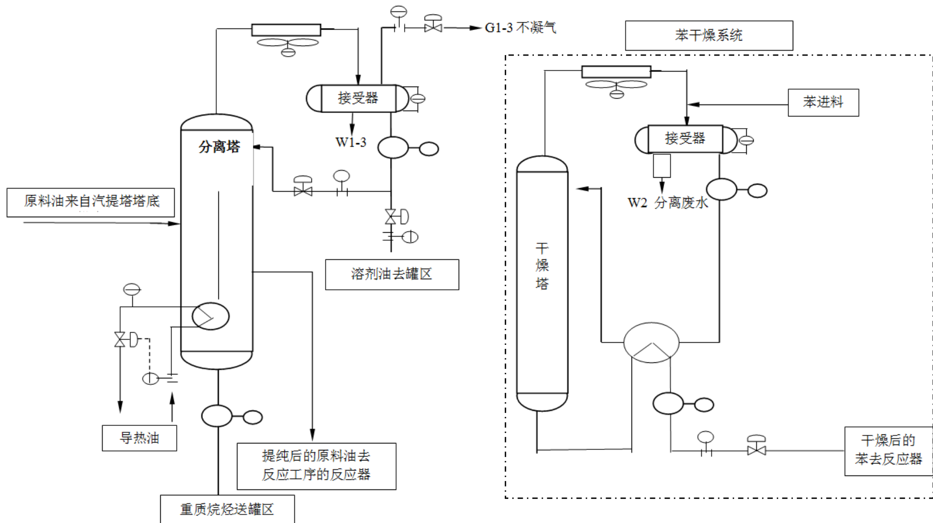
图 3.3-2 净化分离工艺流程图（二）、苯干燥工艺流程图及排污节点图
