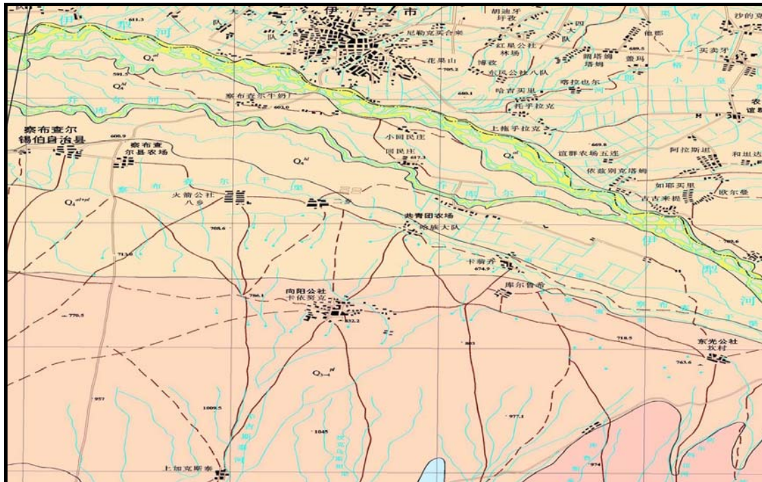
图 4.1-2 厂址工程地质构造图
