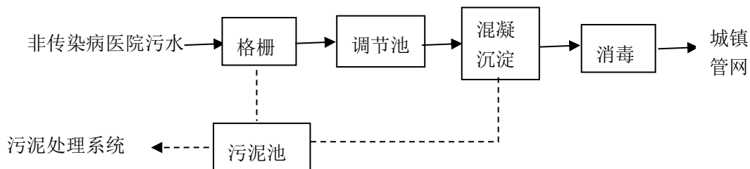
图 6.2-2 非传染病医院污水一级强化处理工艺流程
