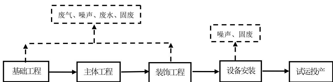
图 3.3-1 污水处理站工艺流程及产污环节图
