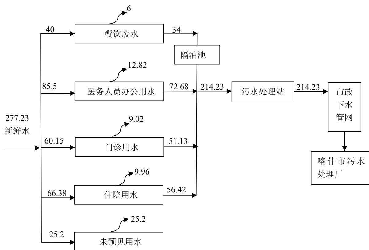
图 3.3-3 水平衡图 (单位 \text{m}^3/\text{d} )
