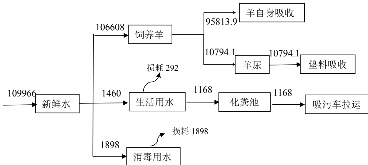
图 3.4-1 本项目水平衡示意图 (单位: \text{m}^3/\text{a} )
