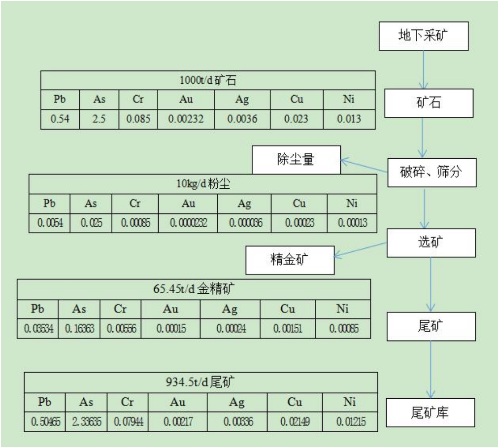
图 3.5-3 本项目重金属平衡图
