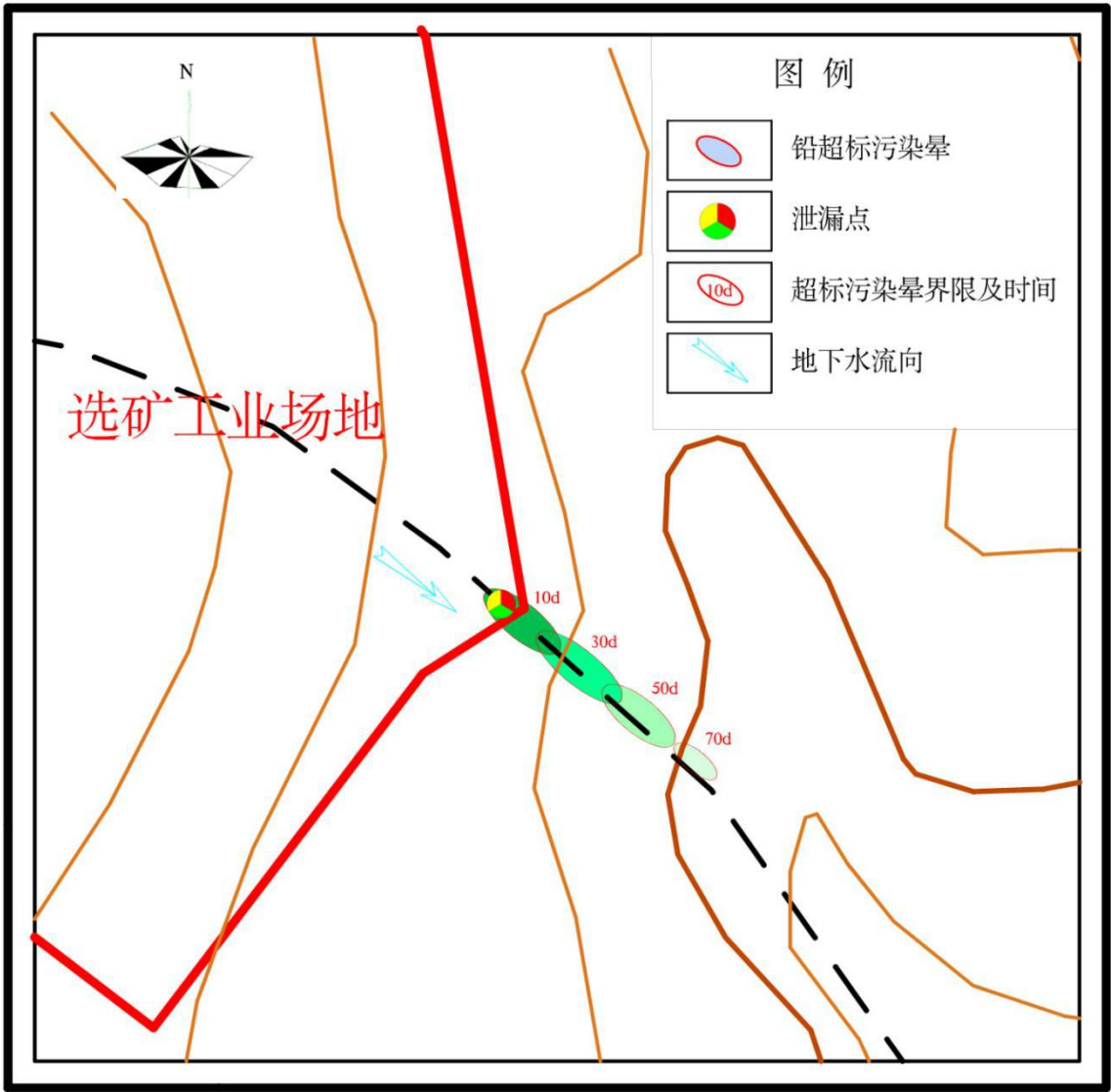
图 5. 2. 3-7 瞬时泄漏 Pb 污染晕示意图
