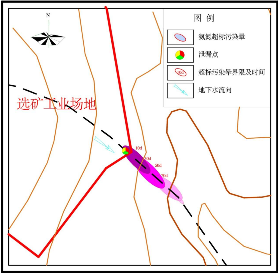
图 5. 2. 3-5 瞬时泄漏 \text{NH}_3\text{-N} 污染晕示意图
