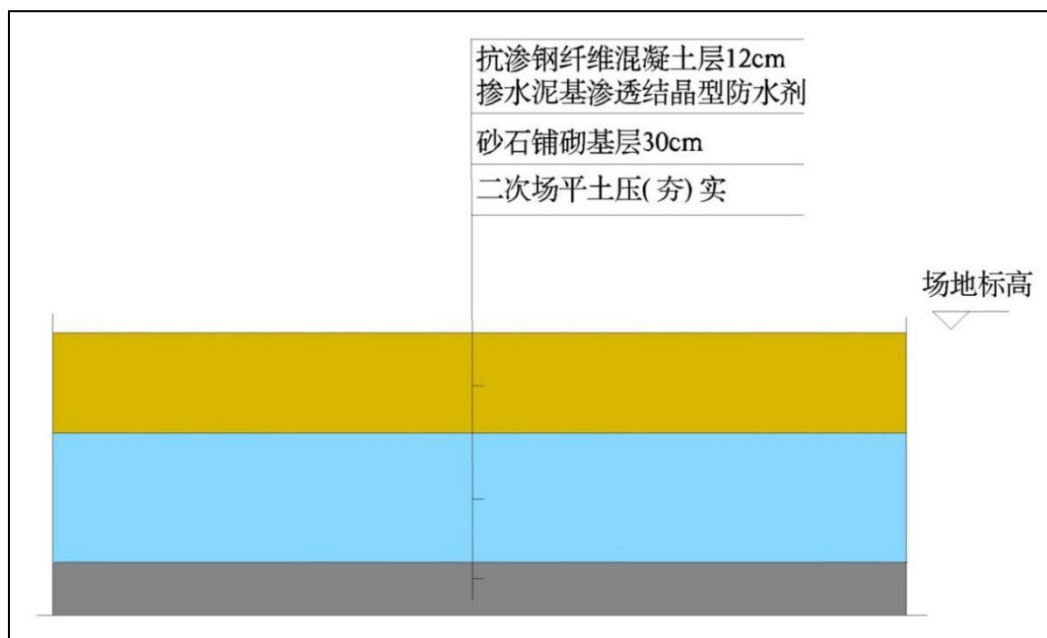
图 7.2.3-4 一般防渗区结构示意图
