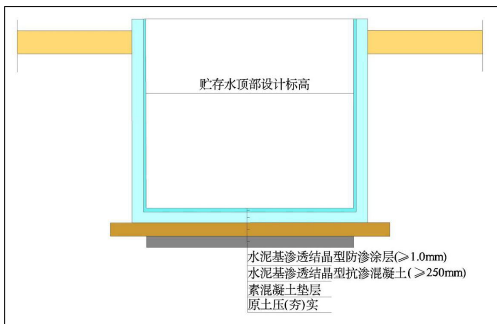
图 7.2.3-2 污水池防渗结构示意图
