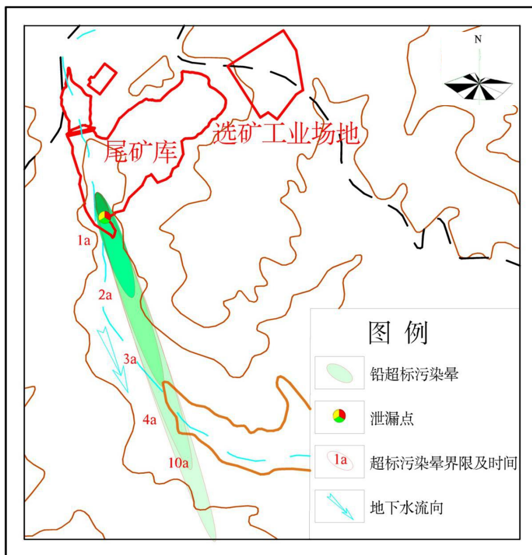
图 5.2.3-13 持续泄漏 Pb 污染晕分布示意图
