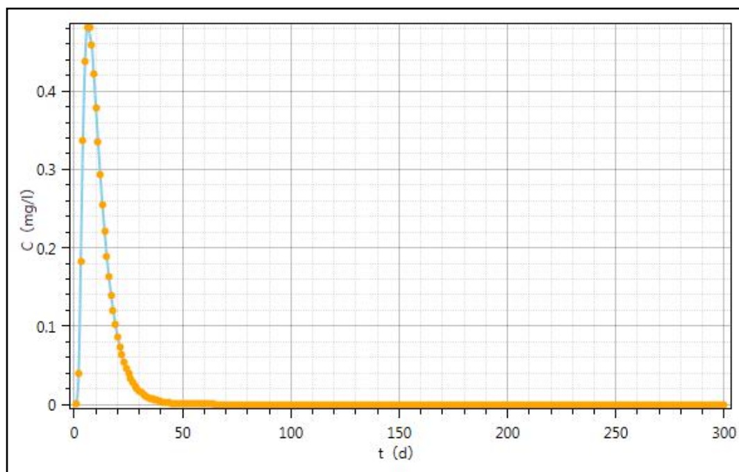
图 5.2.3-8 下游 10m 处含水层中 Pb 浓度变化趋势图
