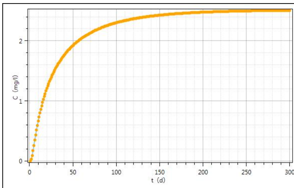
图 5.2.3-12 下游 10m 处含水层中氨氮浓度变化趋势图
