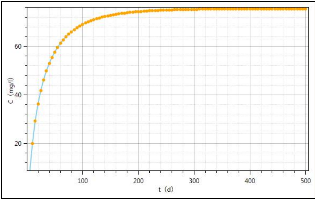
图 5.2.3-10 下游 10m 处含水层中 COD 浓度变化趋势图
