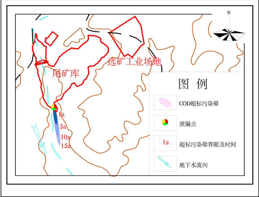
图 5.2.3-9 持续泄漏 COD 污染晕分布示意图
