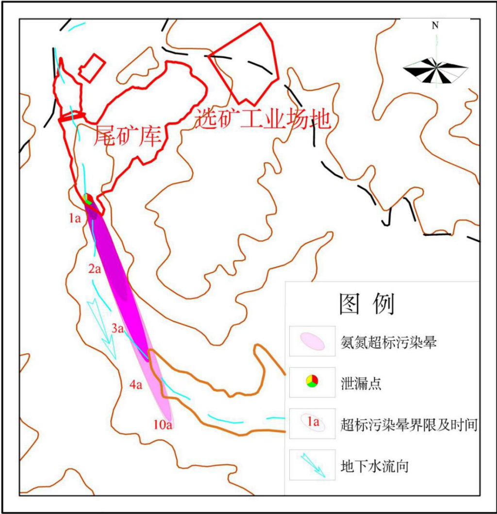
图 5.2.3-11 持续泄漏氨氮污染晕分布示意图
