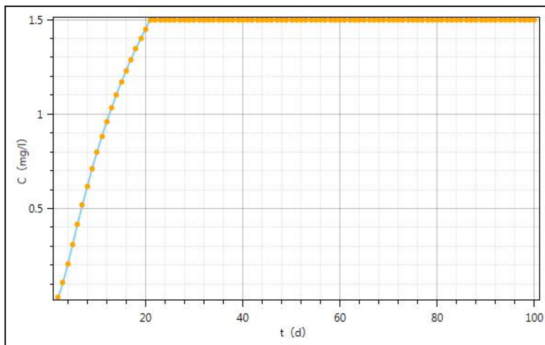
图 5.2.3-14 下游 10m 处含水层中 Pb 浓度变化趋势图
