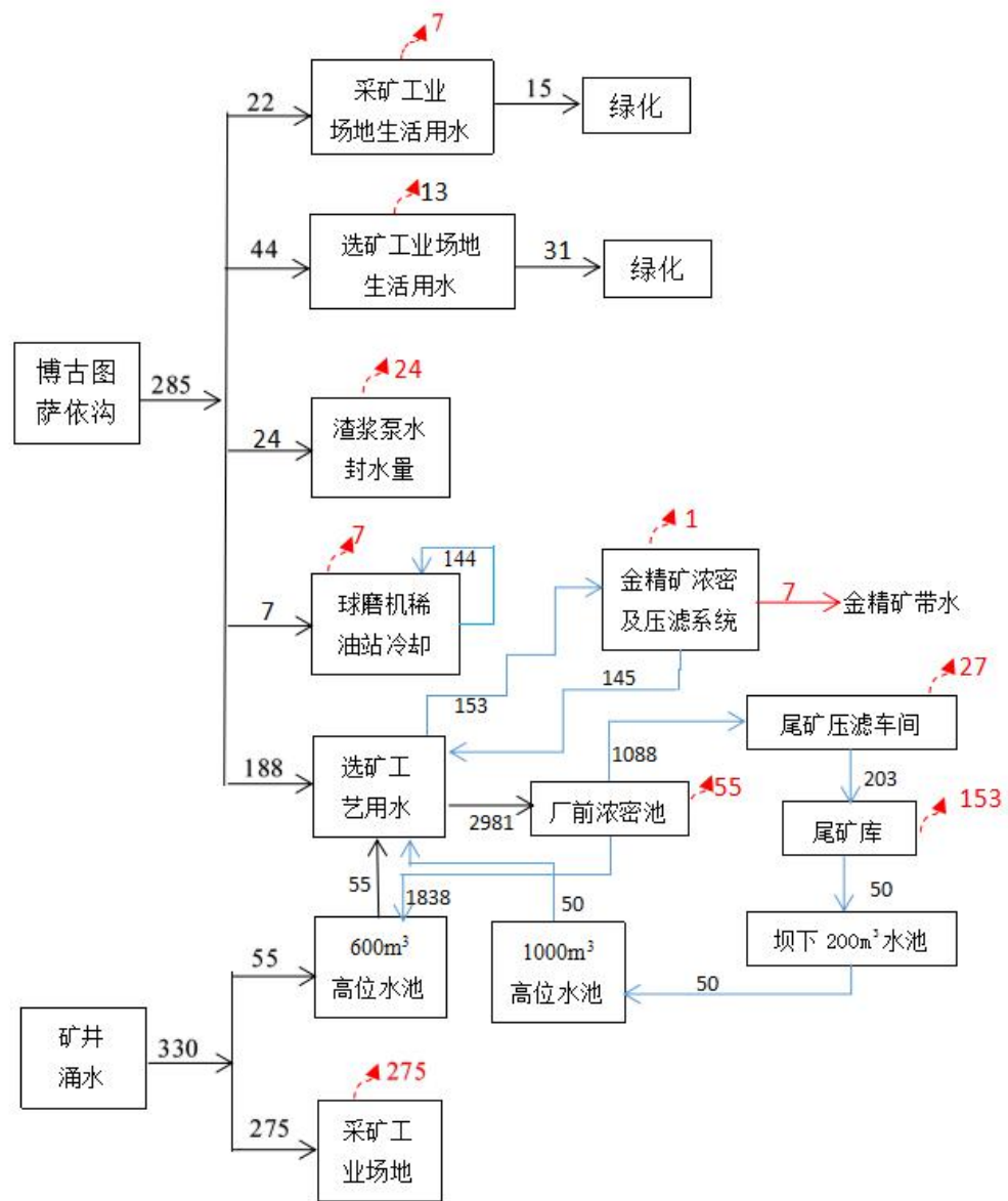
图 3.5-2 本项目水平衡图（单位： \text{m}^3/\text{d} ）
