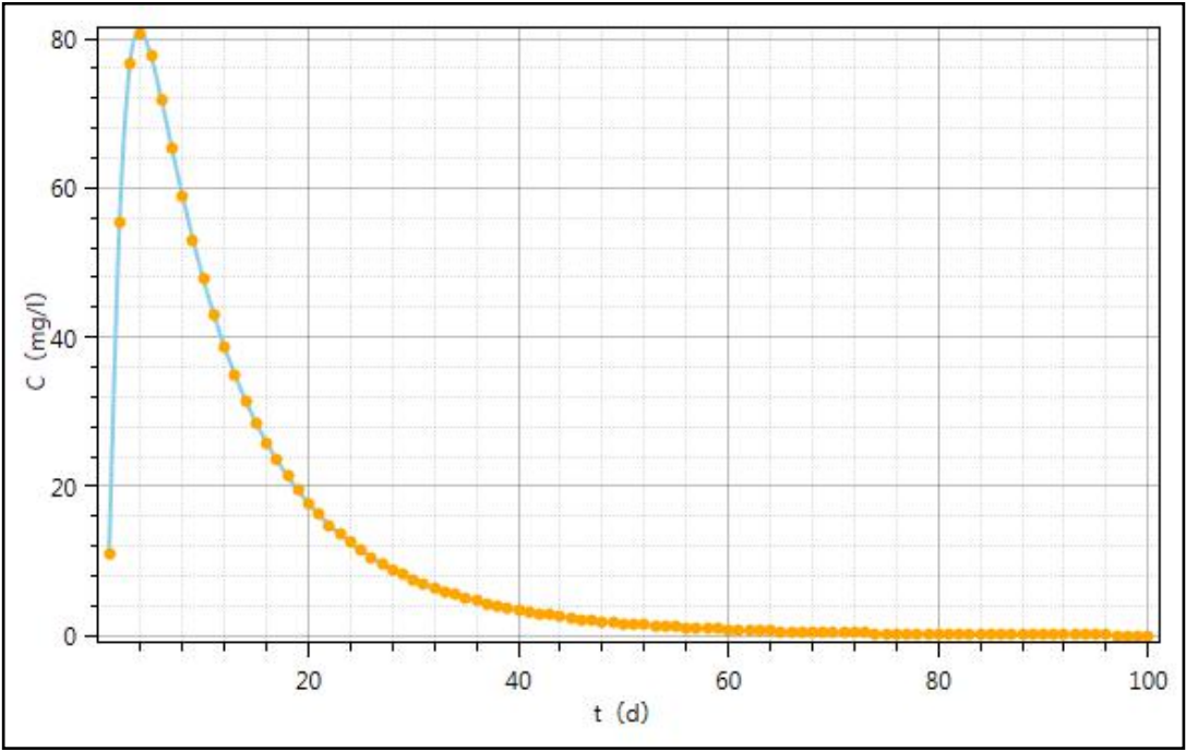
图 5.2.3-4 下游 10m 处含水层中 COD 浓度变化趋势图
