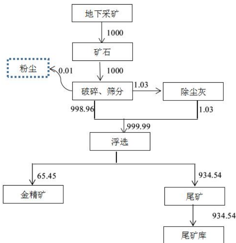
图 3.5-1 本项目物料平衡图
