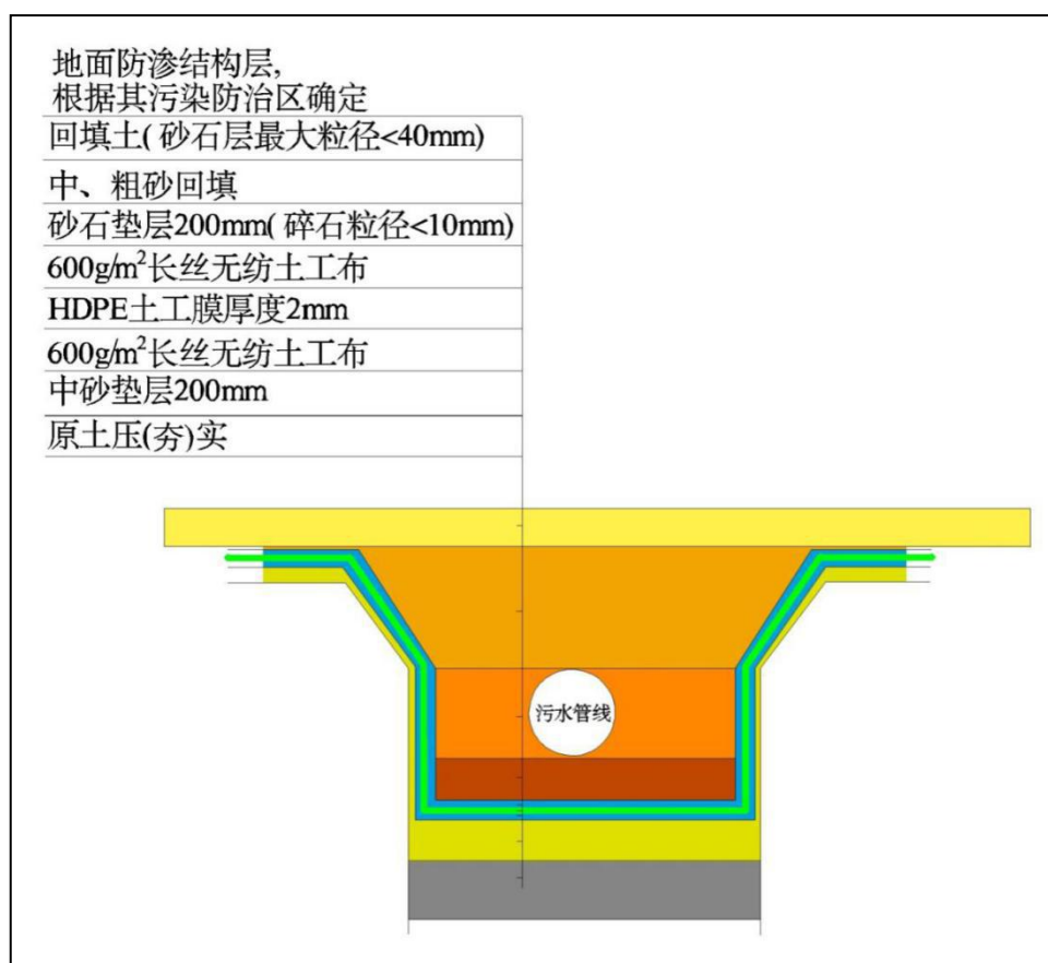
图 7.2.3-3 埋地管道防渗结构示意图
