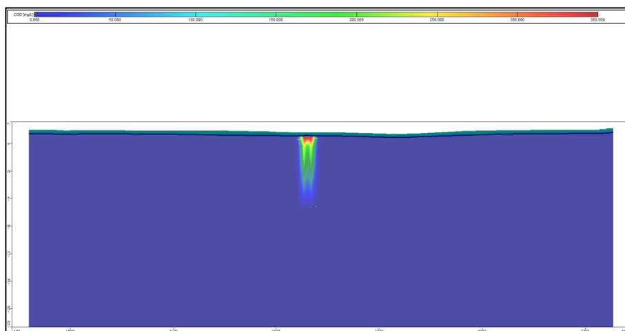
图 6.3-21 非正常情况下 a-a'剖面图 (COD 迁移 20a 扩散图)
