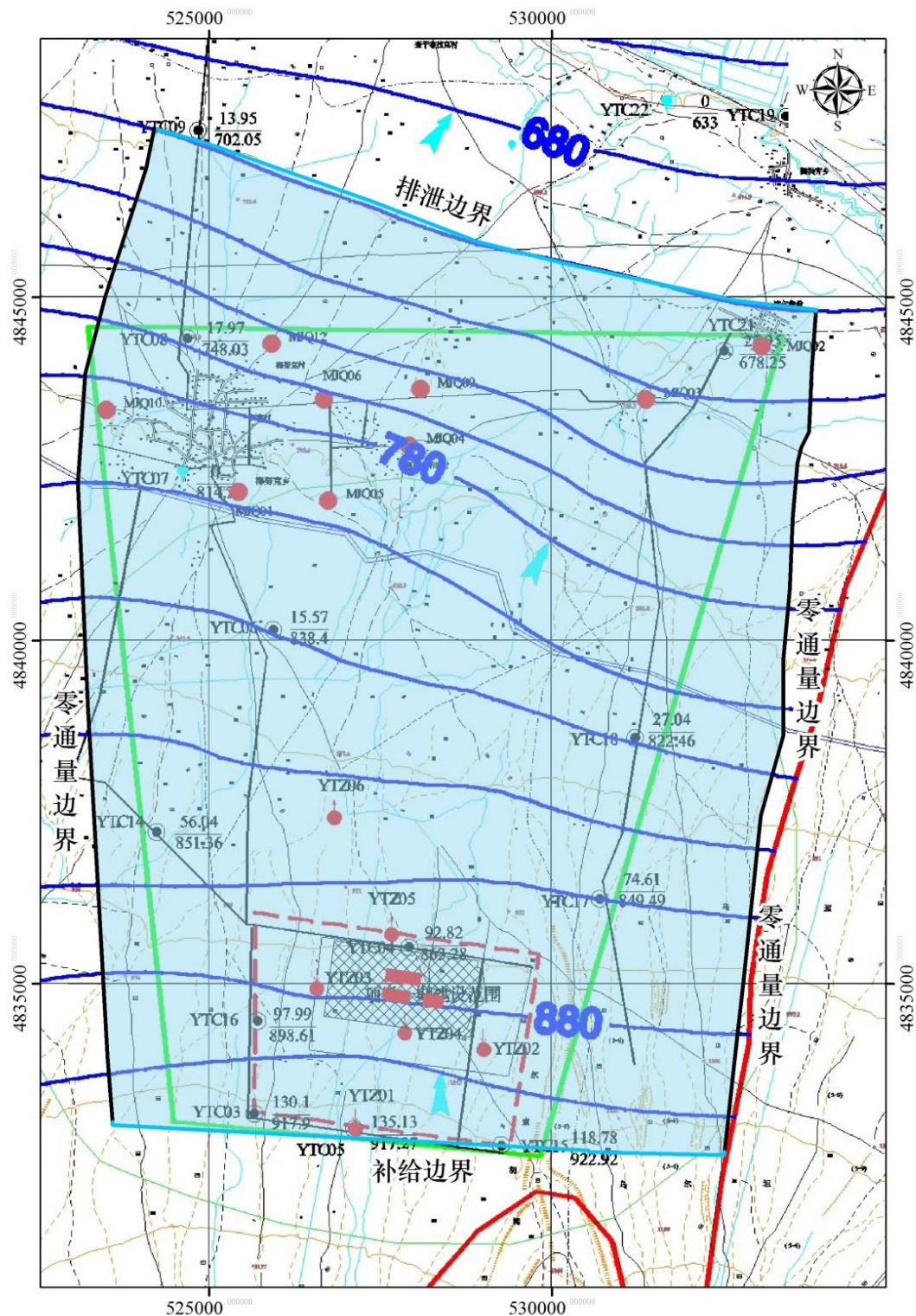
图 6.3-11 地下水模型范围及边界（图中黑色和浅蓝色线条包围区域）
