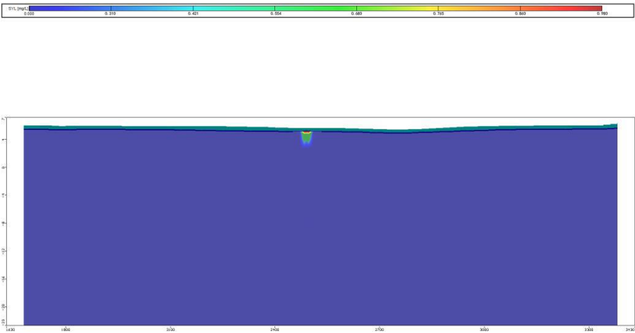
图 6.3-27 正常情况下 a-a'剖面图（苯迁移 20a 扩散图）
