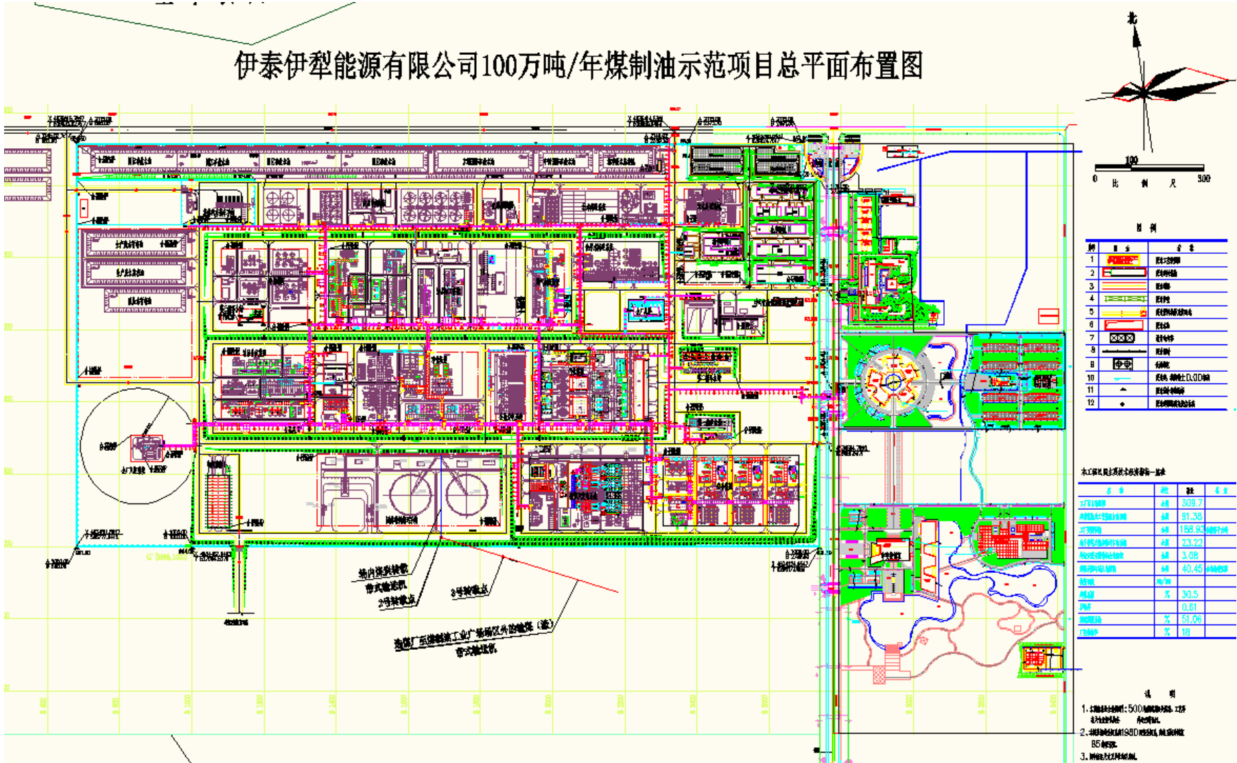
图 3.2-2 现有工程总平面布置示意图
