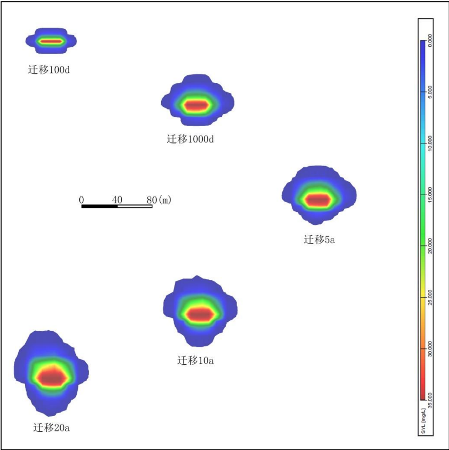
图 6.3-24 非正常情况下氮氮迁移平面图
