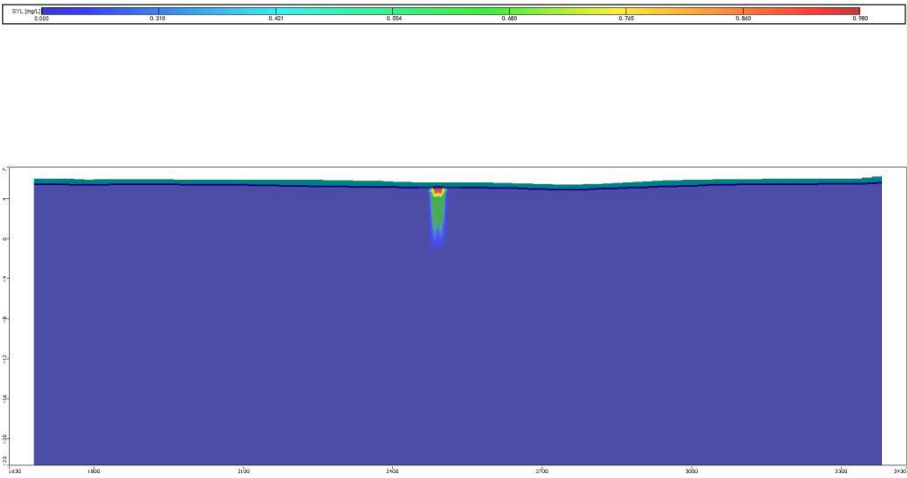
图 6.3-29 非正常情况下 a-a'剖面图（苯迁移 20a 扩散图）
