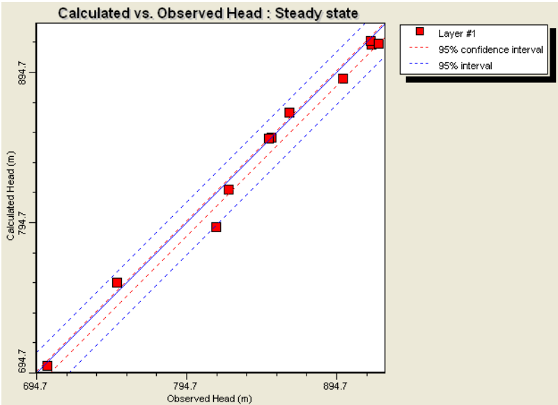
图 6.3-17 实测水位与模拟水位拟合效果图
