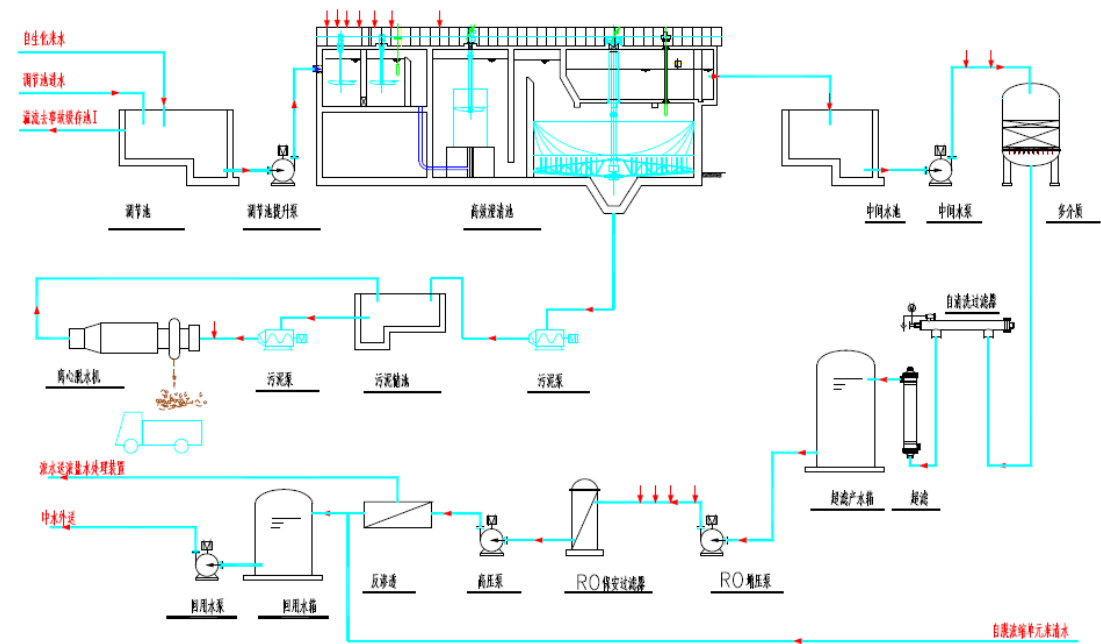
图 7.2-3 废水回用处理装置工艺流程图
