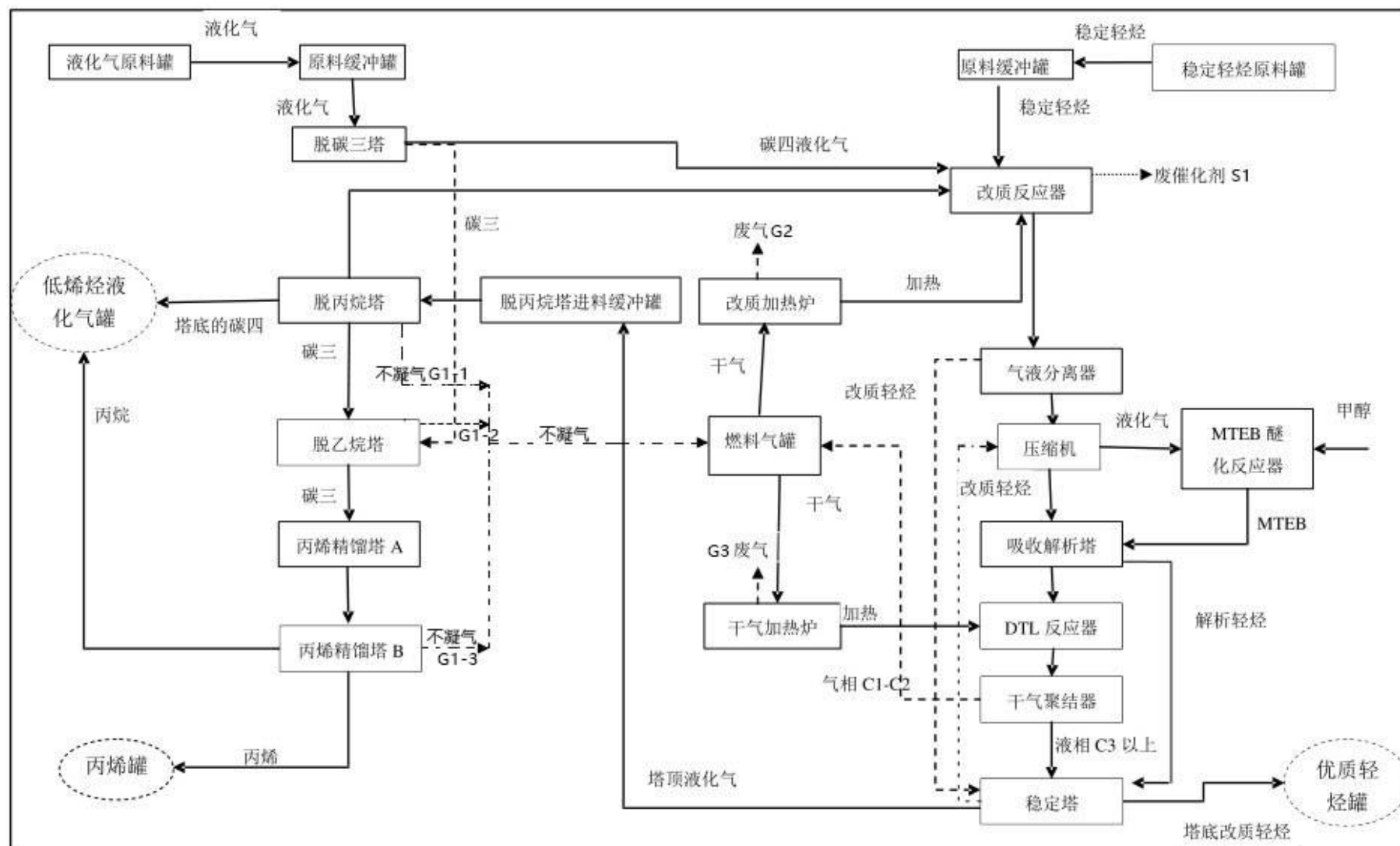
图 4.2-1 工艺流程及产污节点图
