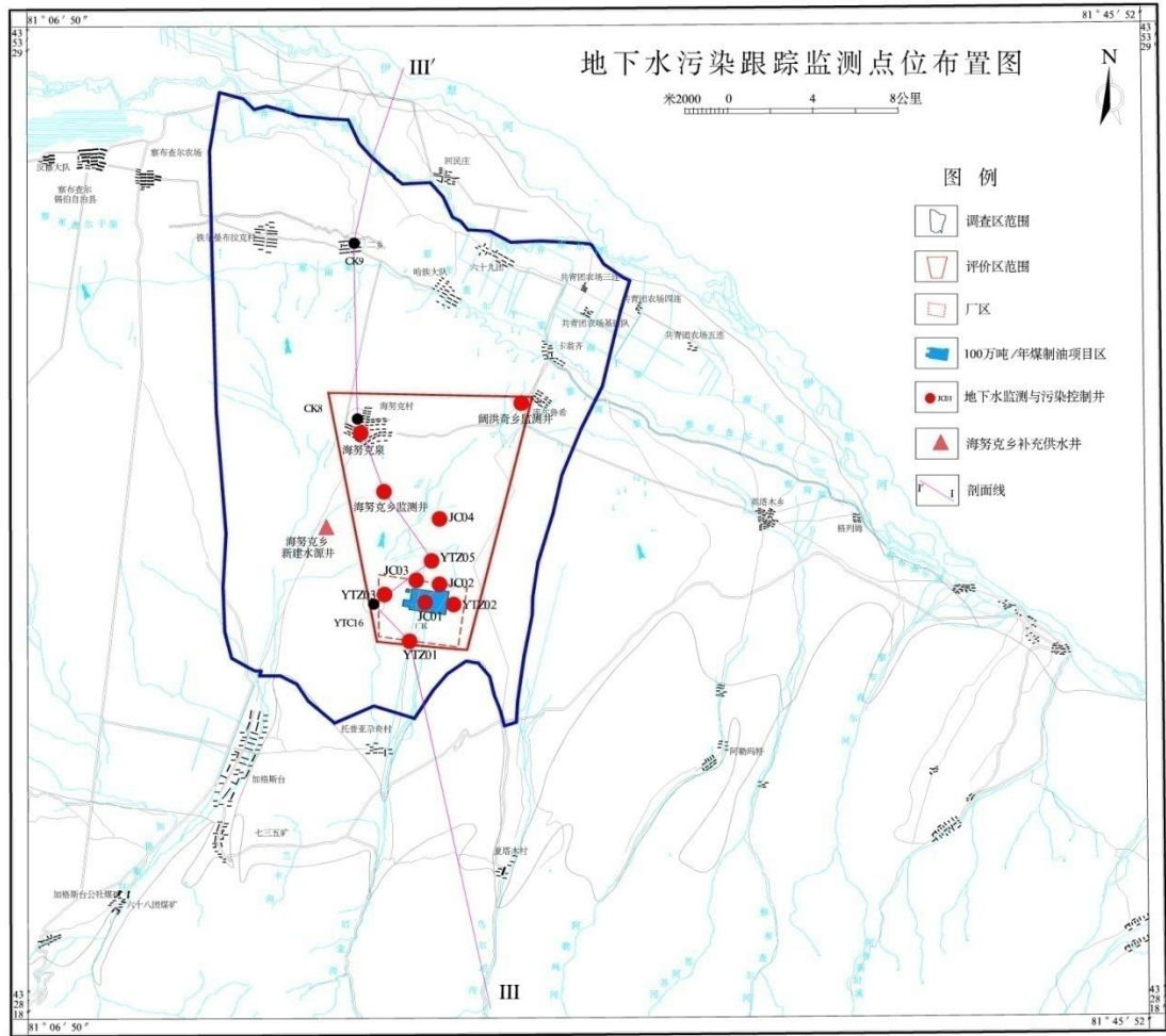
图 7.2-2 地下水跟踪监测井布置示意图
