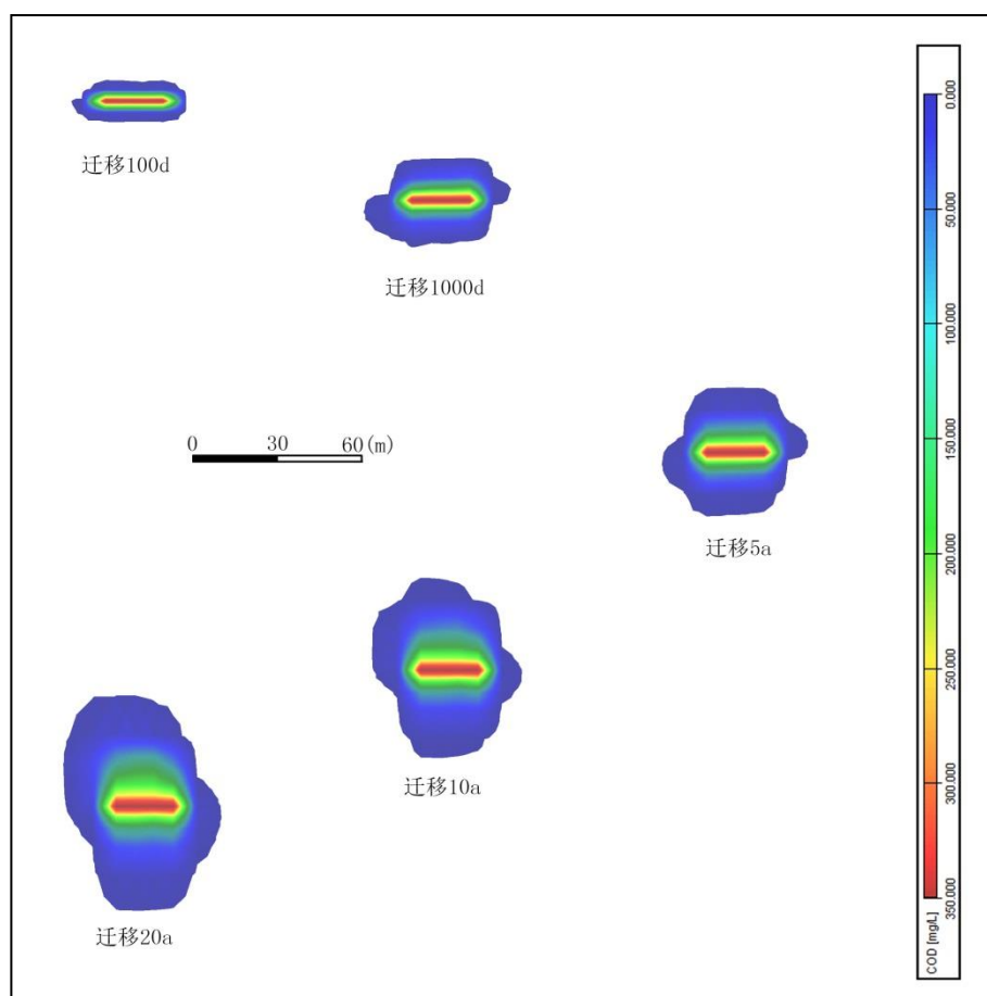
图 6.3-18 正常情况下 COD 迁移平面图
