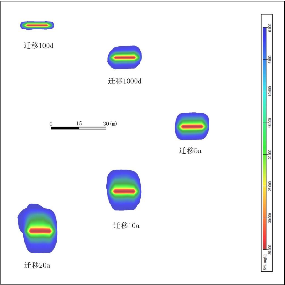
图 6.3-22 正常情况下氨氮迁移平面图
