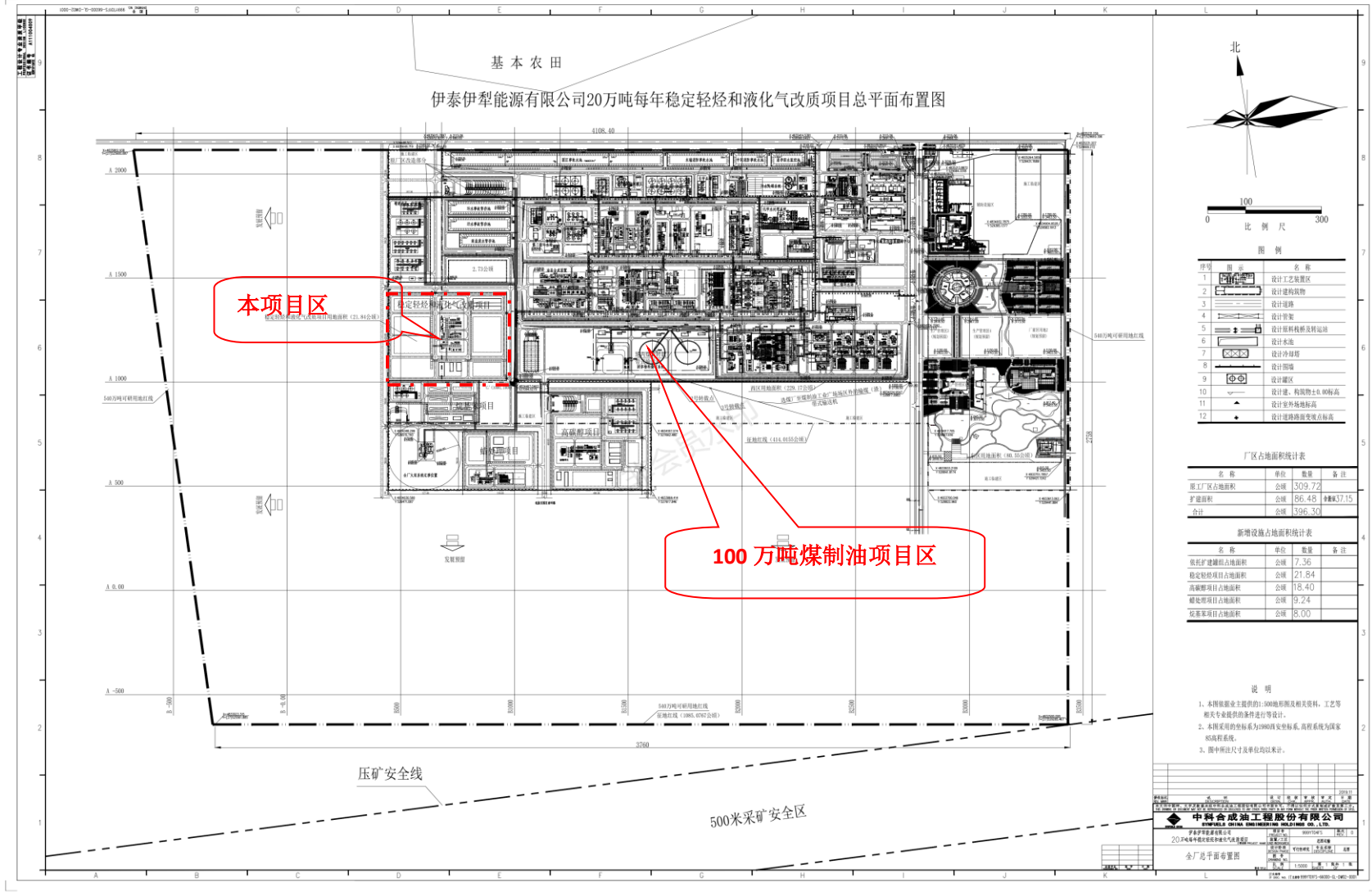
图3.5-1 稳定轻烃和液化气改质项目总平面布置示意图
