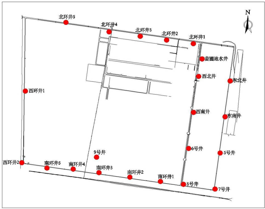
图 6.3-7 伊泰绿化供水井井位示意图
