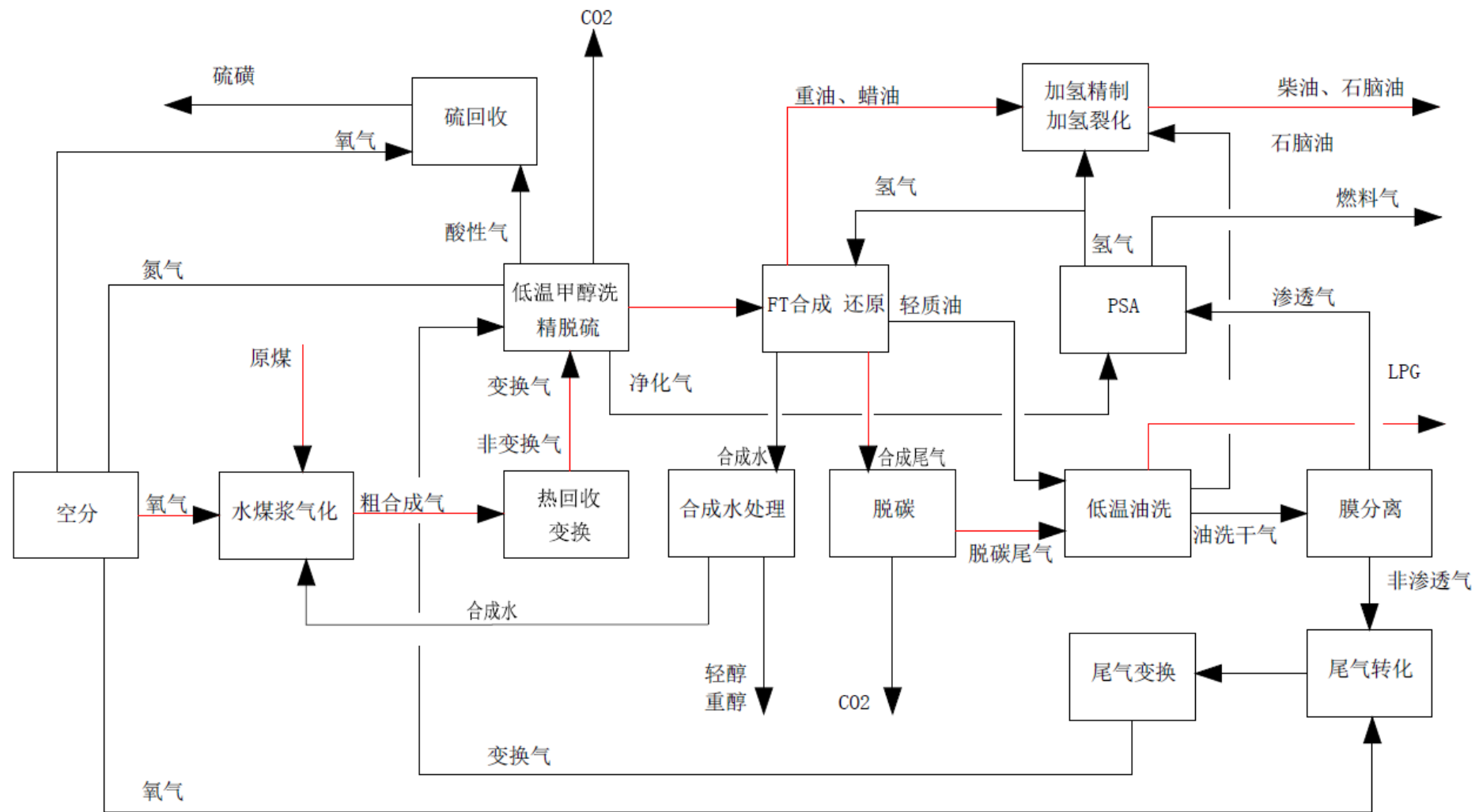
图 3.2-1 现有工程总加工工艺流程示意图
