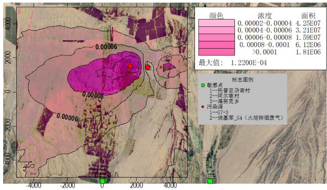
图 6.1-14 HF 日保证率叠加分布图
