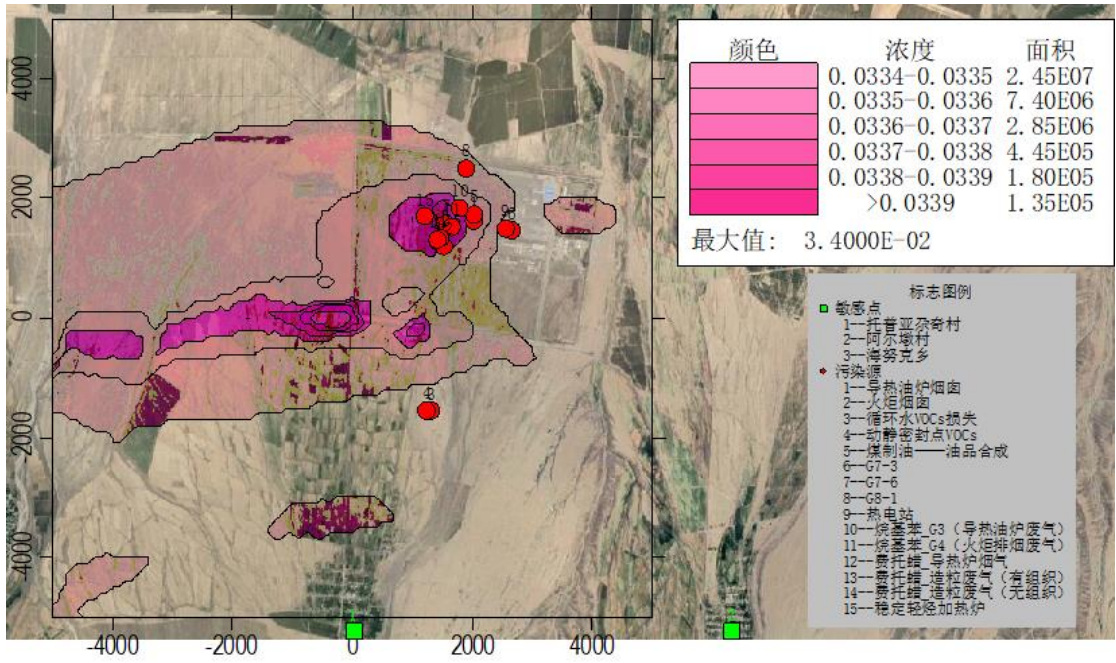
图 6.1-18 NO 2 年均落地浓度分布图 (mg/m 3 )
