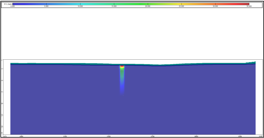
图 6.3-23 正常情况下 a-a'剖面图（氨氮迁移 20a 扩散图）
