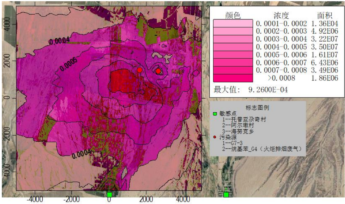
图 6.1-7 HF 最大小时落地浓度分布图
