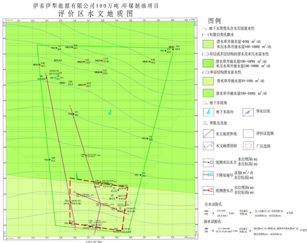
图 6.3-5 评价区水文地质图
