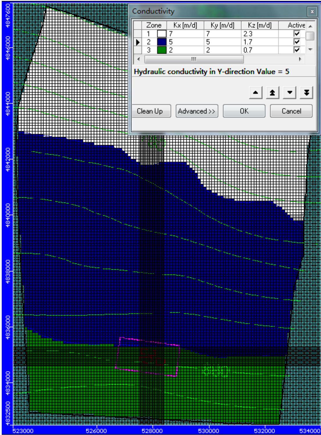
图 6.3-14 模型中初始渗透系数分区图
