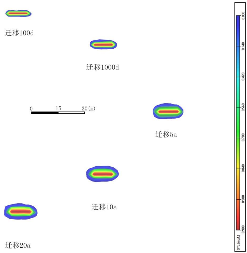
图 6.3-26 正常情况下苯迁移平面图
