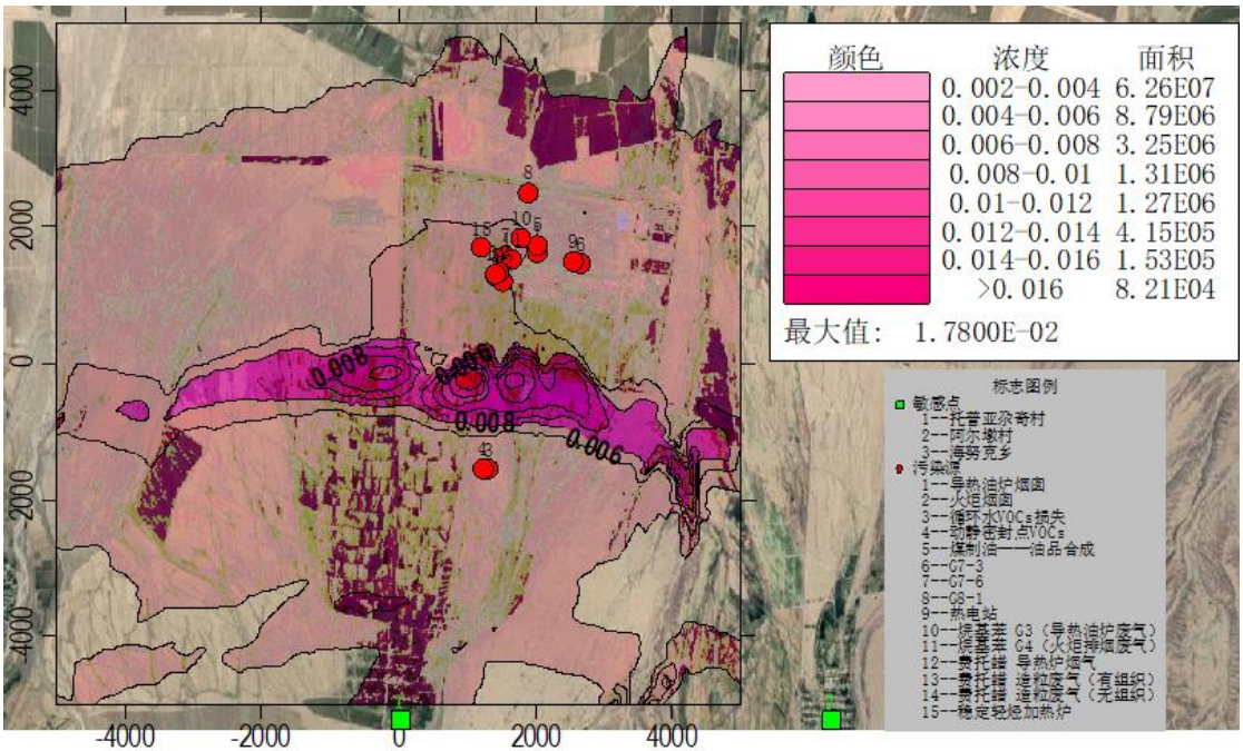
图 6.1-6 NO x 最大小时落地浓度分布图
