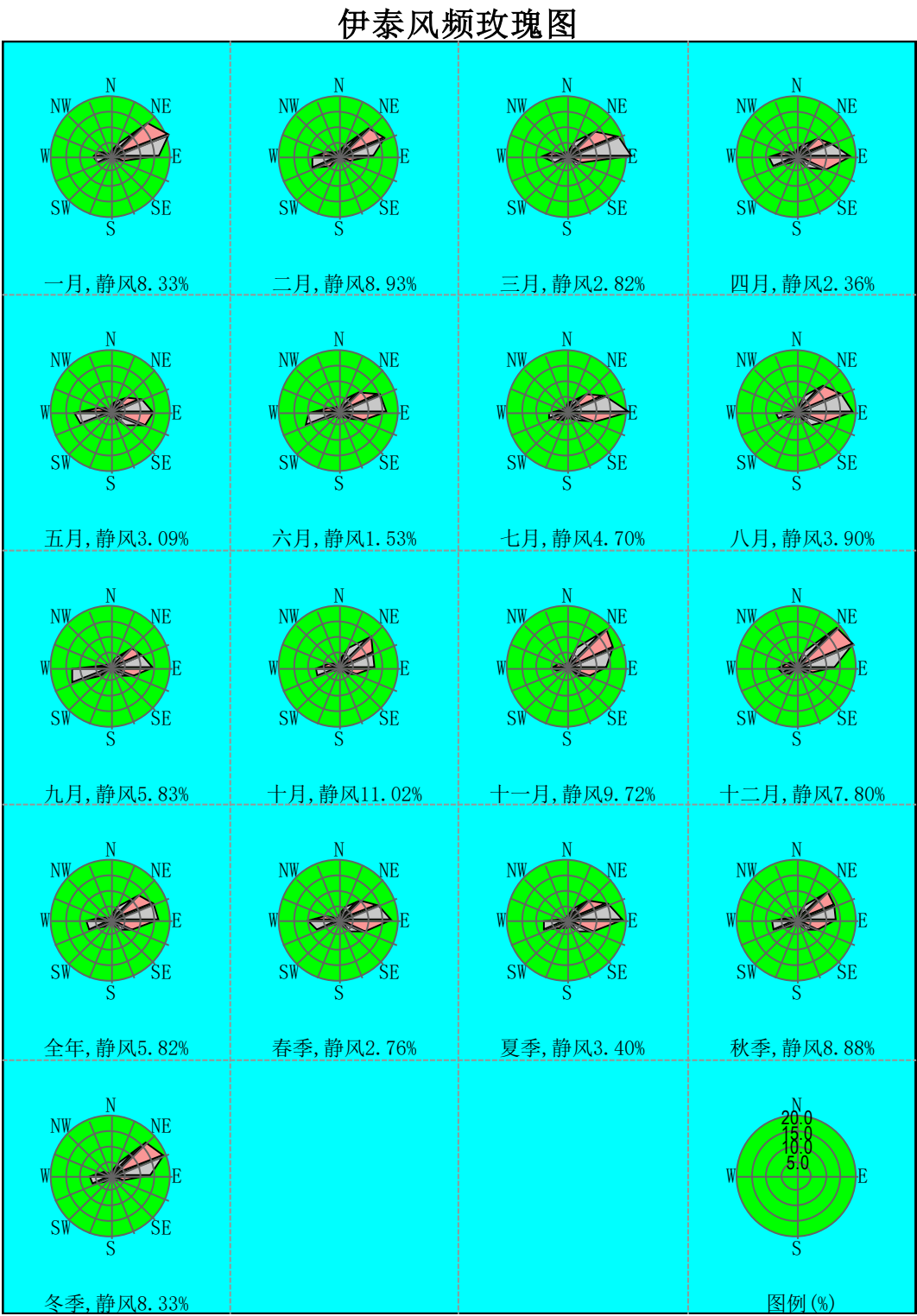
图 6.1-3 伊宁市 2018 年风频玫瑰图
