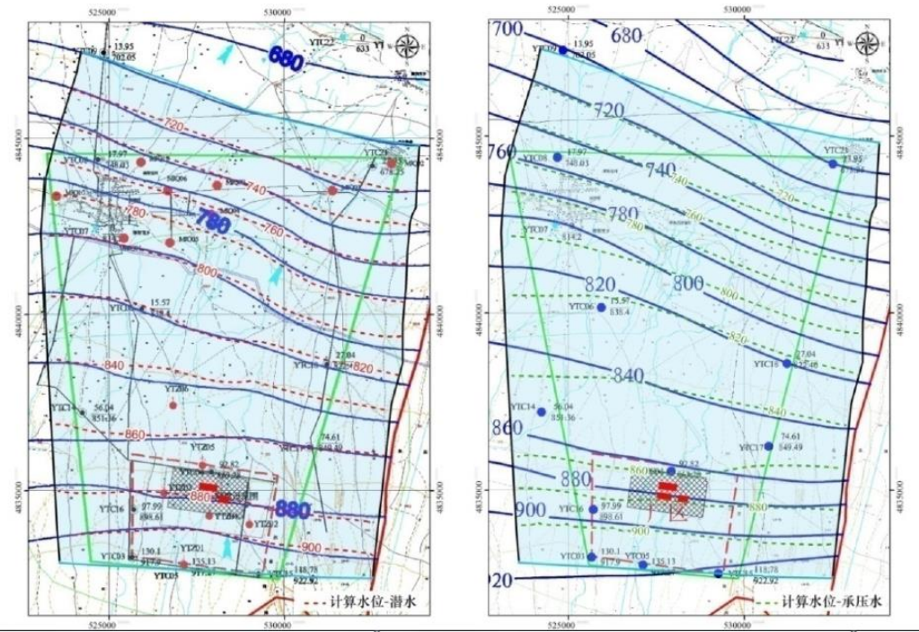
图 6.3-16 模拟等水位线与实测等水位线对比图（左潜水层、右承压水层）
