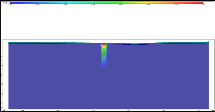
图 6.3-25 正常情况下 a-a'剖面图（氮氮迁移 20a 扩散图）
