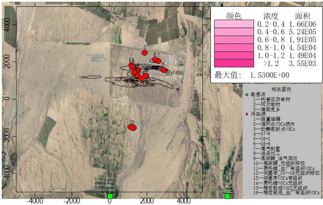
图 6.1-7 VOCs 最大小时落地浓度分布图
