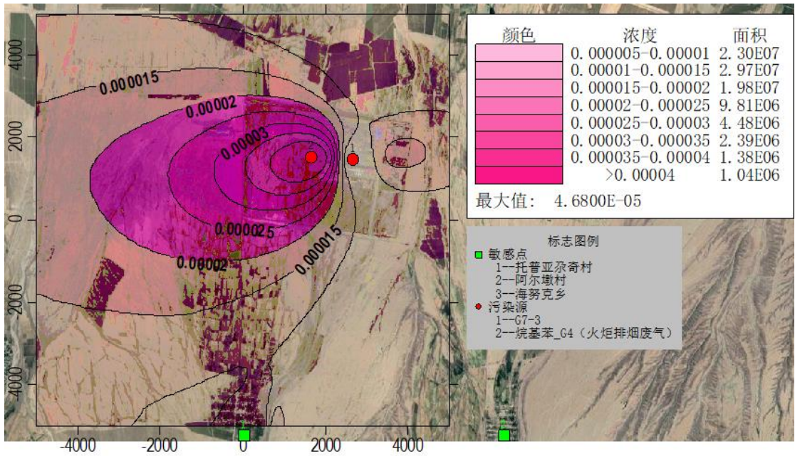
图 6.1-19 HF 年均落地浓度分布图 (mg/m 3 )
