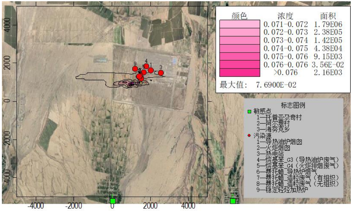
图 6.1-16 PM 10 年均落地浓度分布图 (mg/m 3 )
