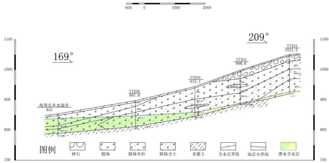
图 6.3-6 厂区 C-C 水文地质剖面图
