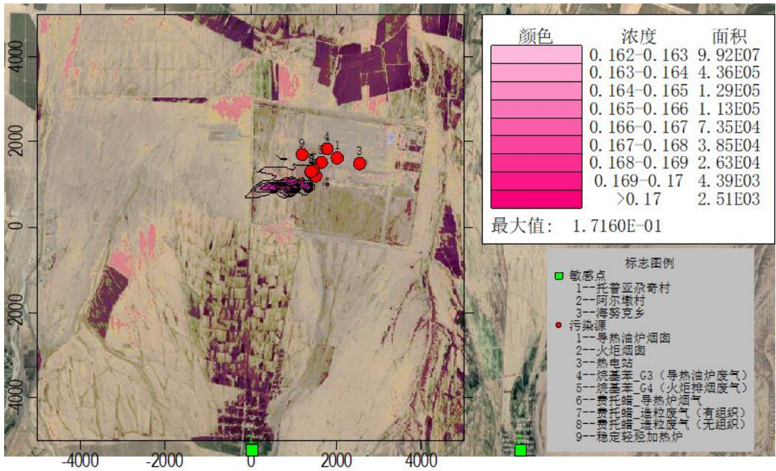
图 6.1-10 PM 10 日保证率叠加分布图
