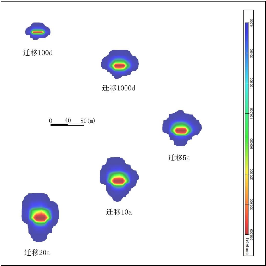
图 6.3-20 非正常情况下 COD 迁移迁移平面图
