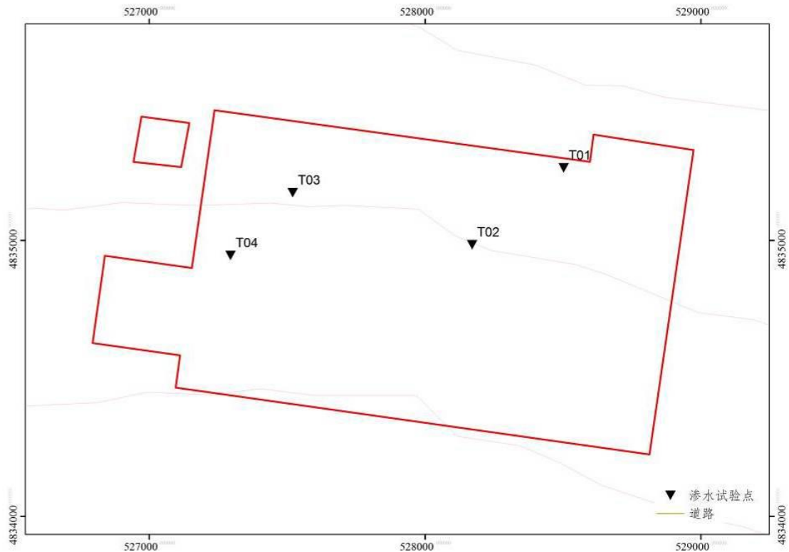
图 6.3-10 厂址区渗水试验点分布图
