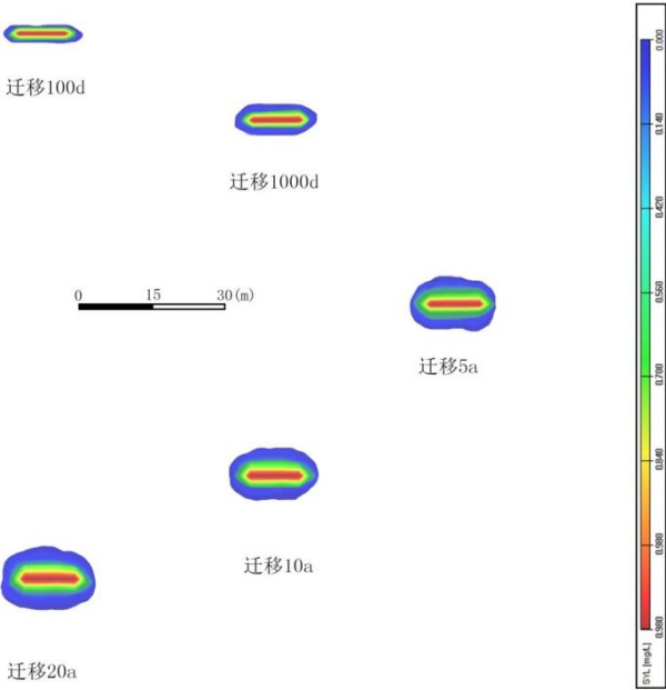
图 6.3-28 非正常情况下苯迁移平面图
