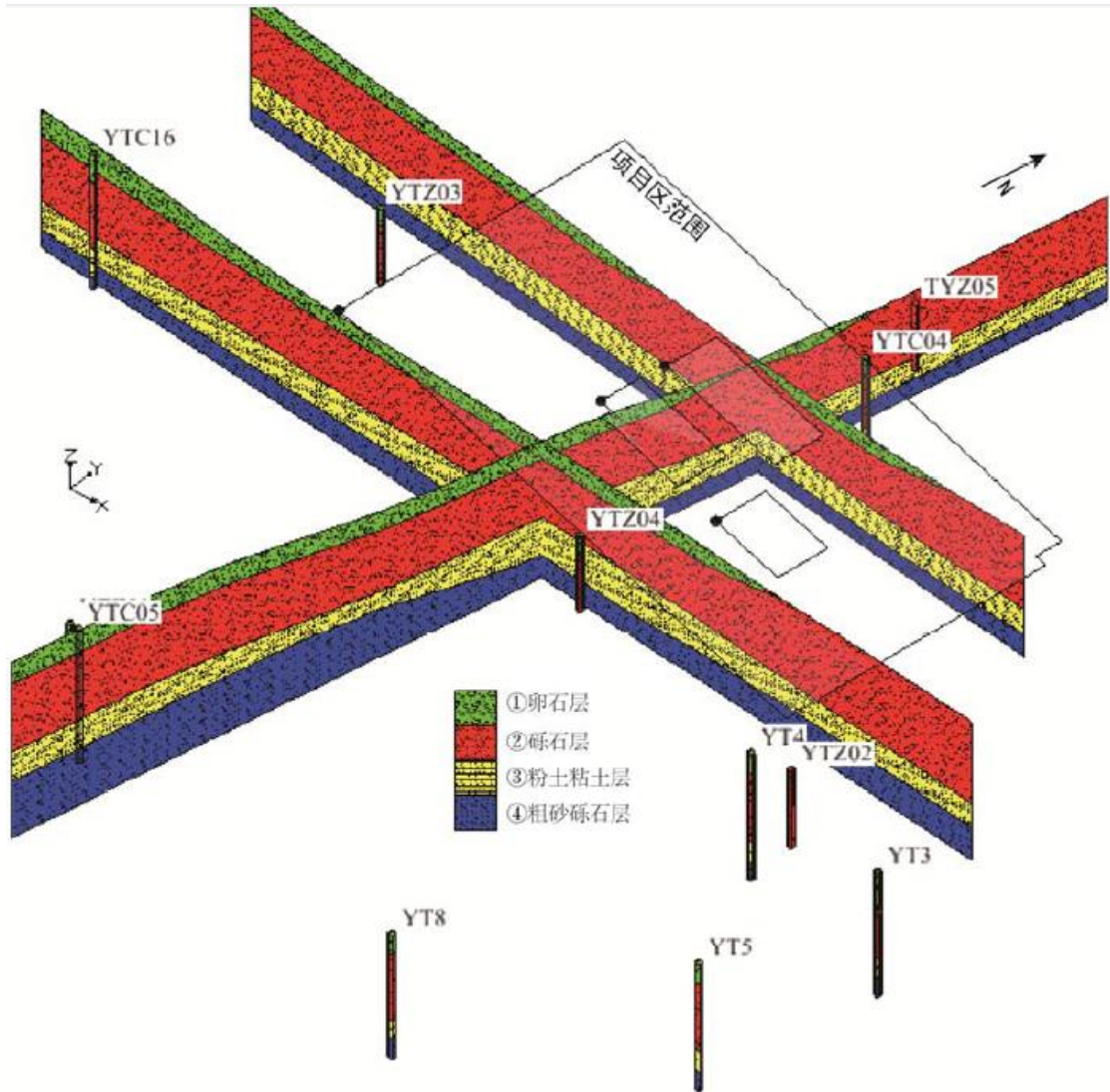
图 6.3-12 项目区地质实体三维视图
