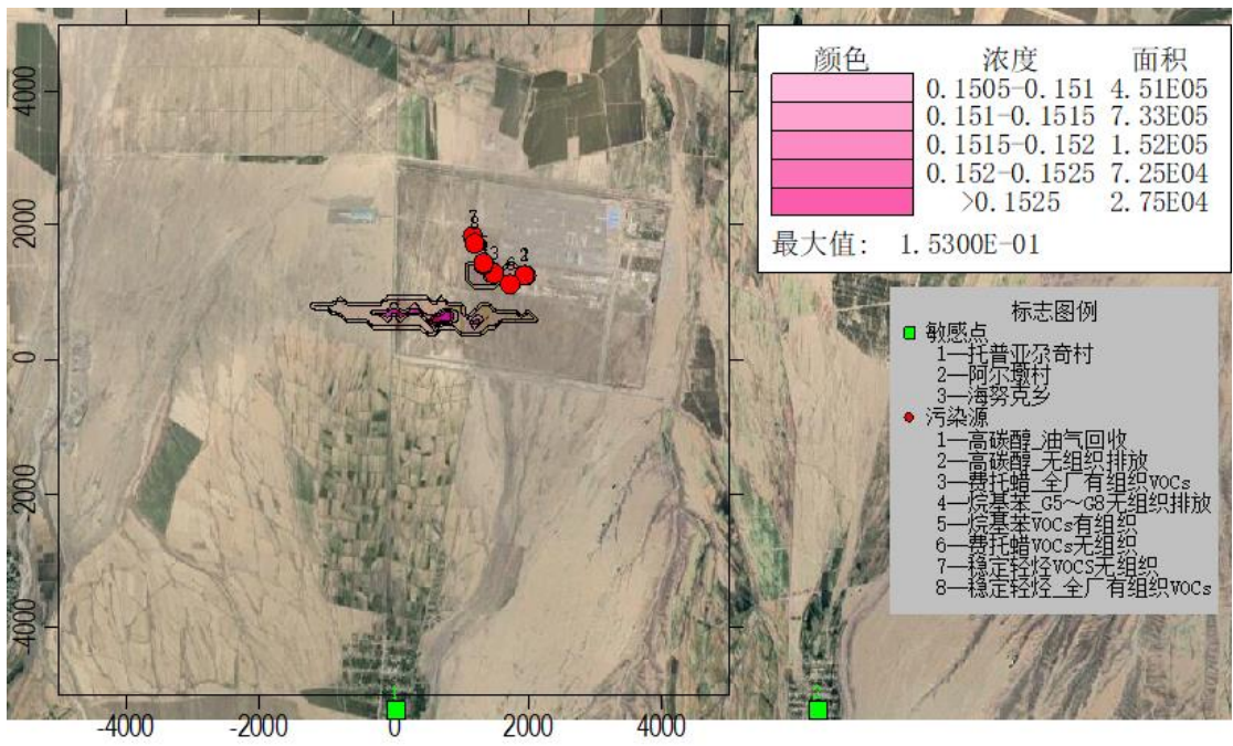
图 6.1-20 NMHC 年均落地浓度分布图 (mg/m³)
