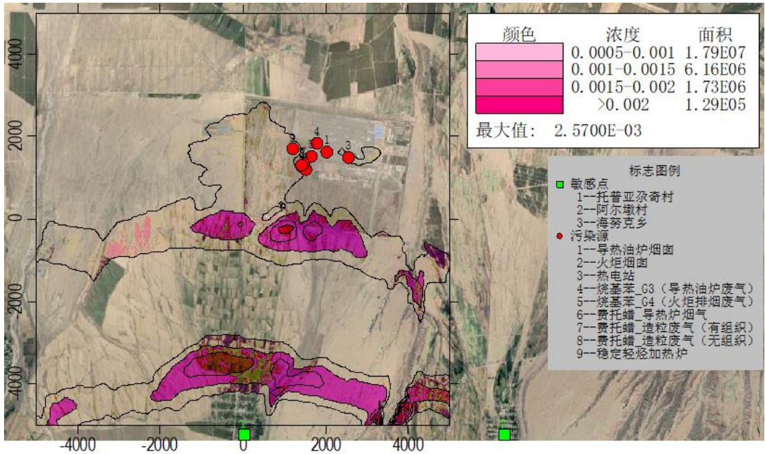
图 6.1-5 SO 2 最大小时落地浓度分布图
