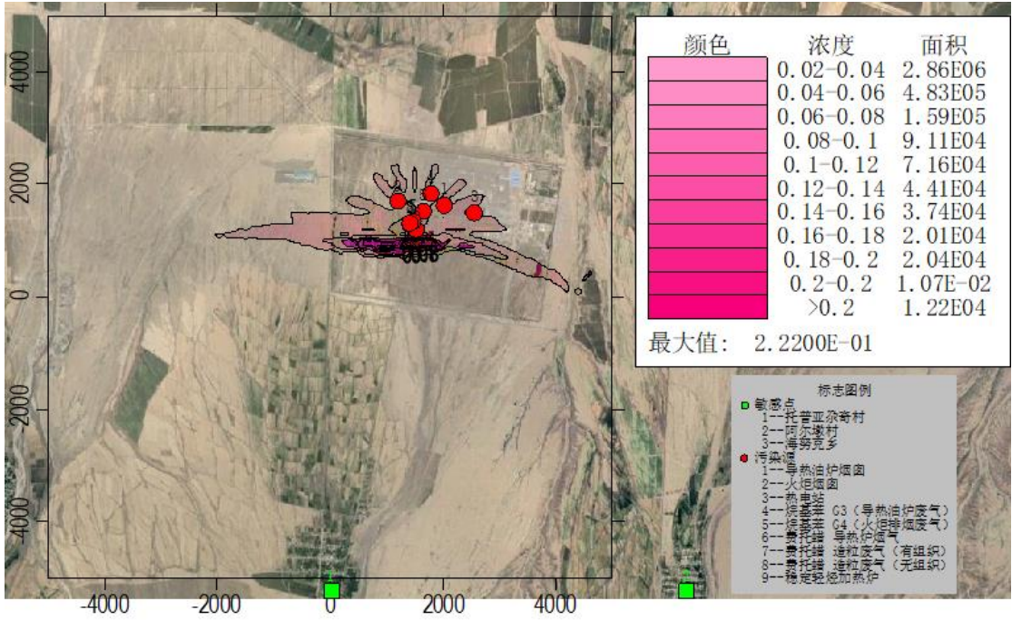
图 6.1-4 PM10 最大小时落地浓度分布图
