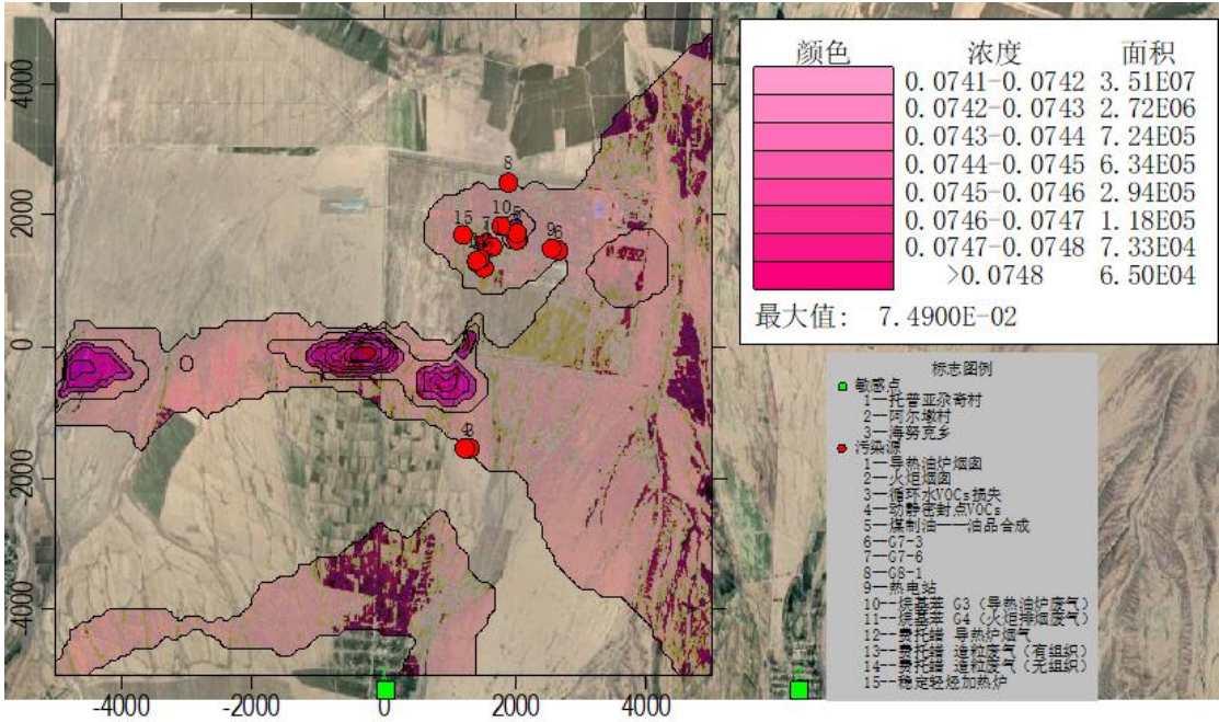
图 6.1-12 NO 2 日保证率叠加分布图
