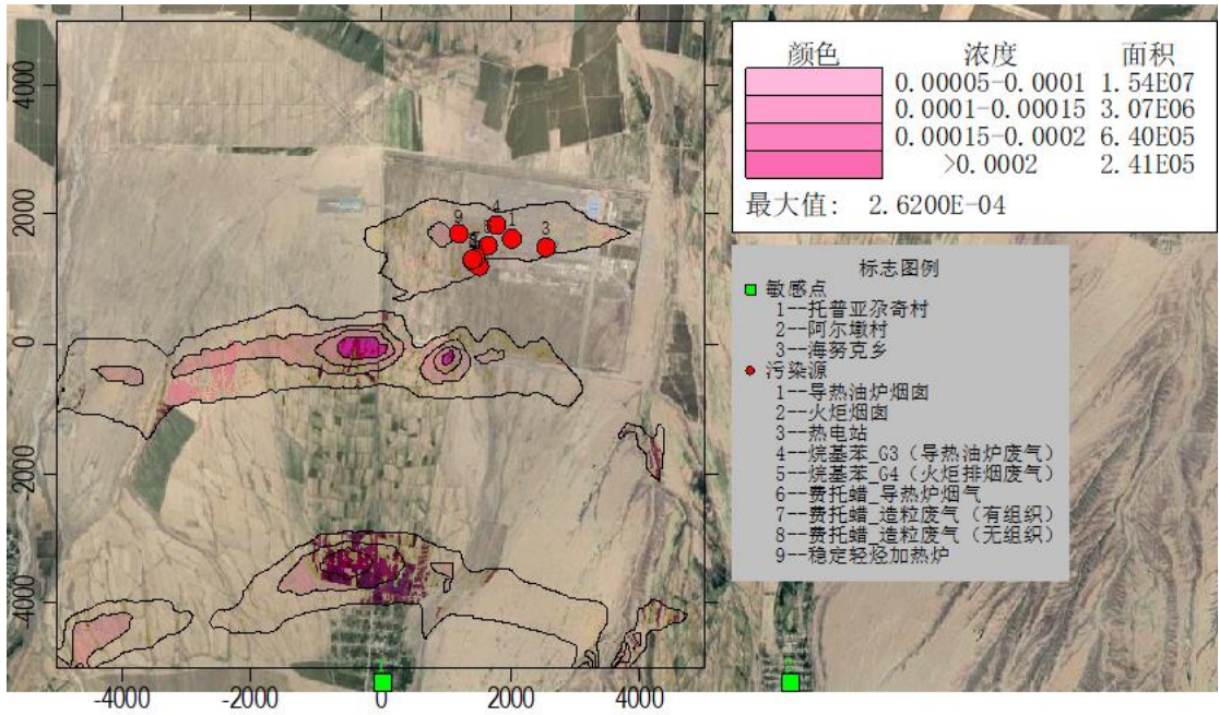
图 6.1-11 SO 2 日保证率叠加分布图
