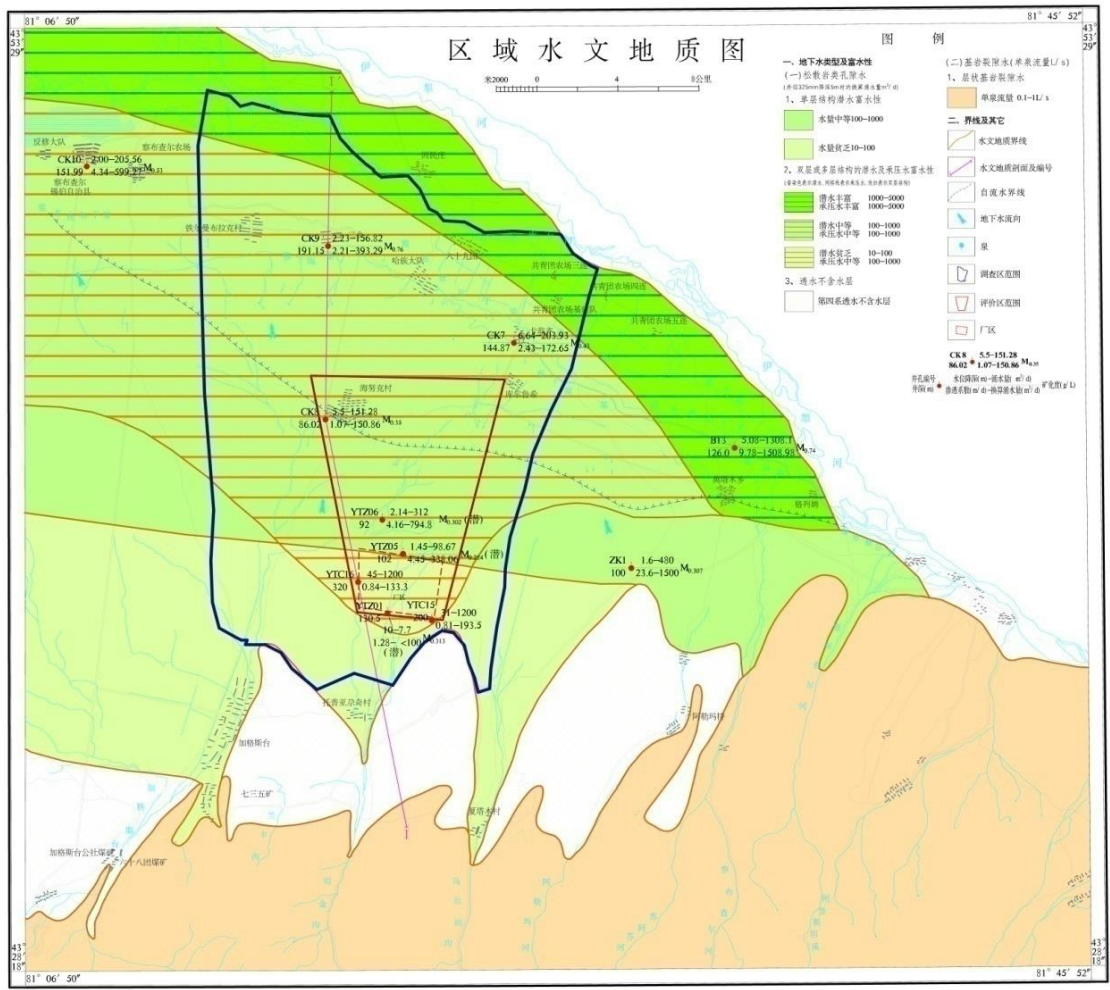
图 6.3-1 区域水文地质图
