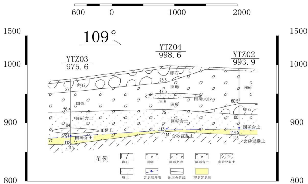
图 6.3-9 厂区 D-D 水文地质剖面图
