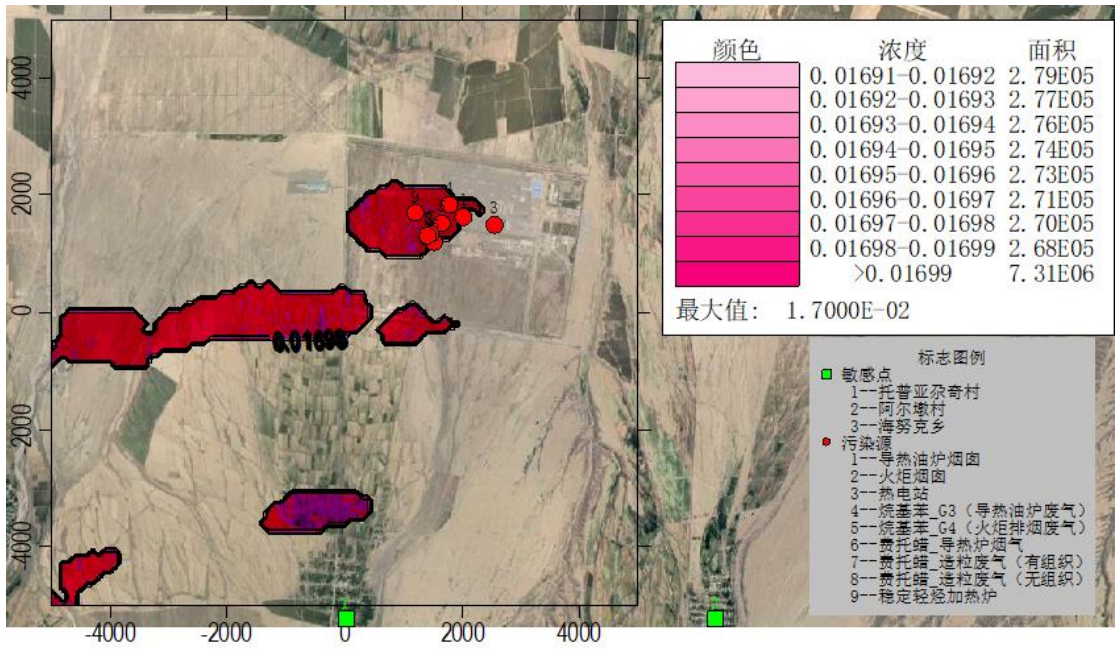
图 6.1-17 SO 2 年均落地浓度分布图 (mg/m 3 )
