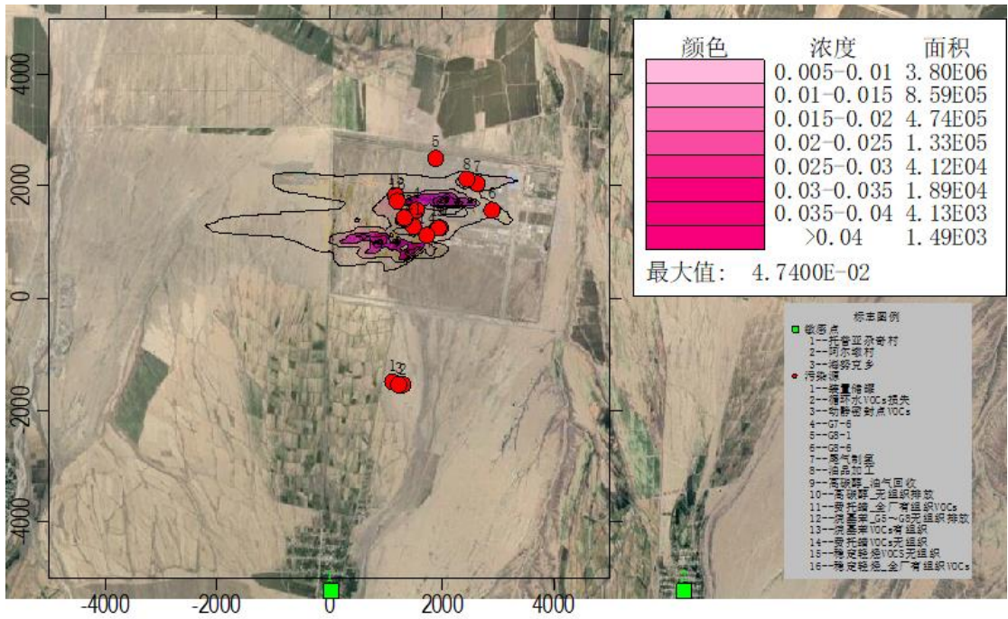
图 6.1-21 VOCs 年均落地浓度分布图 (mg/m³)
