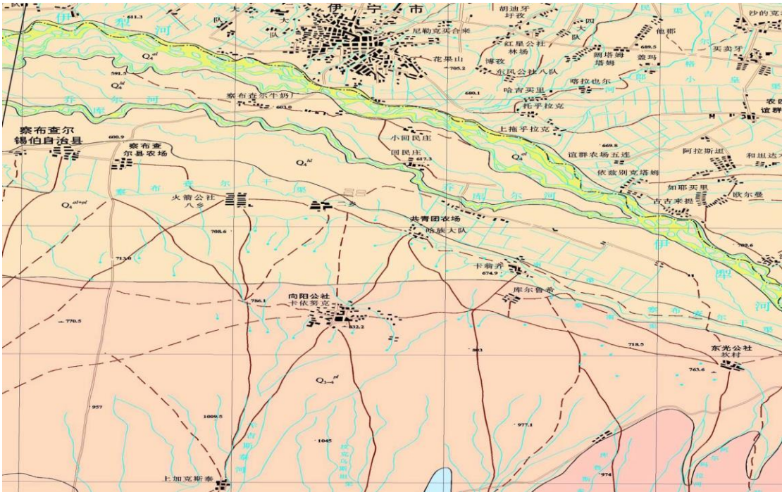
图 5.1-1 厂址工程地质构造图
