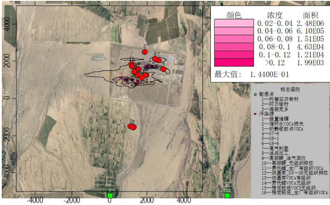
图 6.1-13 VOCs 日保证率叠加分布图
