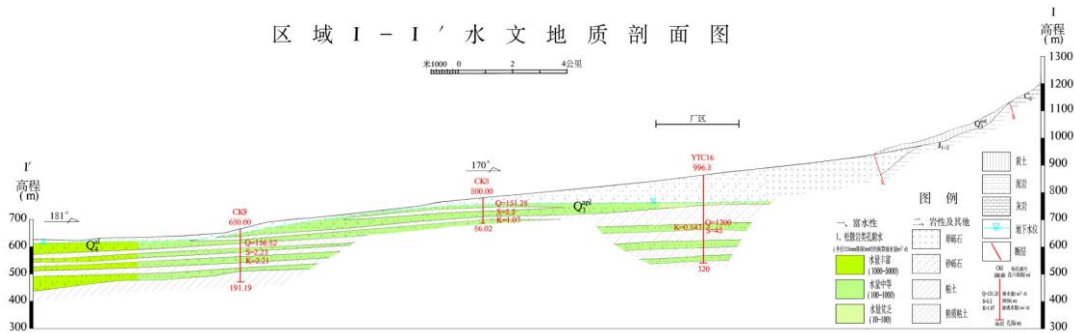
图 6.3-2 区域水文地质剖面图
