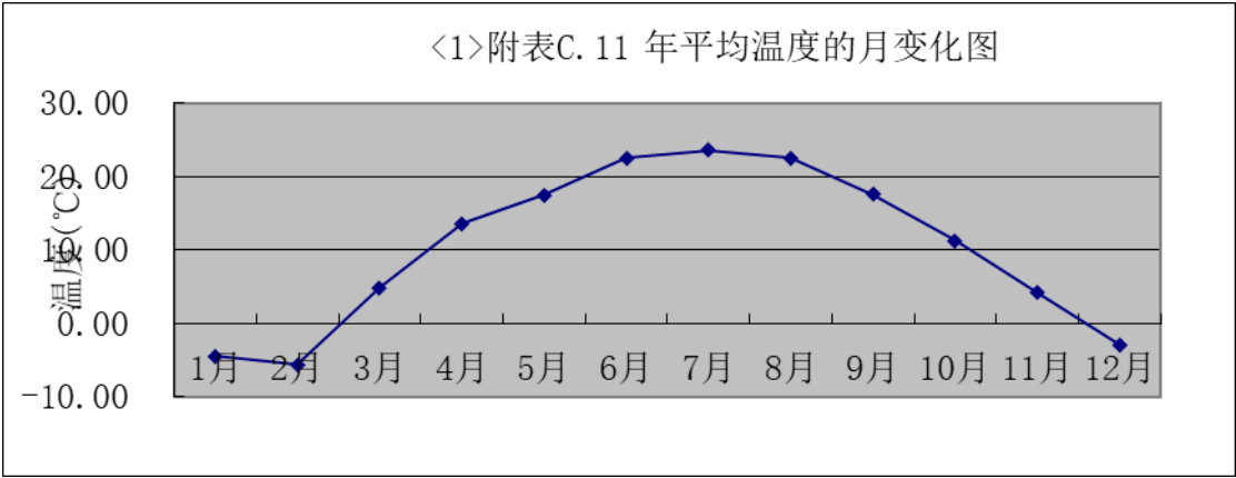
图 6.1-1 伊宁市 2018 年月平均温度变化图
