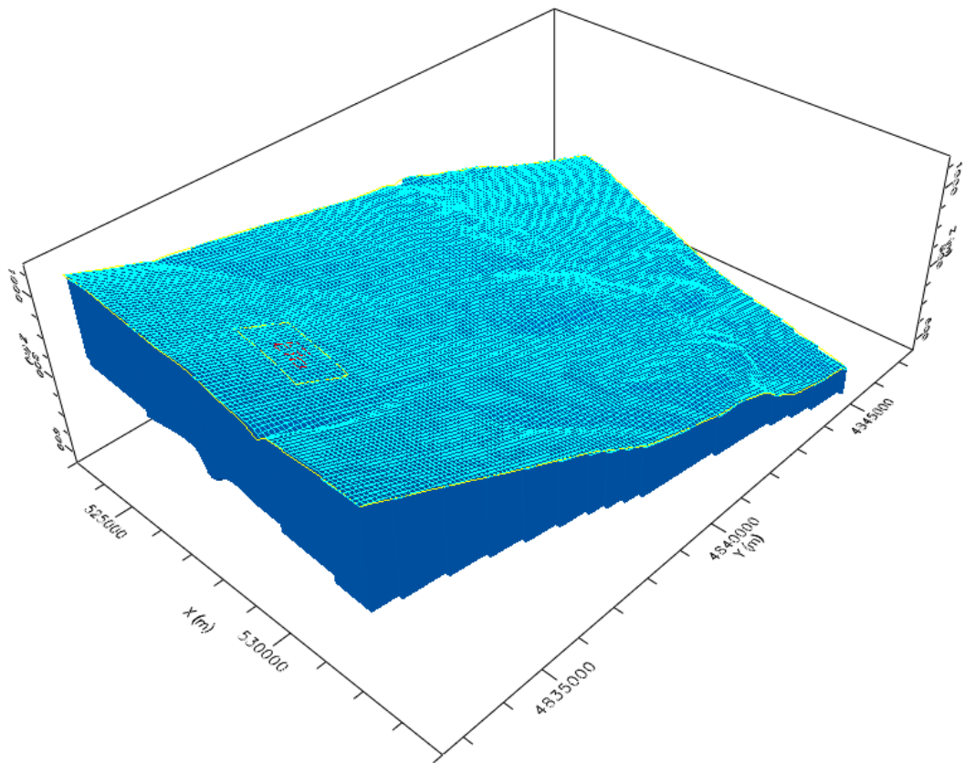
图 6.3-13 模型网格剖分示意图
