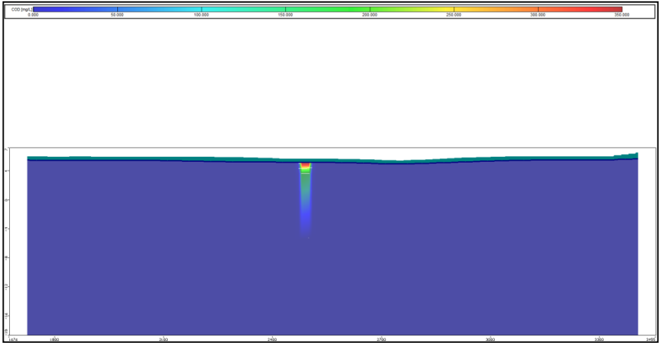
图 6.3-19 正常情况下 a-a'剖面图（COD 迁移 20a 扩散图）
