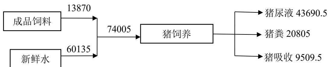
图 3.1-2 物料平衡示意图 单位：t/a
