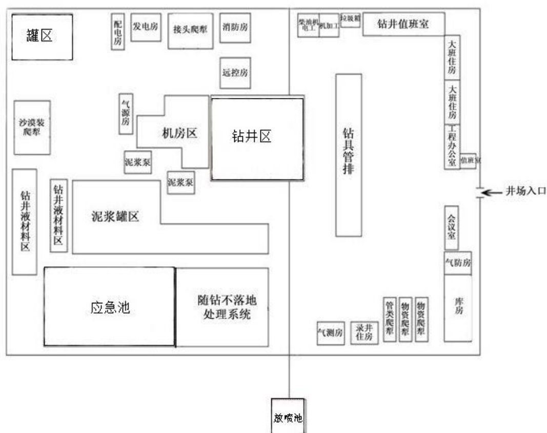
图 4-4 钻井井场平面布置图
