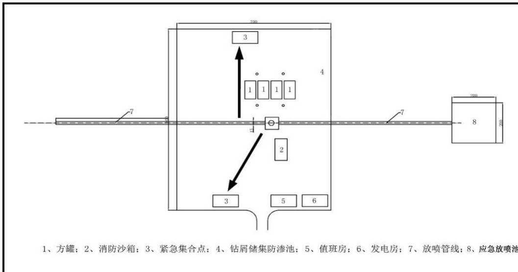
图 4-5 试油期井场平面布置图
