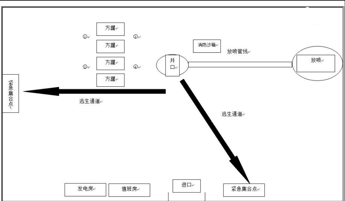
图 4-5 试油期井场平面布置图
