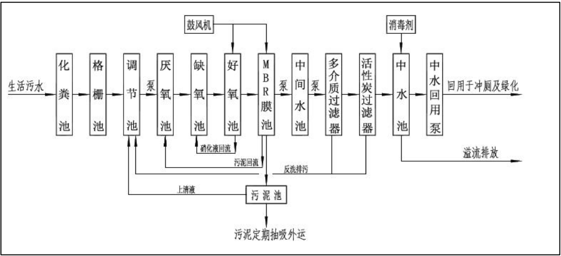
图7.3-2 污水处理工艺流程图
