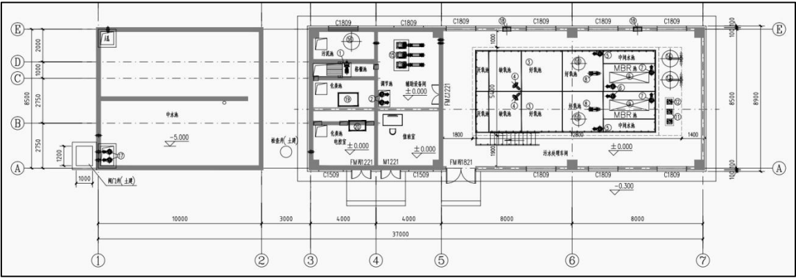
图7.3-1 污水处理设备平面布置图
