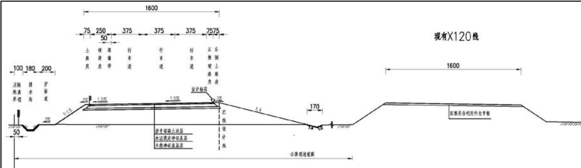
图 3.1-3 公路路基标准横断面图（分离路基）
