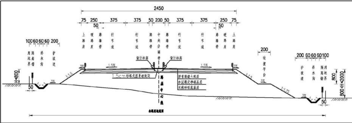
图 3.1-2 公路路基标准横断面图（整体路基）
