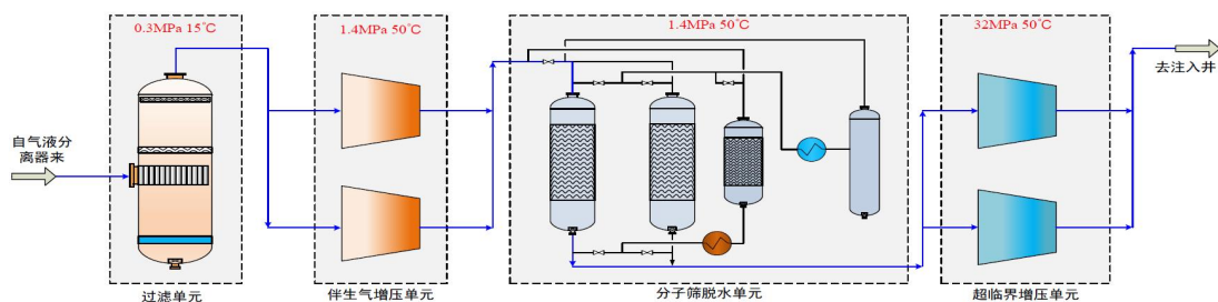
图 3.6-7 伴生气循环注入整体工艺
