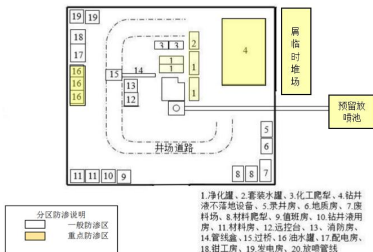
图 3.5-5 单井钻井井场布局示意图
