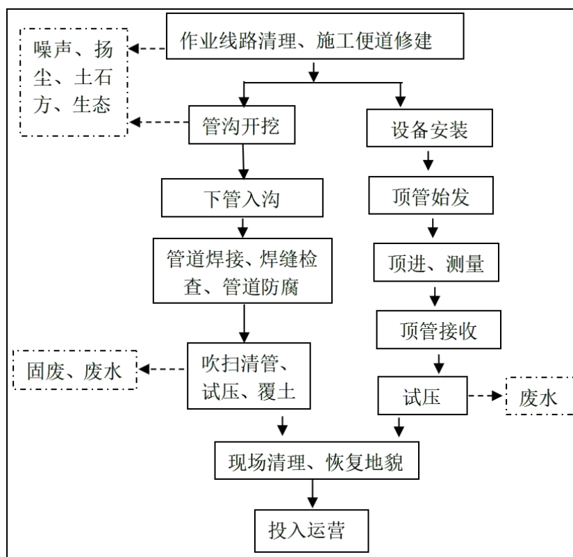
图 3.7-4 集输管线建设工艺流程及产污环节示意图
