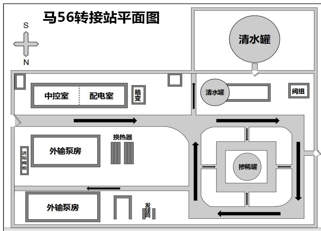
图 3.1-2 马 56 接转站平面布置图
