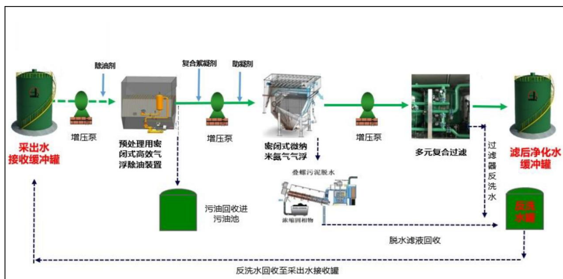
图 3.6-5 牛圈湖联合站新建撬装采出水处理系统工艺流程示意图
