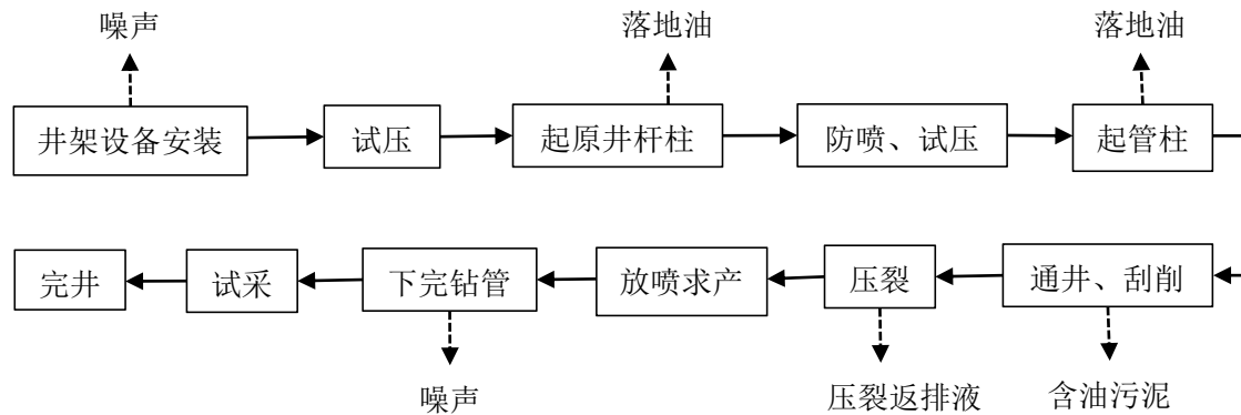
图 3.7-6 压裂作业施工流程及产污环节示意图
