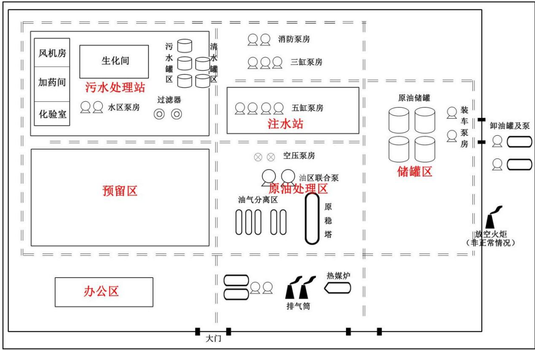
图 3.6-3 牛圈湖联合站平面布置图
