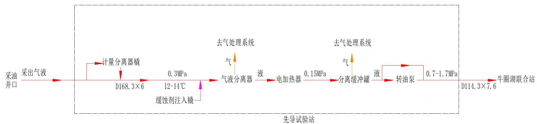
图 3.6-6 先导试验站总体工艺流程图
