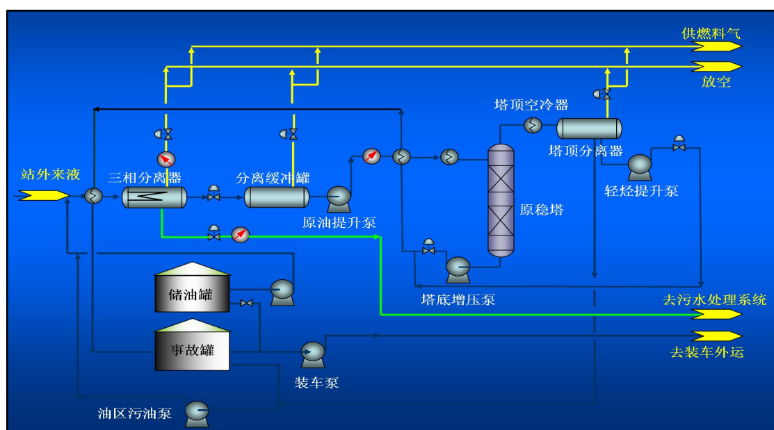
图 3.6-4 牛圈湖联合站原油处理工艺流程示意图
