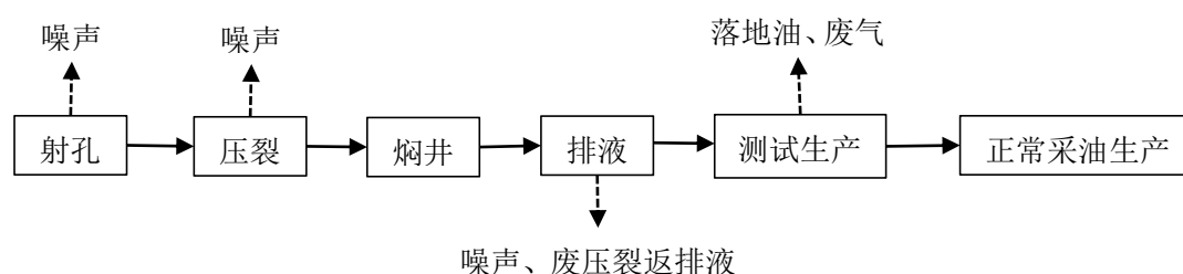
图 3.7-3 压裂作业工艺流程及产污环节图
