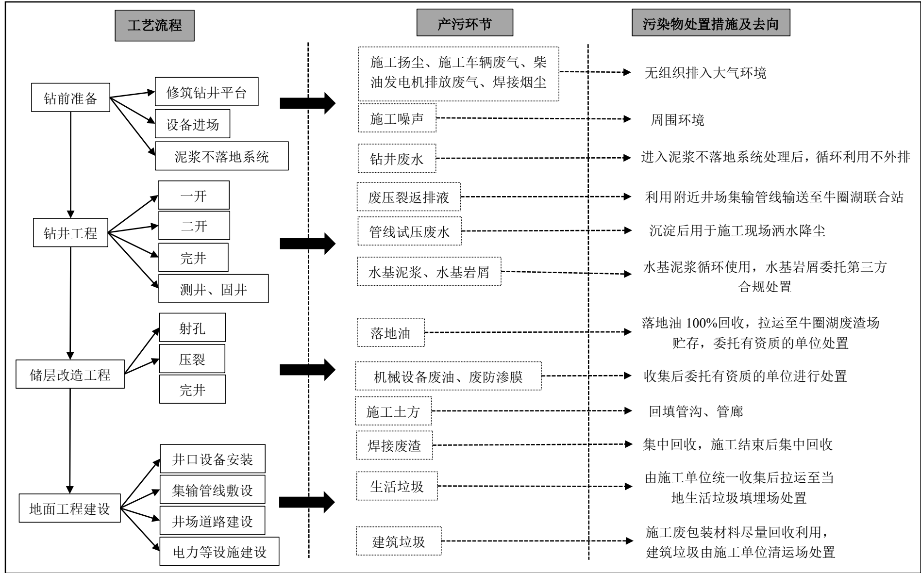
图 3.7-7 施工期主要工艺流程及产污环节示意图
