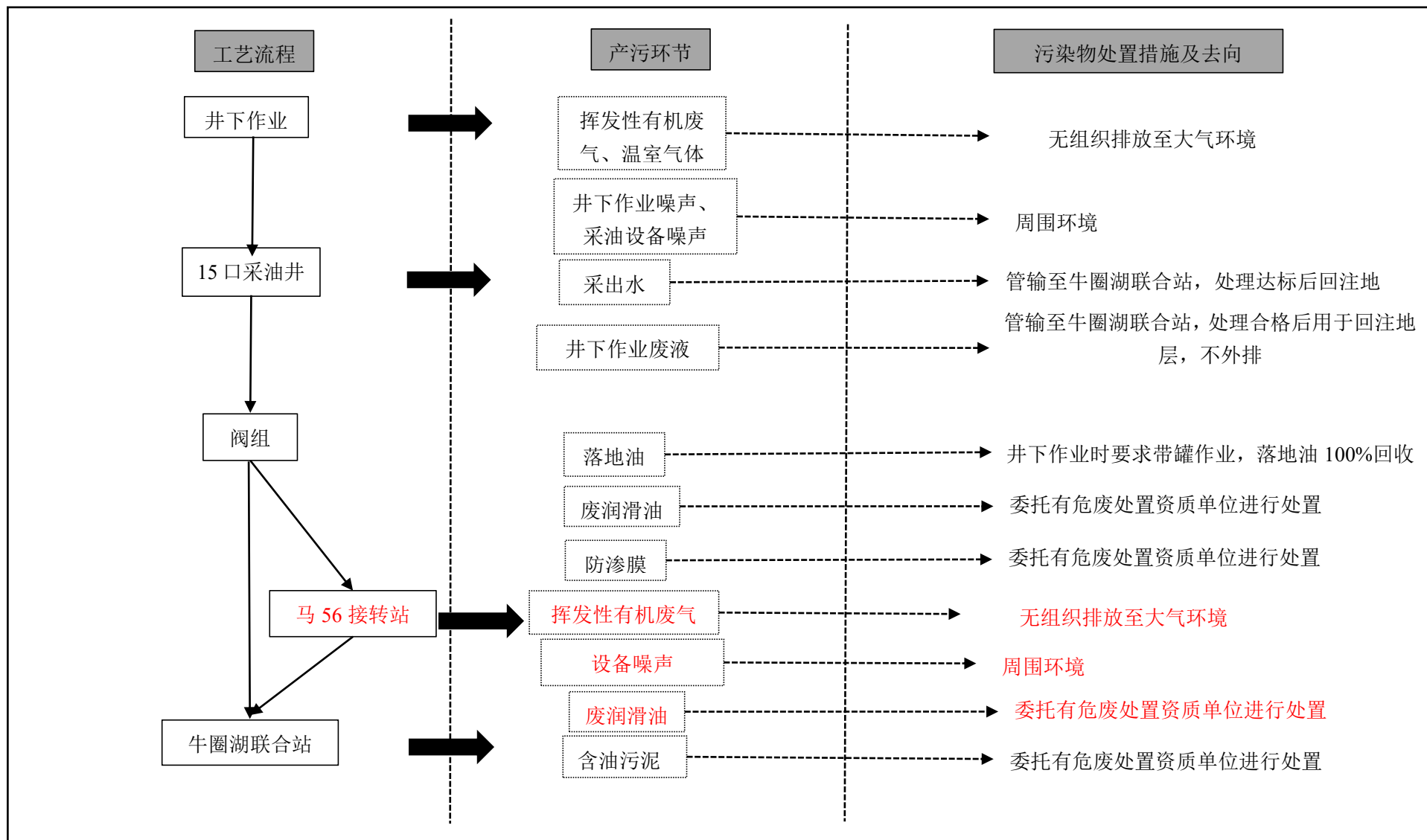
图 3.7-7 运营期主要工艺流程及产污环节示意图
