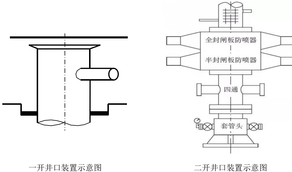
图 3.5-4 水平井井口装置
