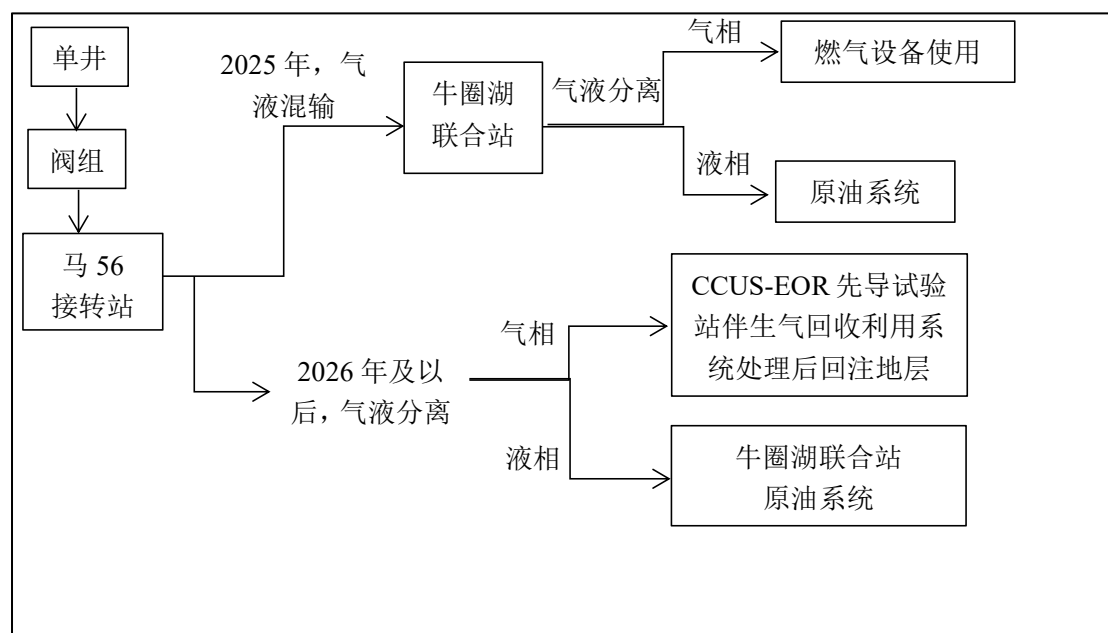
图 3.5-1 总体工艺流向图
