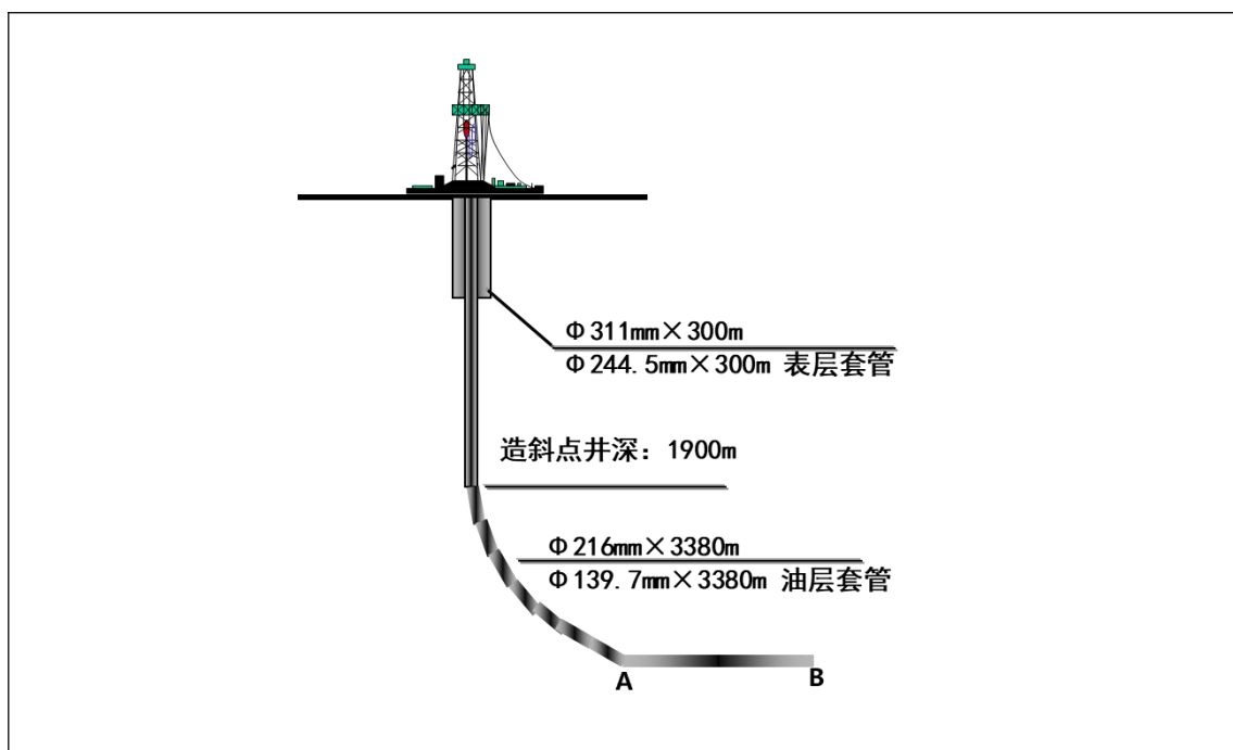
图 3.5-3 井身结构示意图
