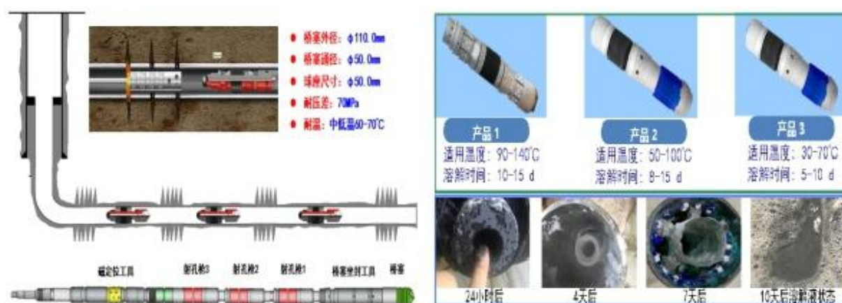
图 3.5-6 水平井桥塞分段压裂工艺图
