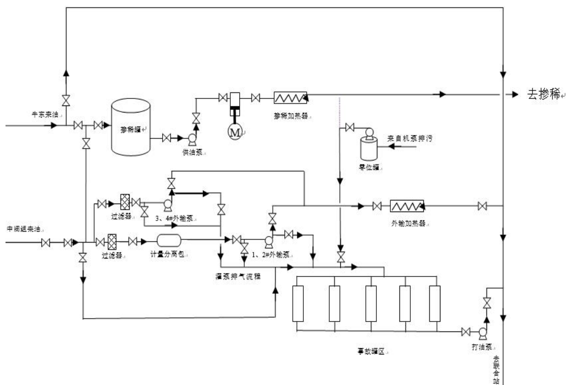
图 3.1-1 马 56 接转站站内工艺流程现状图
