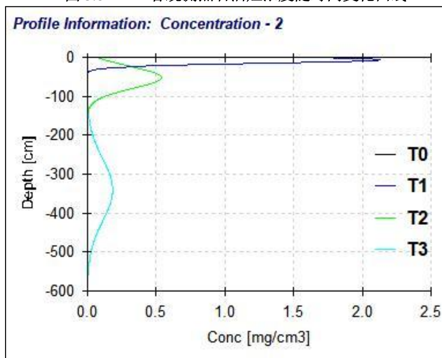
图 5.8-5 石油烃在不同时间沿土壤迁移情况
