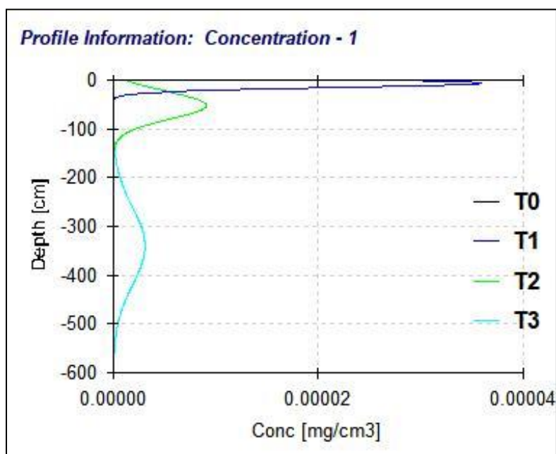
图 5.8-3 石油烃在不同时间沿土壤迁移情况
