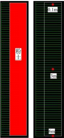
图 5.8-1 土壤岩性概化及观测点分布图
