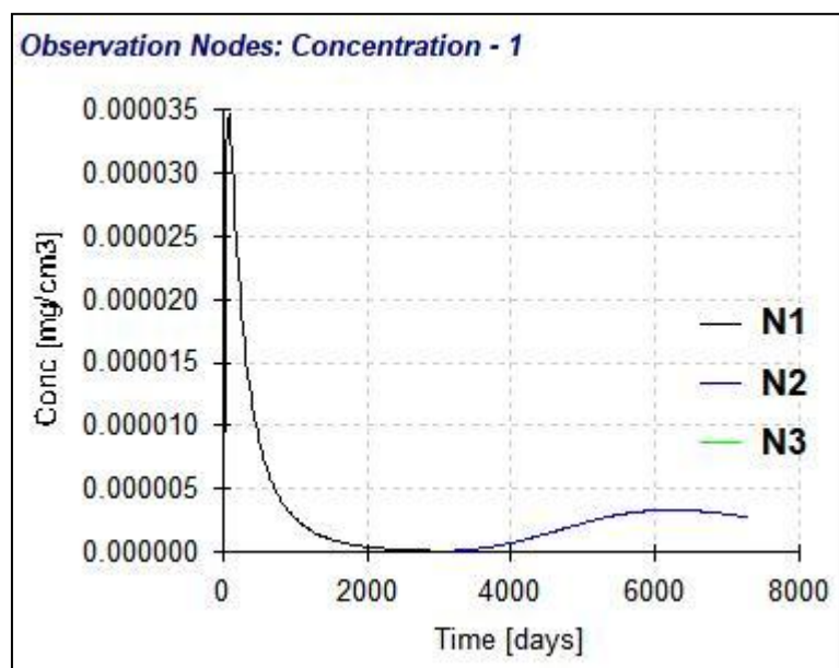
图 5.8-2 各观测点石油烃浓度随时间变化曲线
