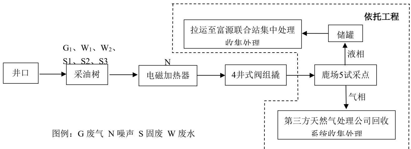
图 3.4-9 运营期集输工艺流程及排污节点图
