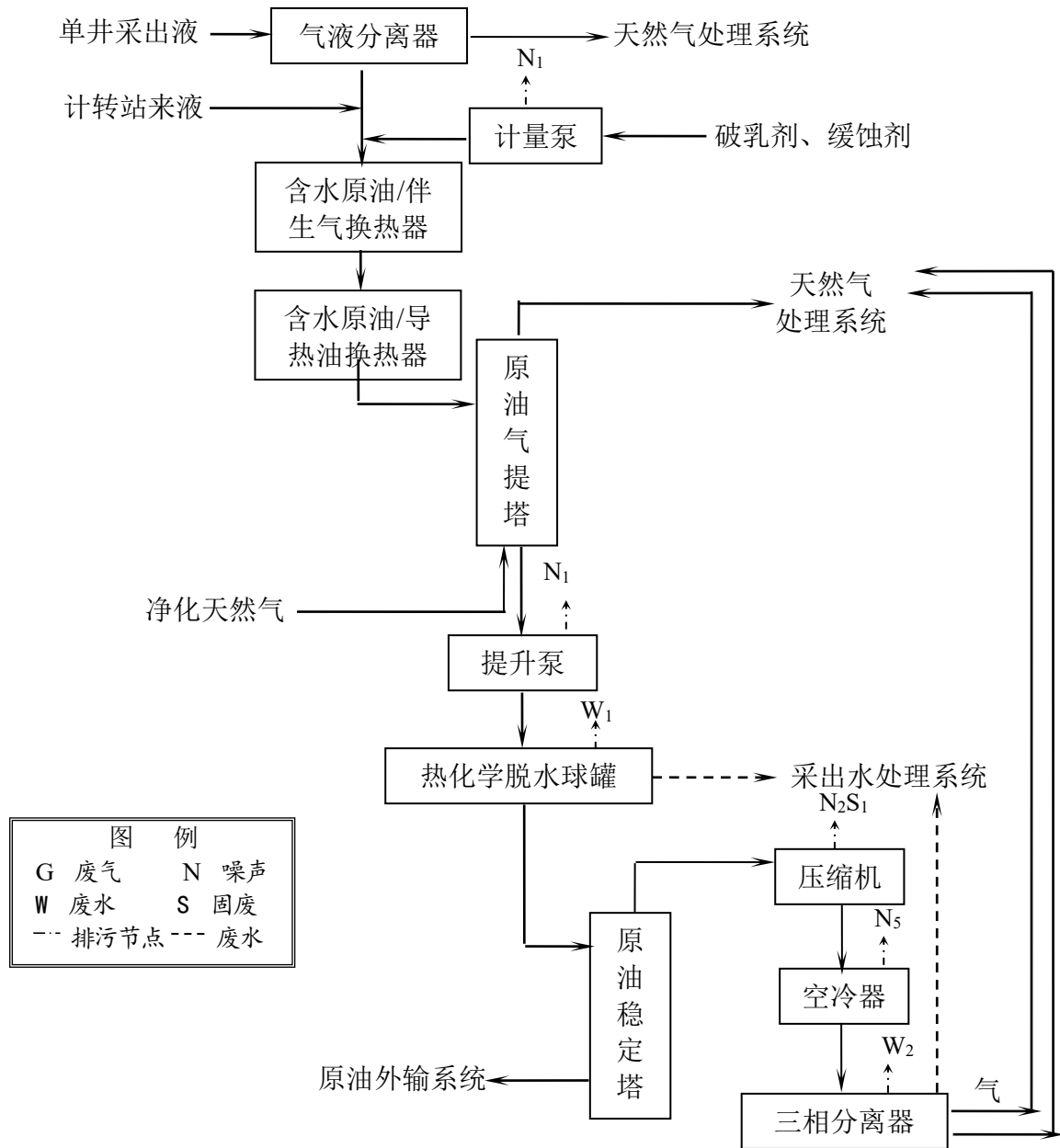
图 3.2-1 原油处理系统工艺流程图
