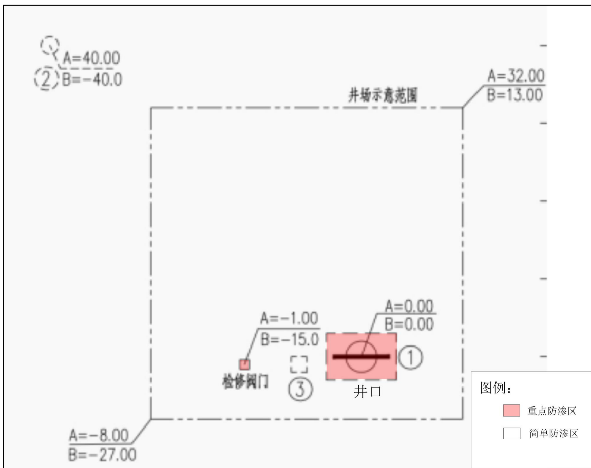
图5.4-5 运营期防渗分区图
