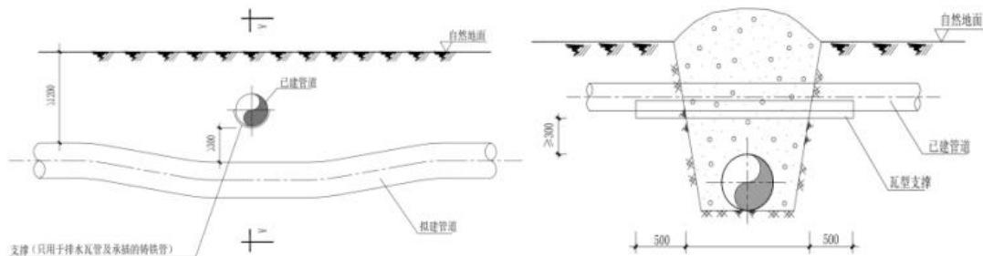
图3.4-7 管线与已建管线穿越示意图
