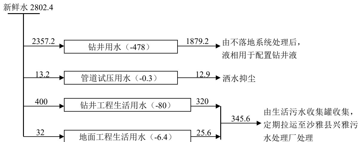
图 3.4-3 项目施工期给排水平衡图 (单位：m 3 )
