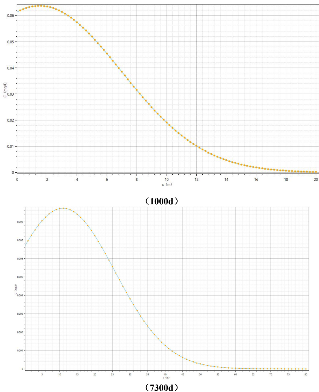
图 5.4-2 施工期石油类运移结果图
