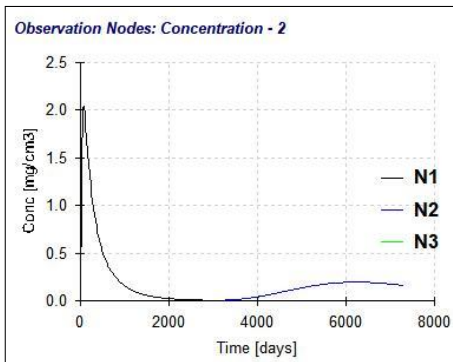
图 5.8-4 各观测点石油烃浓度随时间变化曲线
