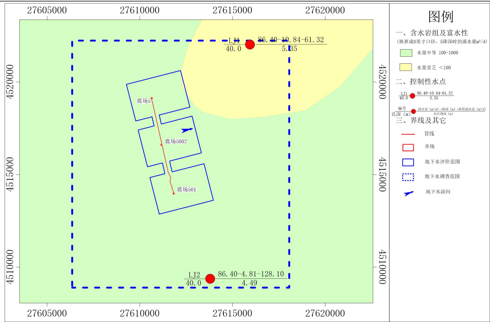
图 5.4-1 评价区水文地质图
