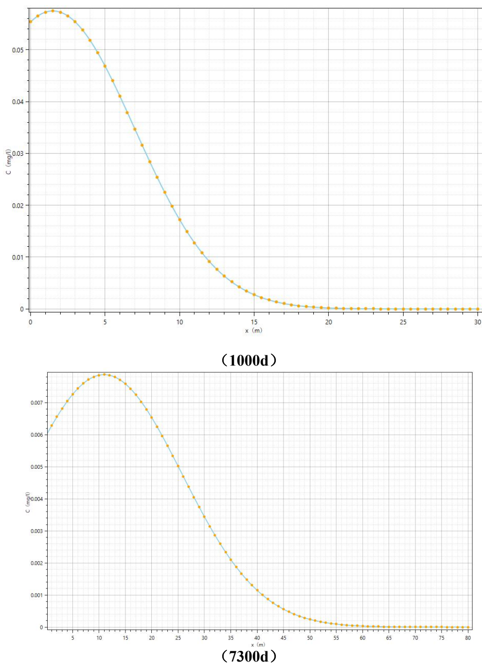
图 5.4-3 运营期石油类运移结果图
