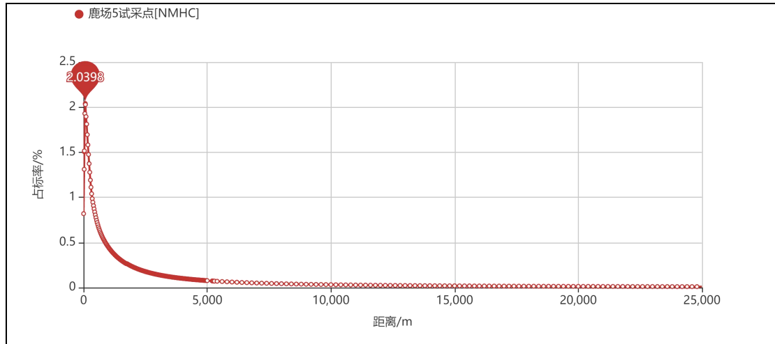
图 5.2-2 面源最大 P_{\max} 和 D_{10\%} 预测结果图
