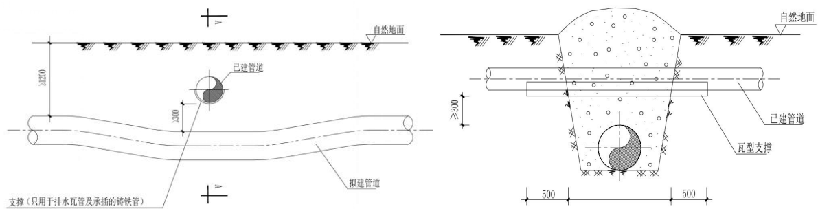
图 3.4-5 管道交叉施工作业示意图
