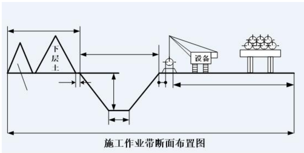
图 3.4-4 一般地段管道施工方式断面示意图
