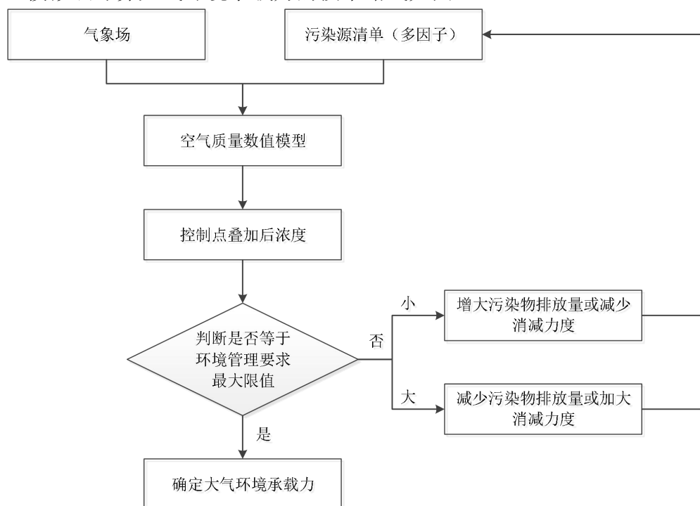
图 5.11-1 大气环境承载力计算技术路线图
