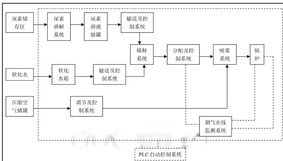
图 3.3-3 SNCR 脱硝工艺流程图
