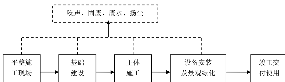
图 3.3-1 施工期工艺流程及产污节点图
