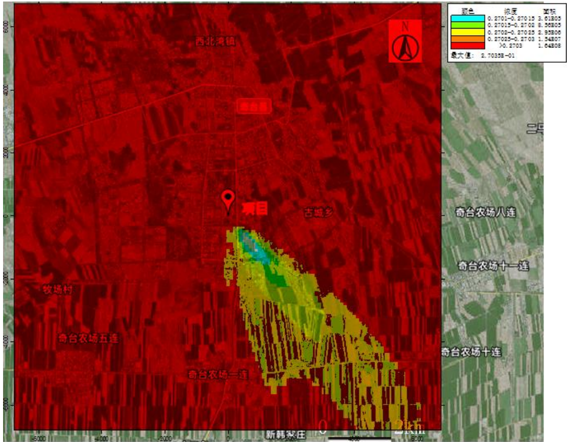
图 5.2-10 网格点本项目叠加拟建项目 PM 10 保证率日均浓度值等值线分布图
