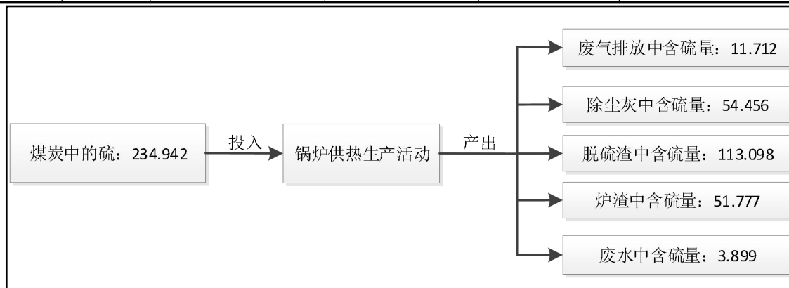
图 3.3-4 项目硫平衡图 (t/a)
