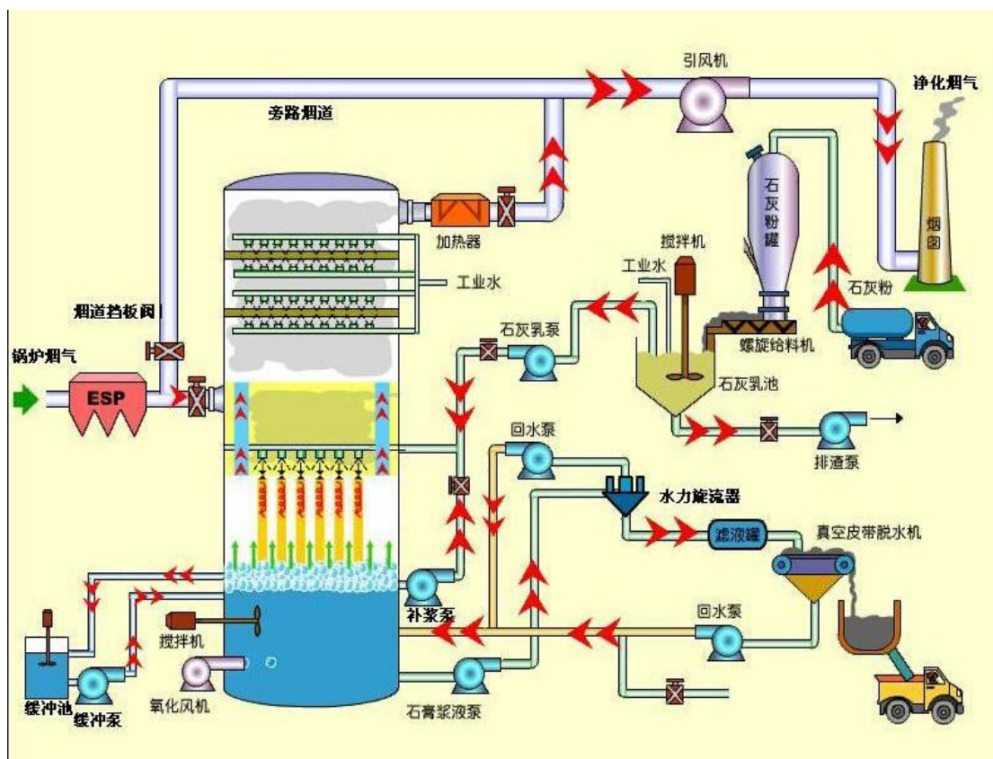
图 6.2-3 石灰石-石膏湿法脱硫工艺流程图
