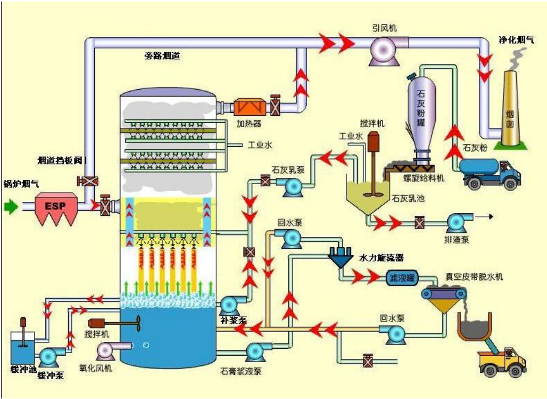
图 3.3-1 石灰石-石膏湿法烟气脱硫工艺流程图
