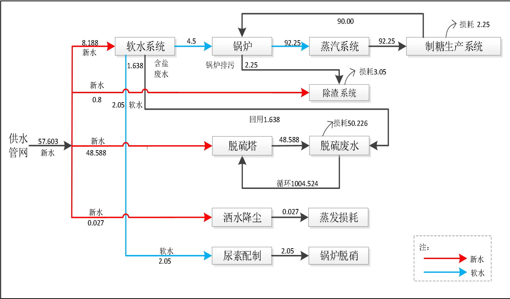
图 3.2-5 项目水平衡图 (m³/h)
