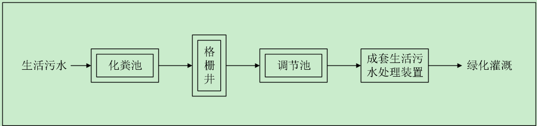
图 6.3-1 生活污水处理工艺流程
