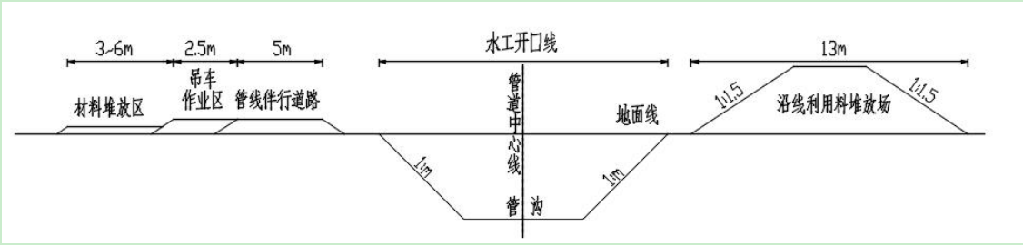
图3.3-3 管道作业带位置关系示意图
