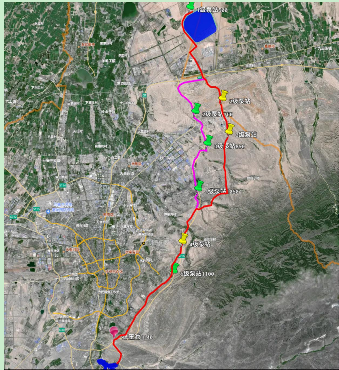
图 3.3-2 工程输水线路比选平面布置图
