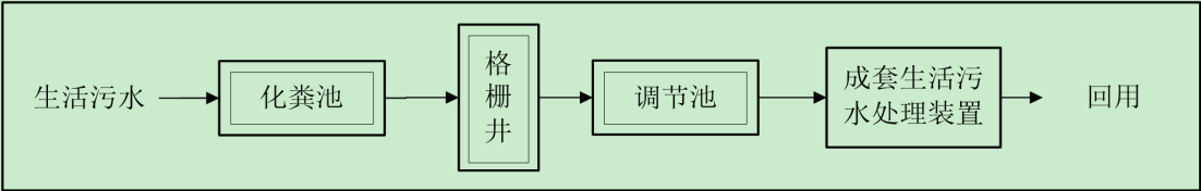
图 6.4-1 管理站生活污水处理工艺流程
