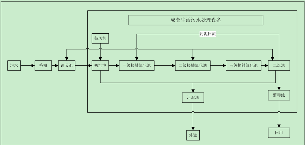
图6.3-2 一体化污水处理装置工艺流程图
