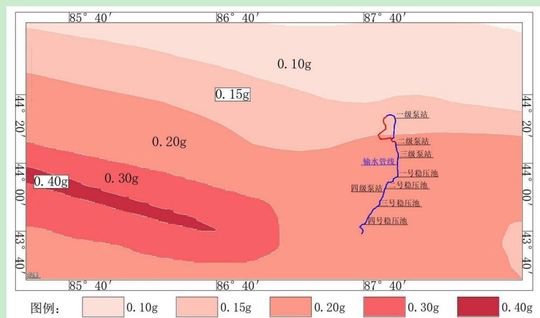
图 2.1-1 地震动峰值加速度区域划分图
