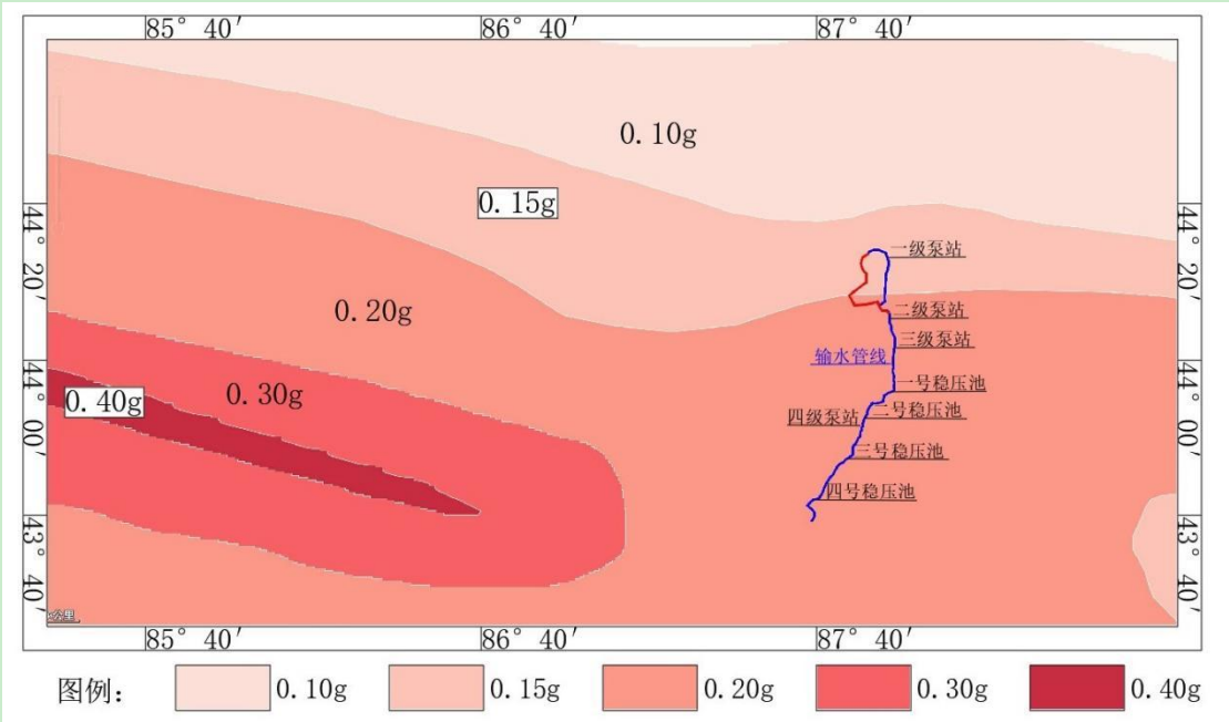
图 4.1-2 地震动峰值加速度区域划分图
