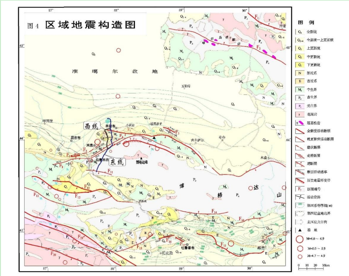
图 4.1-1 区域地震与地质构造纲要图
