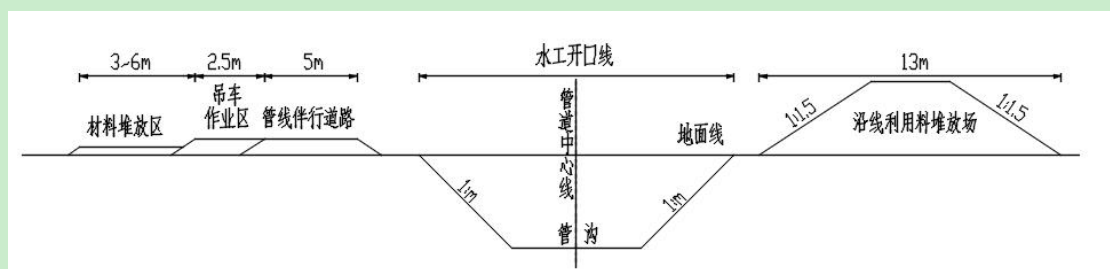
图 2.2-1 管道-临时伴行道路-利用料堆位置关系示意图
