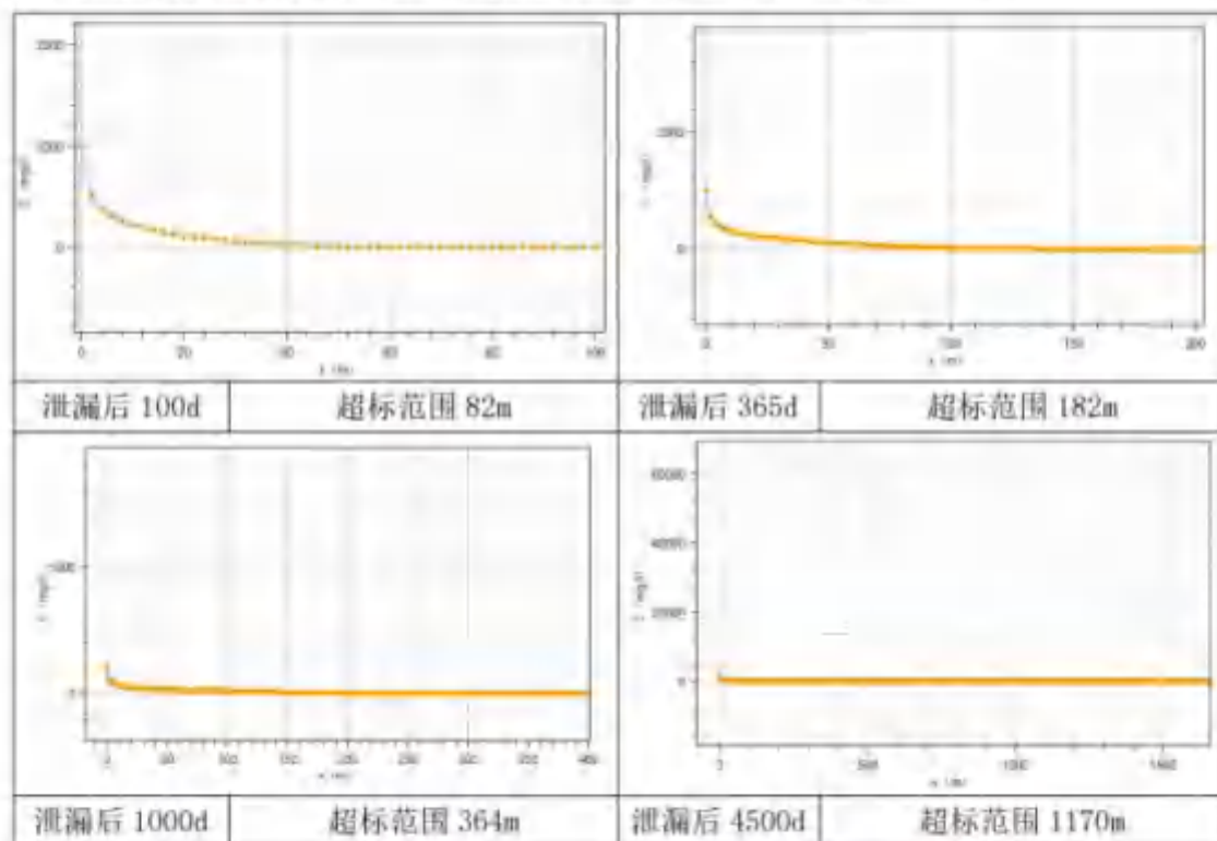
图 6-5 输油管线长期泄漏事故石油类运移范围示意图
