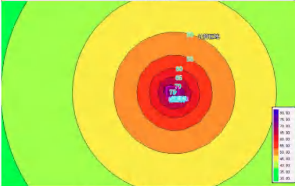
图 6-8 开挖施工场界噪声预测等声级线图
