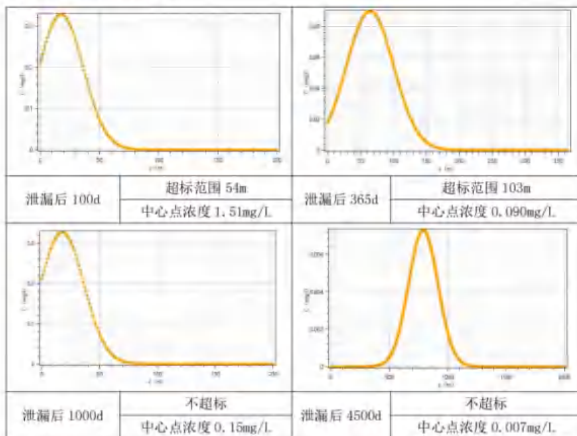
图 6-4 输油管线瞬时泄漏事故石油类运移范围示意图
