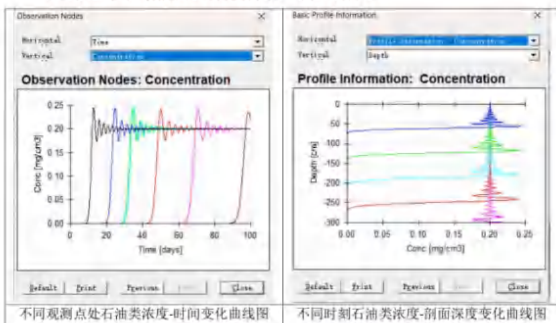
图 6-7 MB5014 单井集油管线泄漏土壤预测结果图
