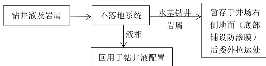
图 6.1-1 水基钻井岩屑处理工艺流程图
