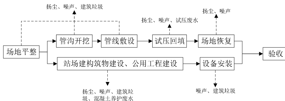
图 3.2-6 施工工艺及产污节点示意图
