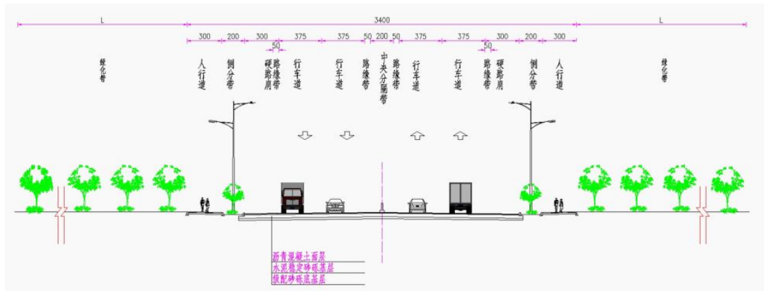
图 3.2-4 K75+809.025-K80+125.737 段路基标准横断面图
