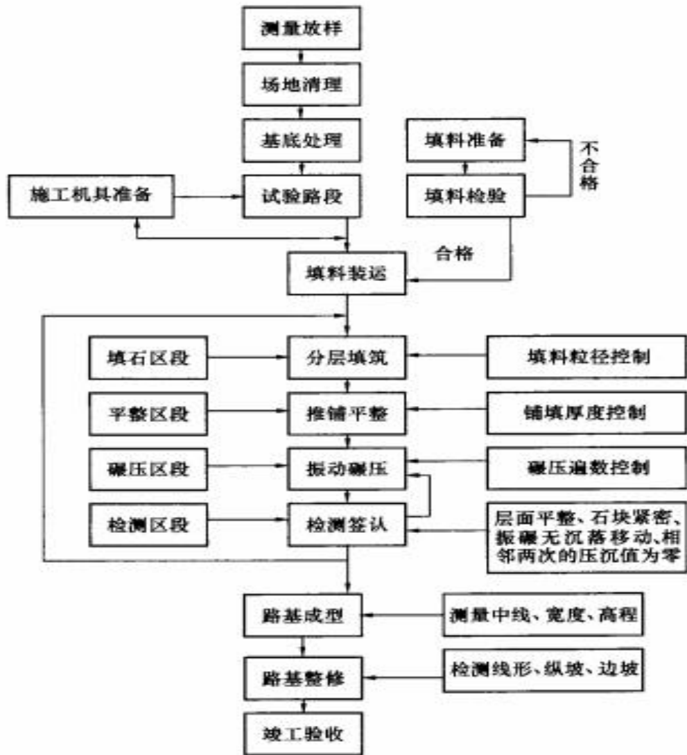
图 3.2-7 填方路基施工程序图
