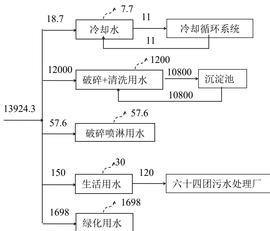
图3.3-1 本项目水平衡图（m 3 /a）
