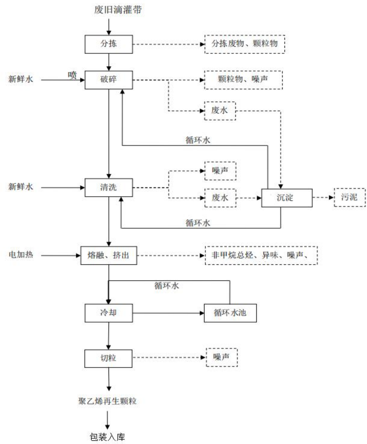
图3.4-2 再生造粒工艺流程及产污节点图
