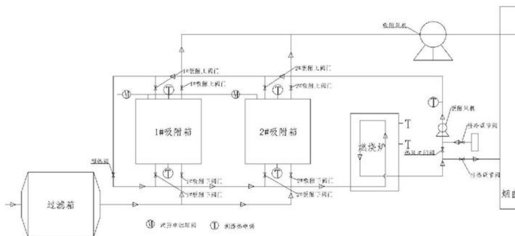
图7.2-1 有机废气处理工艺示意图
