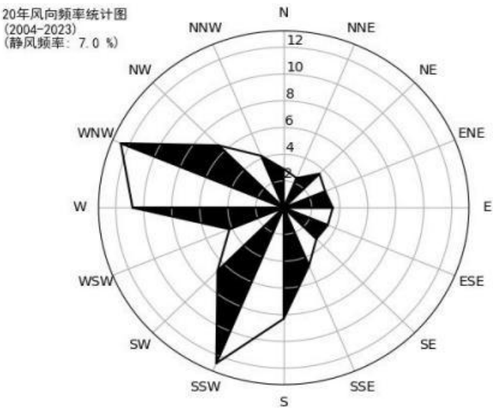
图 6.2-1 吉木萨尔县近 20 年风向玫瑰图（静风频率为 7.0%）
