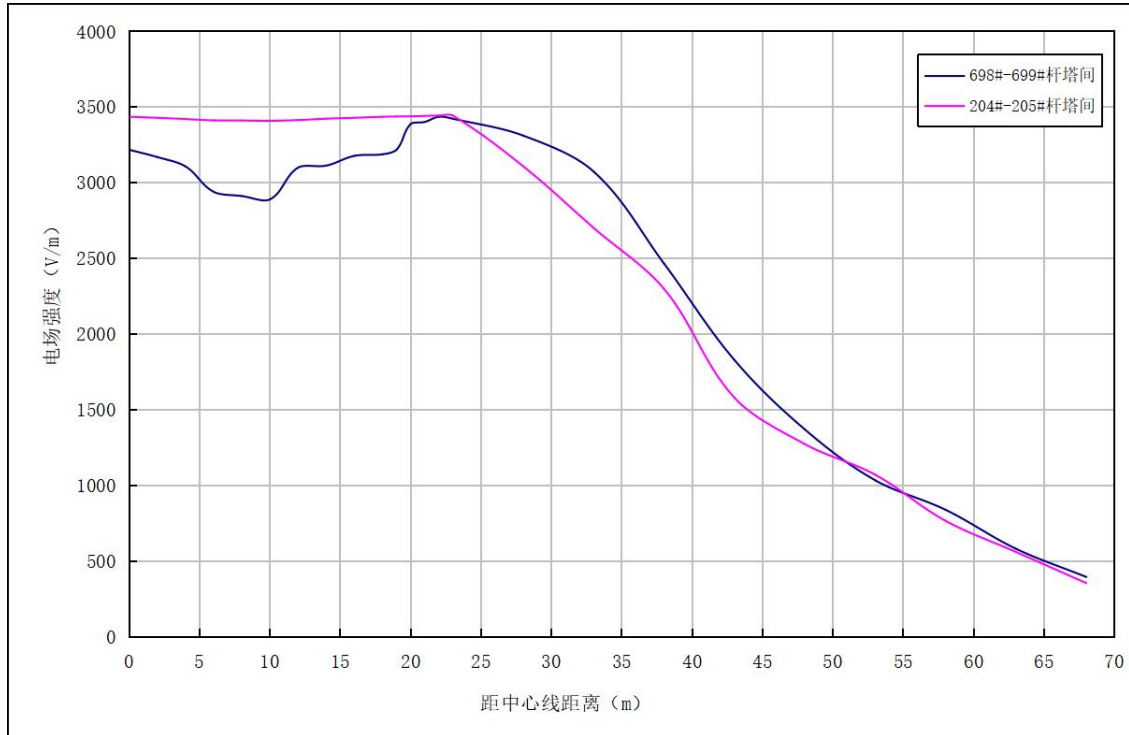
图 6.1-3 750kV 巴吐Ⅱ线 698#-699#杆塔、204#-205#杆塔间工频电场强度衰减断面曲线图
