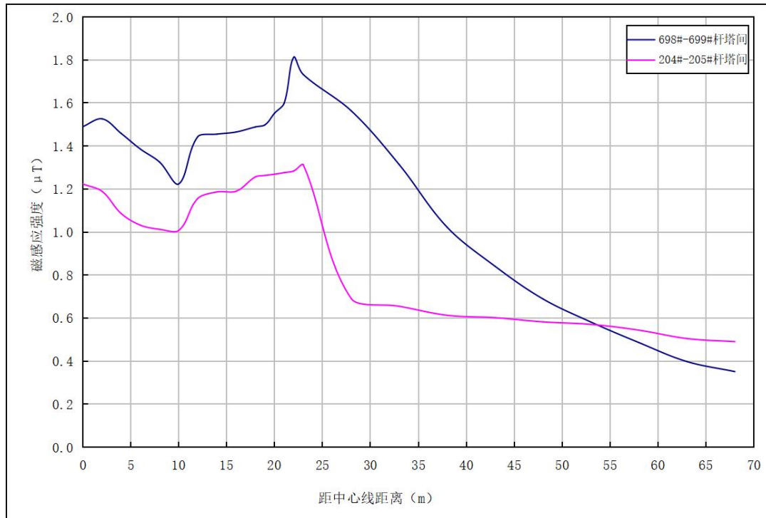
图 6.1-4 750kV 巴吐Ⅱ线 698#-699#杆塔、204#-205#杆塔间频磁感应强度衰减断面曲线图
